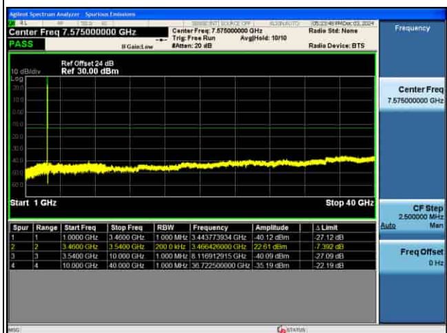
CSE_5G_n77(K)_30KHz_.PI2-BPSK_70M CH634332_1RB@1_
