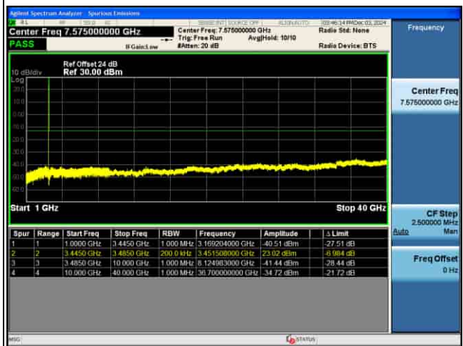
CSE_5G_n77(K)_30KHz_.PI2-BPSK_30M CH633334_1RB@1_
