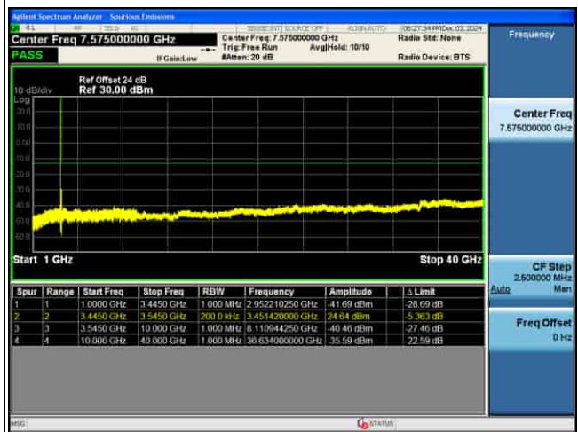
CSE_5G_n77(K)_30KHz_.PI2-BPSK_90M CH633334_1RB@1_
