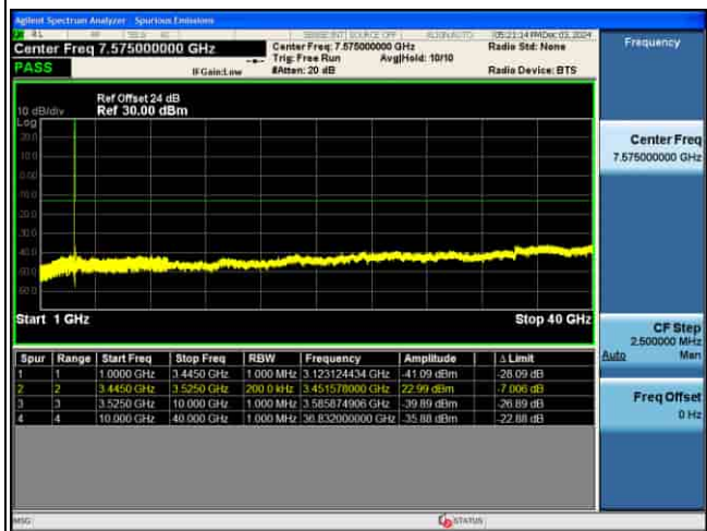
CSE_5G_n77(K)_30KHz_.PI2-BPSK_70M CH633334_1RB@1_
