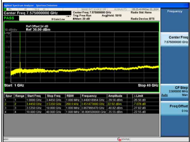
CSE_5G_n77(K)_30KHz_.PI2-BPSK_80M CH633334_1RB@1_
