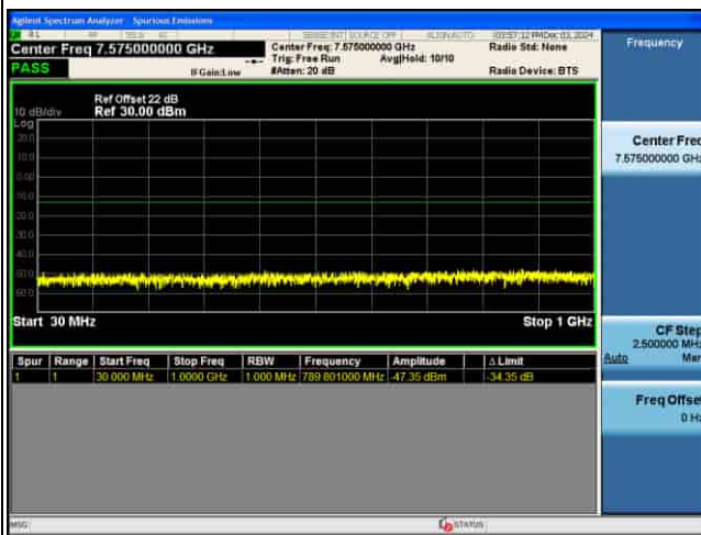
CSE_5G_n77(K)_30KHz_QPSK_50M CH631668_1RB@1
