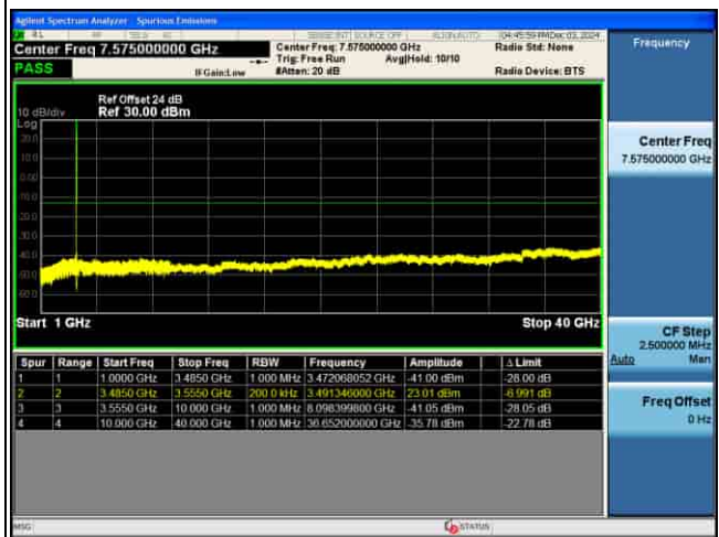
CSE_5G_n77(K)_30KHz_QPSK_70M CH632334_1RB@1_
