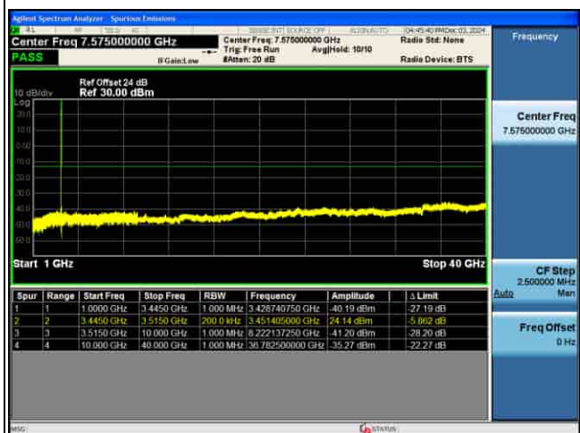
CSE_5G_n77(K)_30KHz_QPSK_60M CH633334_1RB@1_
