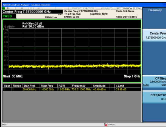
CSE_5G_n77(K)_30KHz_QPSK_20M CH630668_1RB@1
