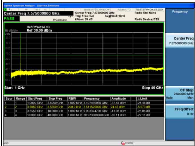
CSE_5G_n77(K)_30KHz_QPSK_50M CH631668_1RB@1_
