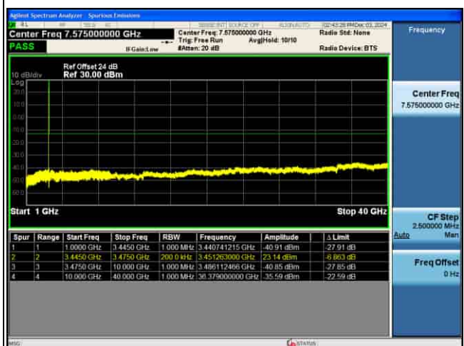
CSE_5G_n77(K)_30KHz_16QAM_20M CH630668_1RB@1_
