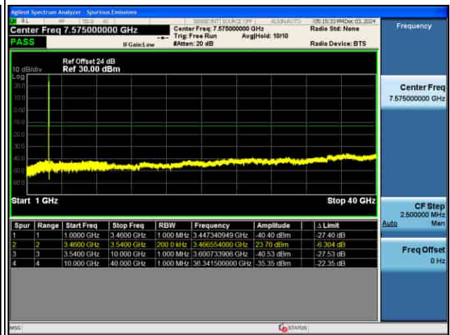
CSE_5G_n77(K)_30KHz_16QAM_70M CH634332_1RB@1_
