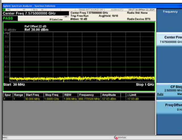
CSE_MIMO(ANT5)_n48_30KHz_QPSK_40M CH641666_1RB@1
