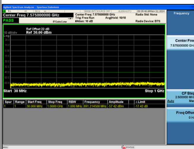
CSE_MIMO(ANT5)_n48_30KHz_QPSK_40M CH645332_1RB@1
