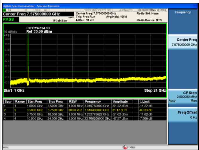
CSE_5G_n48_30KHz_QPSK_20M CH646000 1RB@1_
