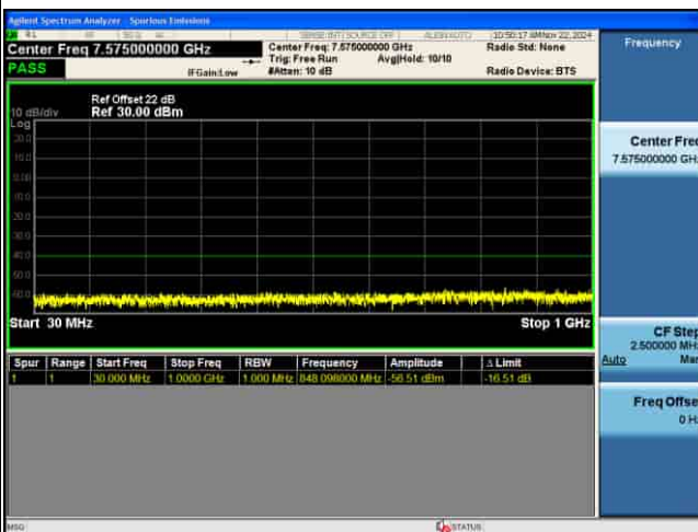
CSE_MIMO(ANT5)_n48_30KHz_QPSK_20M CH646000_1RB@1
