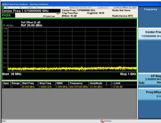
CSE_MIMO(ANT5)_n48_30KHz_QPSK_20M CH641666_1RB@1
