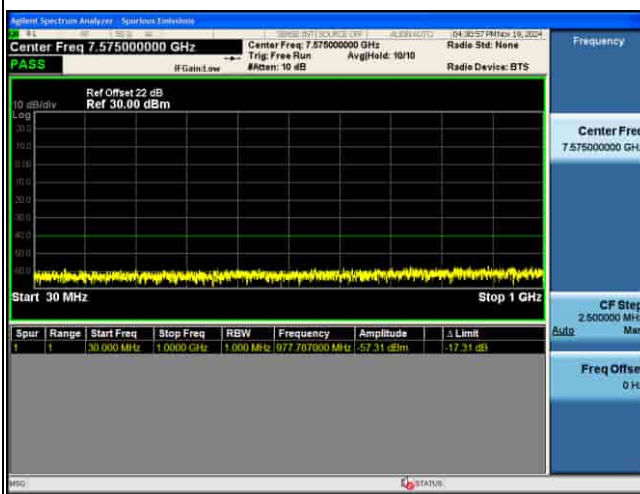
CSE_5G_n48_30KHz_16QAM_20M CH641666 1RB@1
