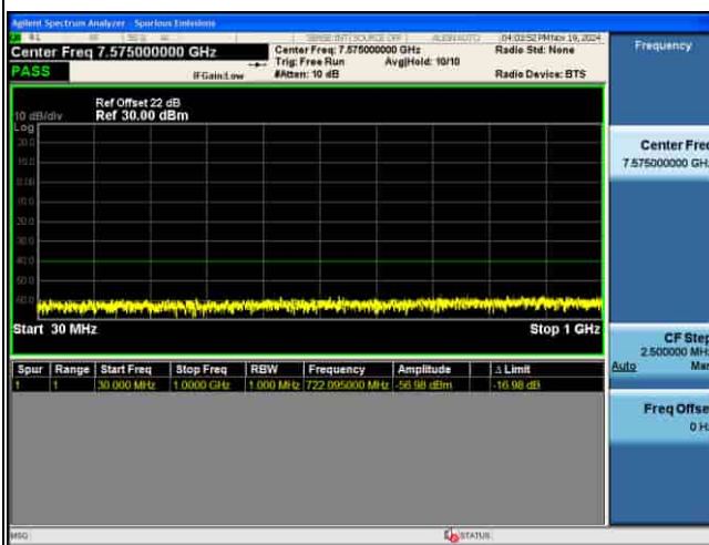
CSE_5G_n48_30KHz_.PI2-BPSK_30M CH641666 1RB@1_
