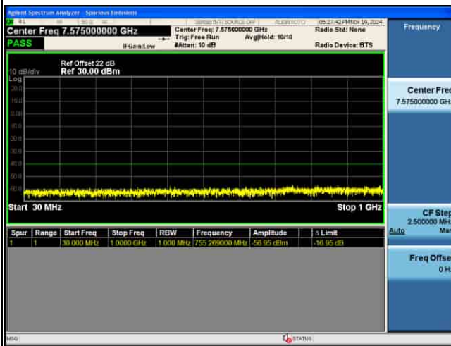
CSE_5G_n48_30KHz_QPSK_15M CH641666 1RB@1
