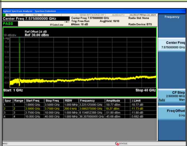
CSE_MIMO(ANT5)_n48_30KHz_QPSK_15M CH646166_1RB@1_
