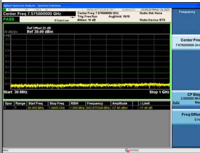
CSE_5G_n48_30KHz_QPSK_30M CH641666 1RB@1
