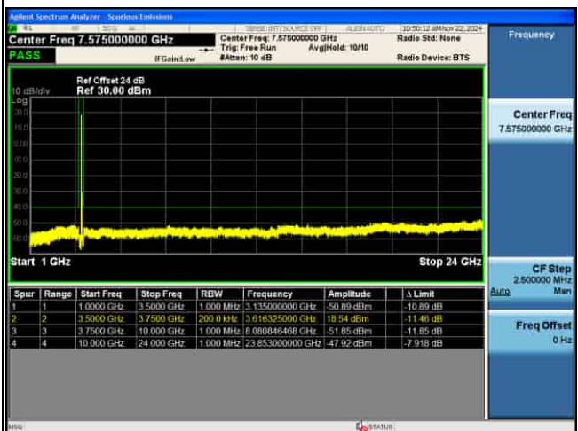
CSE_MIMO(ANT5)_n48_30KHz_QPSK_20M CH646000_1RB@1_
