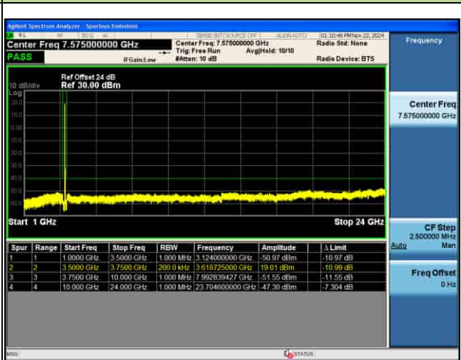
CSE_MIMO(ANT5)_n48_30KHz_QPSK_15M CH641666_1RB@1_
