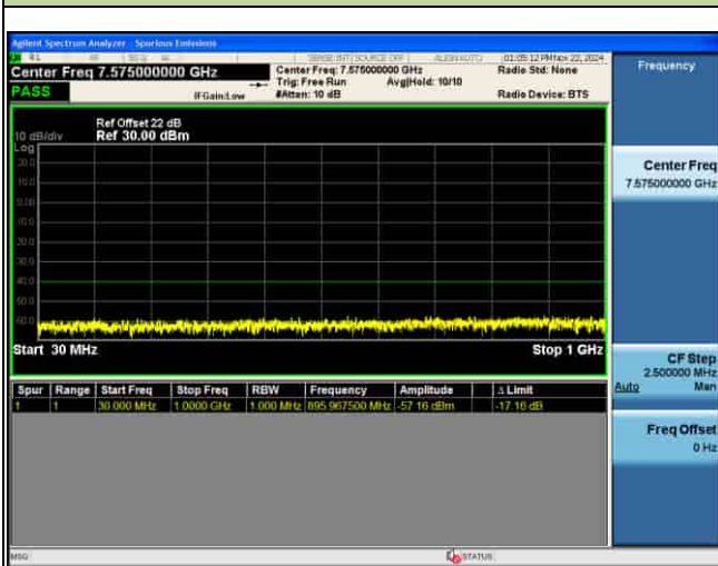
CSE_MIMO(ANT5)_n48_30KHz_QPSK_15M CH646166_1RB@1
