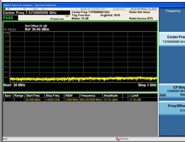
CSE_5G_n48_30KHz_.PI2-BPSK_40M CH641666 1RB@1_
