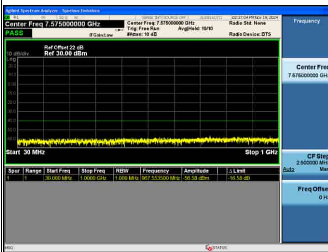
CSE_5G_n48_30KHz_QPSK_40M CH641666 1RB@1
