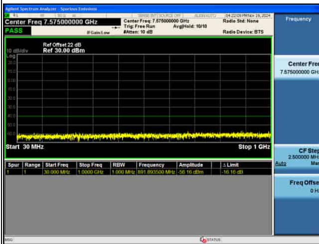
CSE_5G_n48_30KHz_QPSK_20M CH641666 1RB@1
