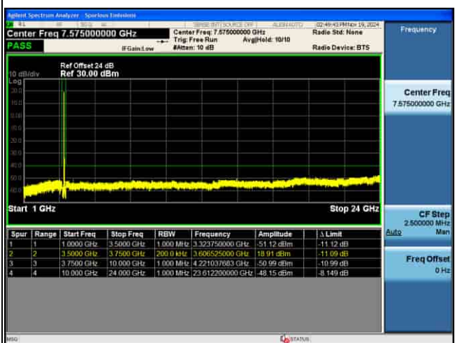
CSE_5G_n48_30KHz_QPSK_40M CH645332 1RB@1_
