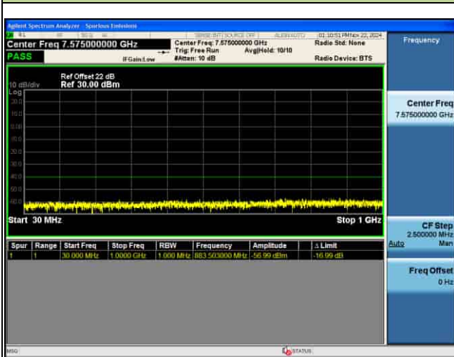
CSE_MIMO(ANT5)_n48_30KHz_QPSK_15M CH641666_1RB@1
