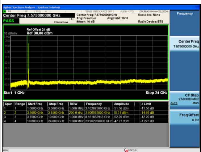
CSE_MIMO(ANT5)_n48_30KHz_QPSK_40M CH645332_1RB@1_
