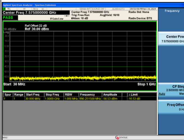
CSE_5G_n48_30KHz_QPSK_10M CH641666 1RB@1
