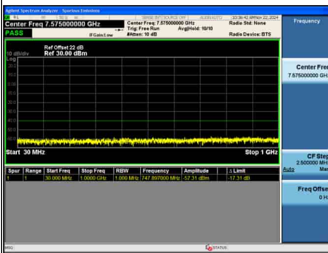
CSE_MIMO(ANT5)_n48_30KHz_QPSK_30M CH641666_1RB@1
