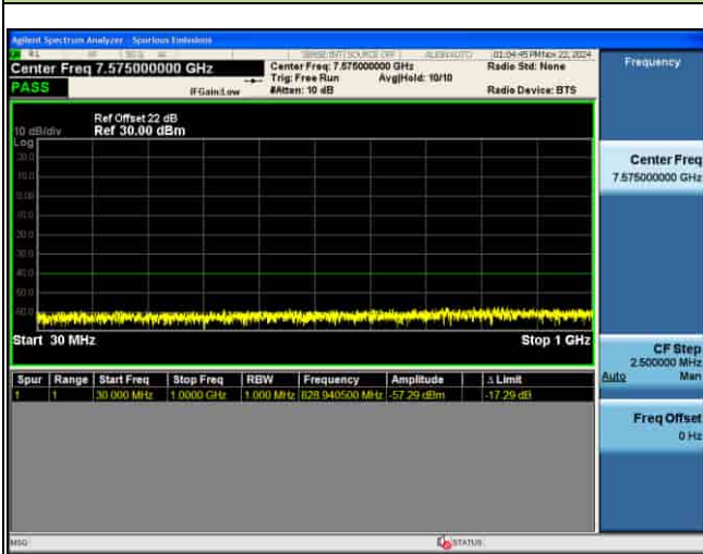
CSE_MIMO(ANT5)_n48_30KHz_QPSK_15M CH637168_1RB@1
