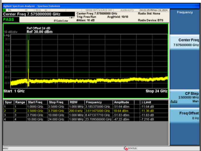
CSE_5G_n48_30KHz_QPSK_30M CH645666 1RB@1_
