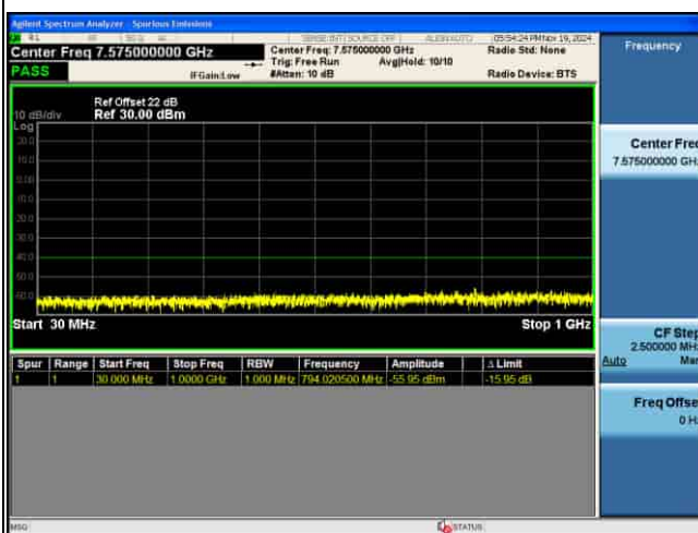
CSE_5G_n48_30KHz_QPSK_10M CH646332 1RB@1
