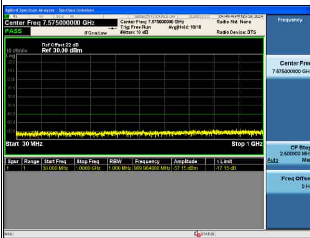
CSE_5G_n48_30KHz_256QAM_20M CH641666 1RB@1
