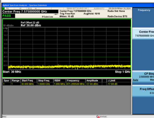
CSE_5G_n48_30KHz_QPSK_15M CH646166 1RB@1
