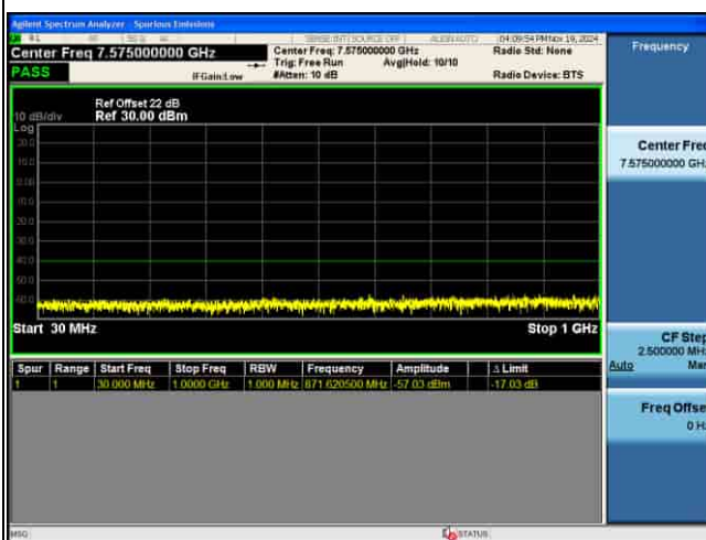
CSE_5G_n48_30KHz_.PI2-BPSK_30M CH645666 1RB@1_
