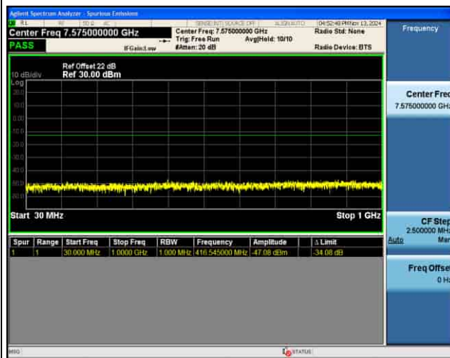
CSE_4G_B66_.QPSK_15M CH132597 1RB@0
