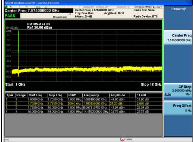
CSE_4G_B66_.QPSK_15M CH132597 1RB@0_
