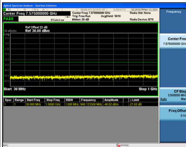
CSE_4G_B41_256QAM_20M CH41490 1RB@0
