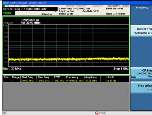
CSE_4G_B41_256QAM_20M CH41490 1RB@0
