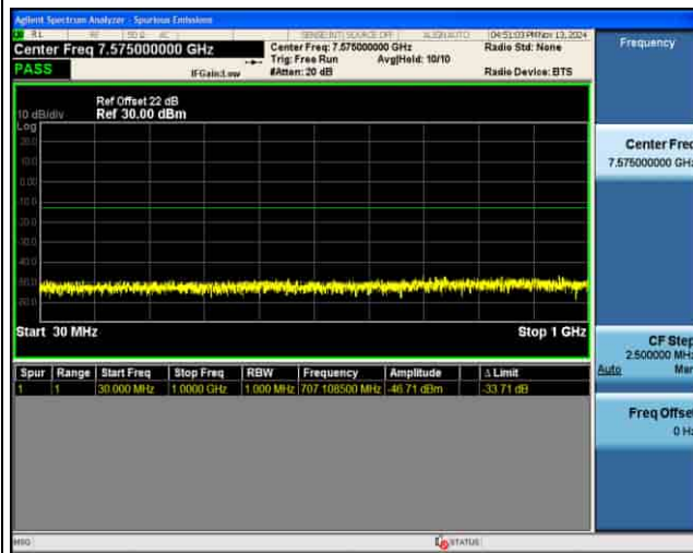
CSE_4G_B66_.QPSK_15M CH132322 1RB@0
