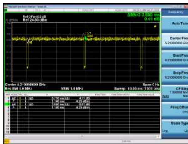
802.11 ac(80MHz)
