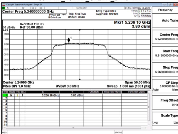
802.11n_20MHz_ChainA_5240MHz
