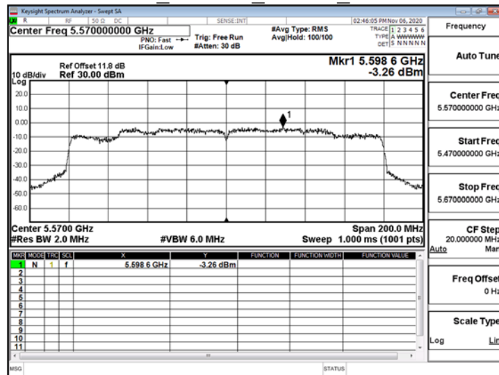
802.11ax_160MHz_ChainB_5570MHz
