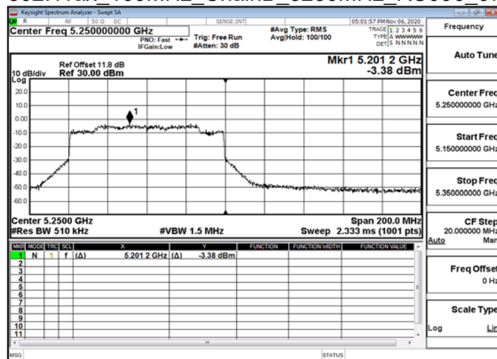
802.11ax_160MHz_ChainB_5250MHz_RU996_S67
