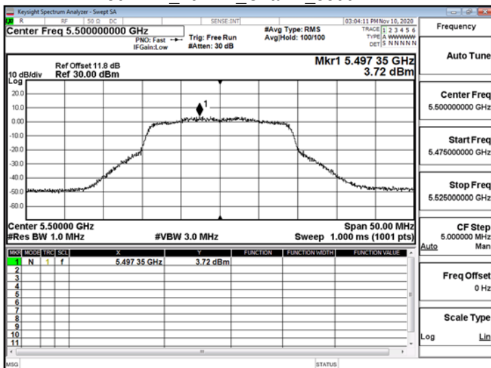
802.11n_20MHz_ChainB_5500MHz
