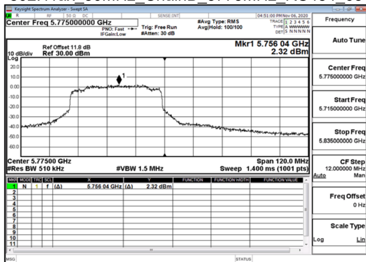
802.11ax_80MHz_ChainB_5775MHz_RU484_66
