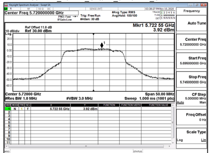
802.11n_20MHz_ChainB_5720MHz_UNII 2C
