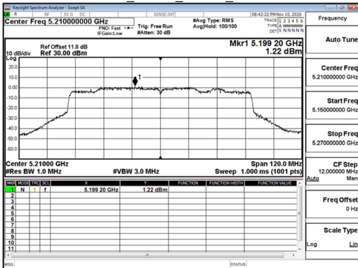
802.11ac_80MHz_ChainA_5210MHz
