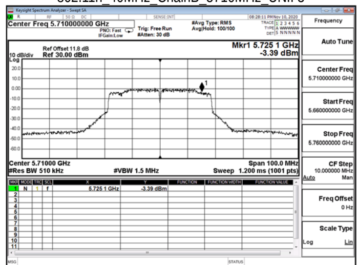
802.11n_40MHz_ChainB_5710MHz_UNII 3
