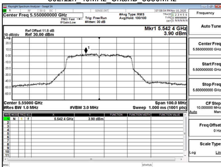
802.11n_40MHz_ChainB_5550MHz
