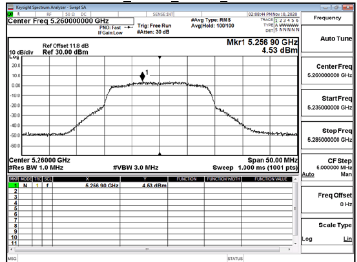
802.11n_20MHz_ChainB_5260MHz
