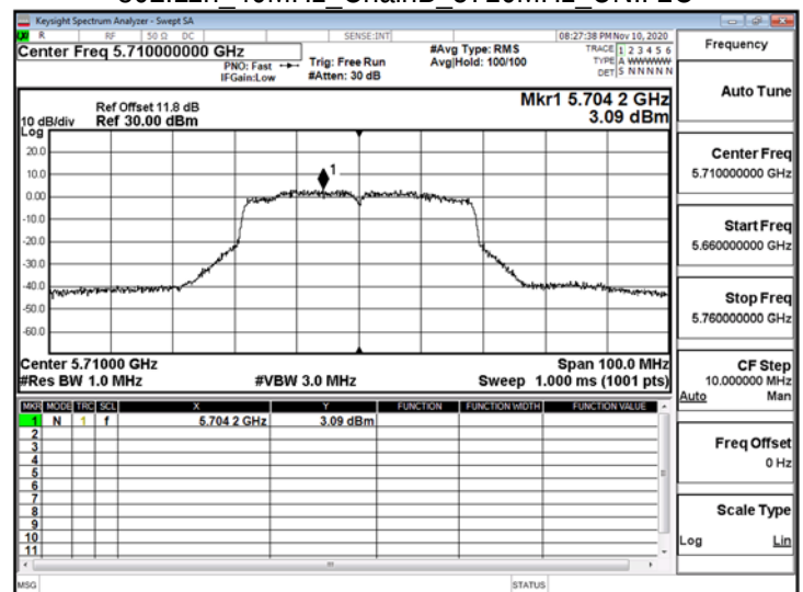
802.11n_40MHz_ChainB_5710MHz_UNII 3
