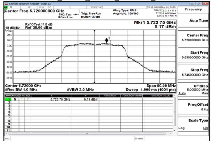
802.11n_20MHz_ChainA_5720MHz_UNII 3
