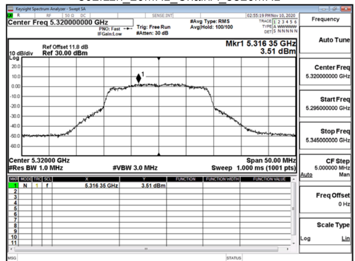
802.11n_20MHz_ChainA_5320MHz
