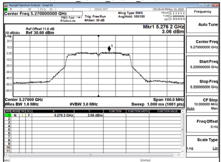
802.11n_40MHz_ChainB_5270MHz
