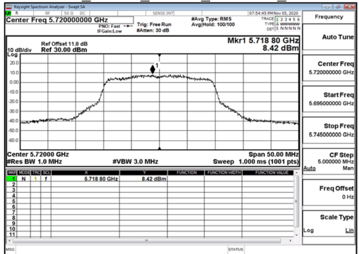
802.11ax 20MHz ChainB 5720MHz UNII 3
