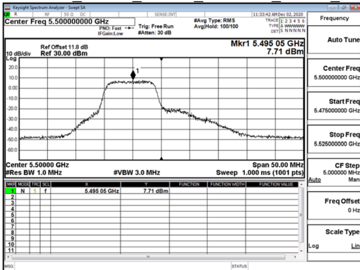
802.11ax 20MHz_ChainB_5500MHz_RU26_0
