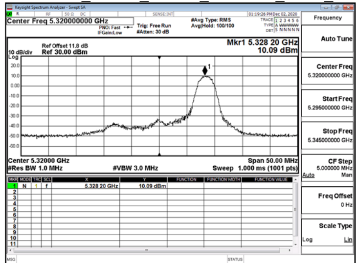
802.11ax 20MHz_ChainB_5320MHz_RU52_40
