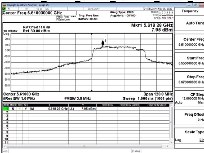
802.11ax 80MHz ChainB 5610MHz RU484 66
