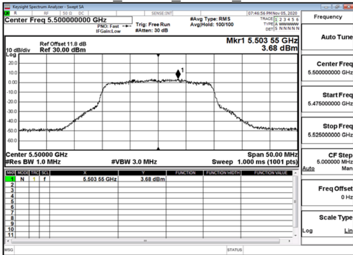
802.11ax 20MHz_ChainB_5500MHz_RU106_53
