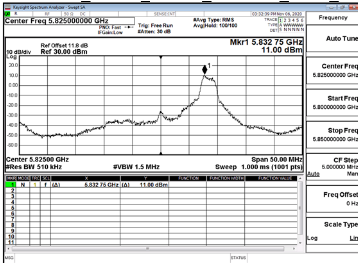
802.11ax 20MHz ChainB 5825MHz RU52 40
