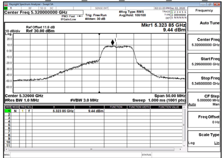
802.11ax 20MHz_ChainB_5320MHz_RU26_8
