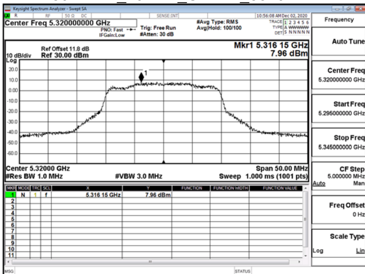
802.11ax 20MHz_ChainB_5320MHz
