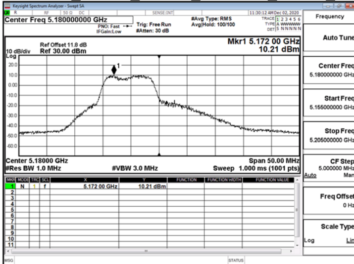
802.11ax 20MHz_ChainB_5180MHz_RU26_0
