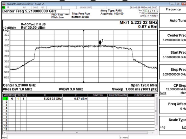
802.11ax 80MHz ChainB 5210MHz RU484 65
