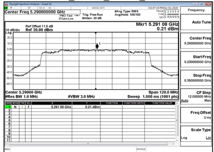
802.11ax 80MHz ChainB 5290MHz RU484 66
