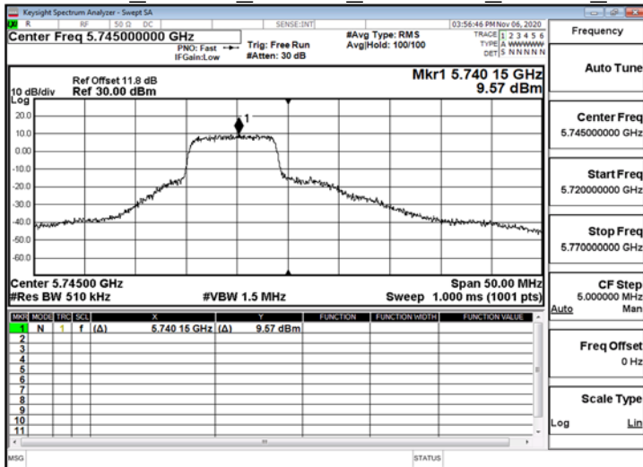
802.11ax 20MHz ChainB 5745MHz RU26 0
