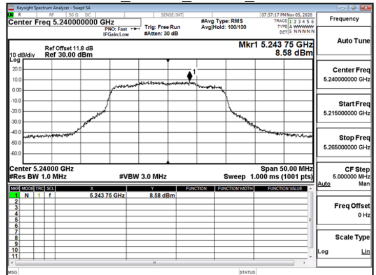
802.11ax 20MHz_ChainB_5240MHz
