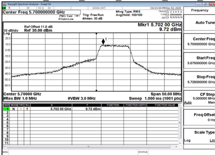
802.11ax 20MHz ChainB 5700MHz RU26 8
