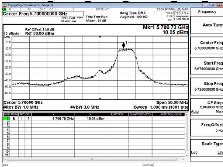
802.11ax 20MHz ChainB 5700MHz RU52 40
