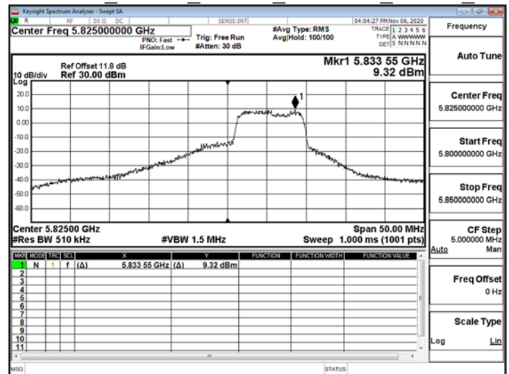
802.11ax 20MHz ChainB 5825MHz RU106 54
