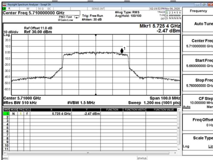
802.11ax_40MHz_ChainB_5710MHz_UNII 3
