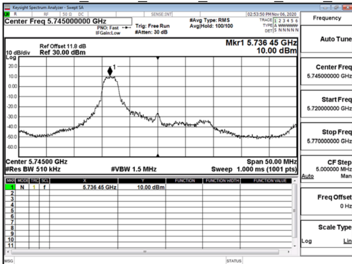
802.11ax 20MHz ChainB 5745MHz RU52 37
