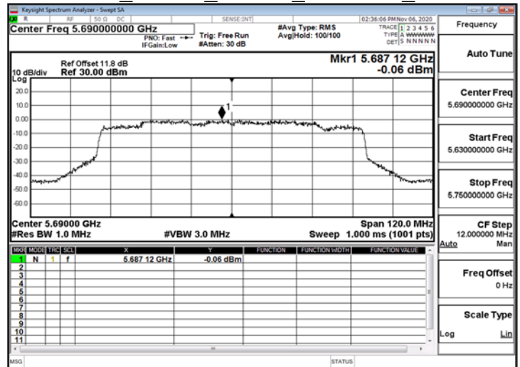
802.11ax 80MHz ChainB 5690MHz UNII 3
