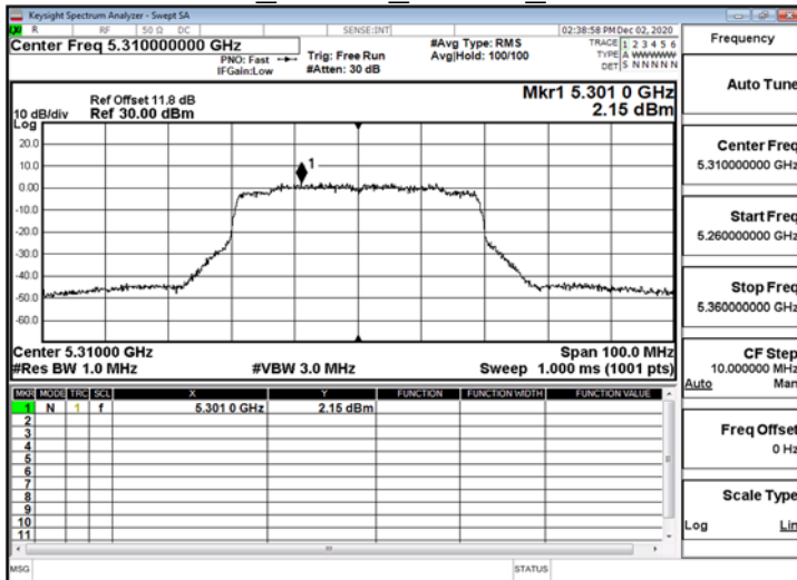
802.11ax_40MHz_ChainB_5310MHz_RU242_62
