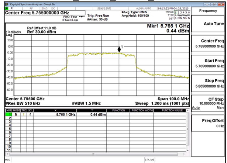
802.11ax_40MHz_ChainB_5755MHz_RU242_61
