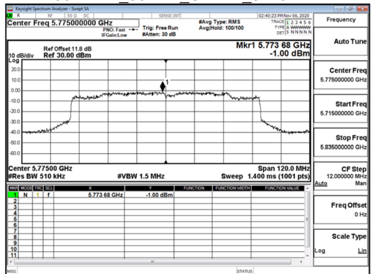
802.11ax 80MHz ChainB 5775MHz
