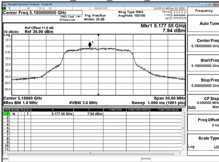
802.11ax 20MHz_ChainB_5180MHz_RU106_53
