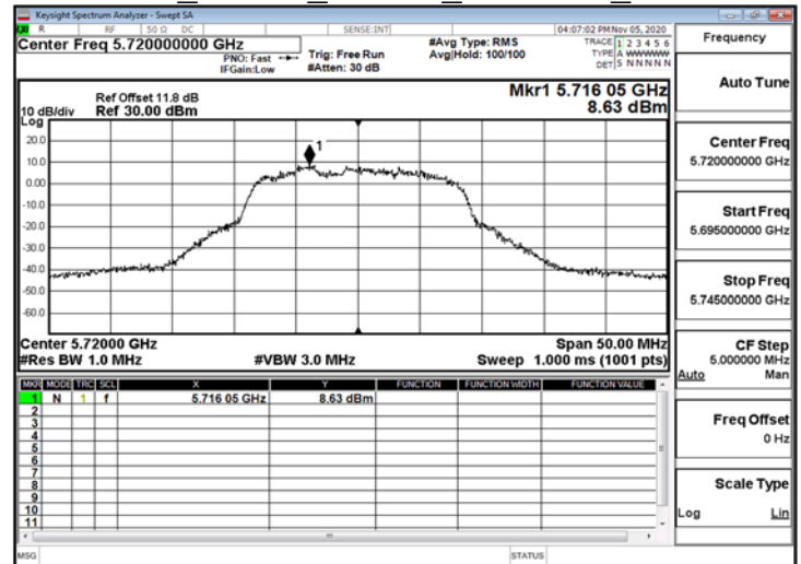
802.11a_20MHz_ChainB_5720MHz_UNII 3
