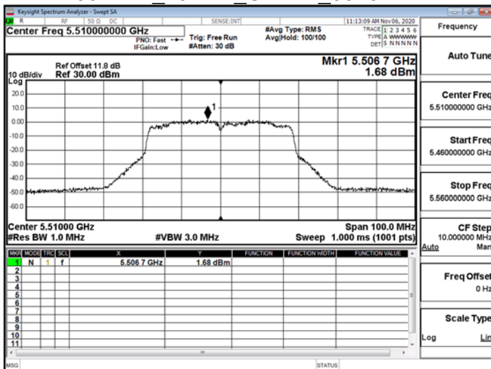
802.11n_40MHz_ChainB_5510MHz
