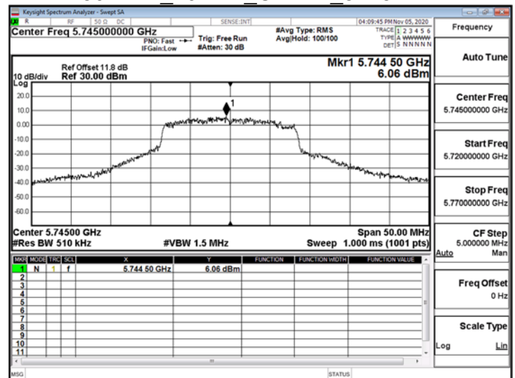
802.11a_20MHz_ChainB_5745MHz
