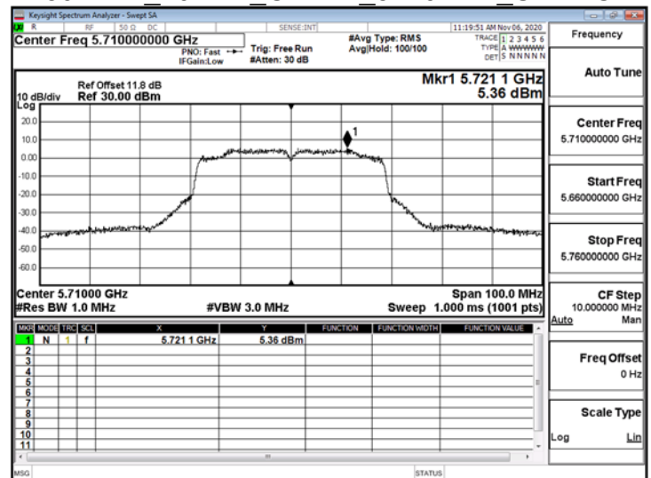
802.11n_40MHz_ChainB_5710MHz_UNII_2C
