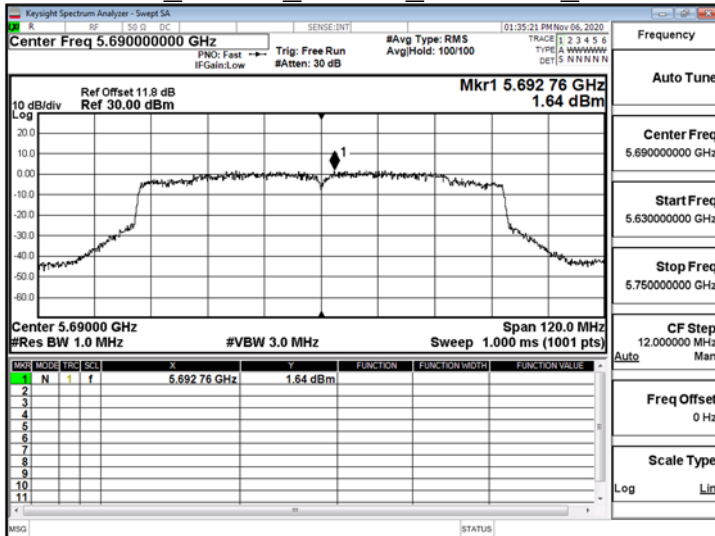
802.11ac_80MHz_ChainB_5690MHz_UNII 3
