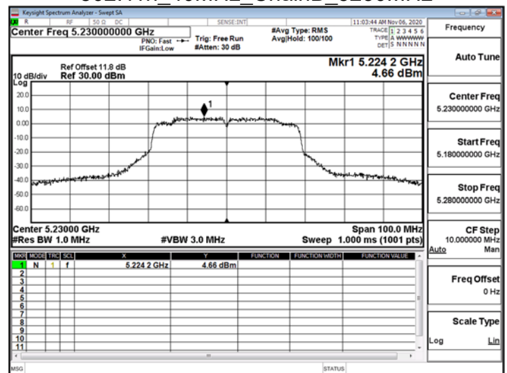
802.11n 40MHz ChainB 5230MHz
