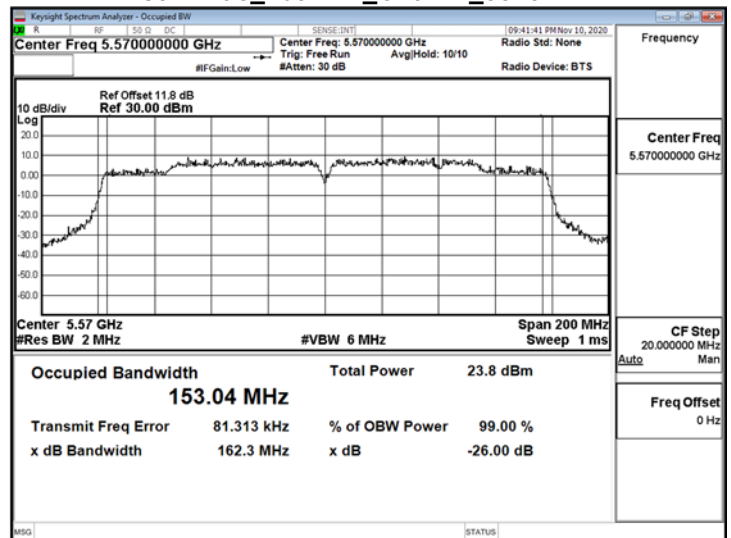
802.11ac_160MHz_ChainA_5570MHz
