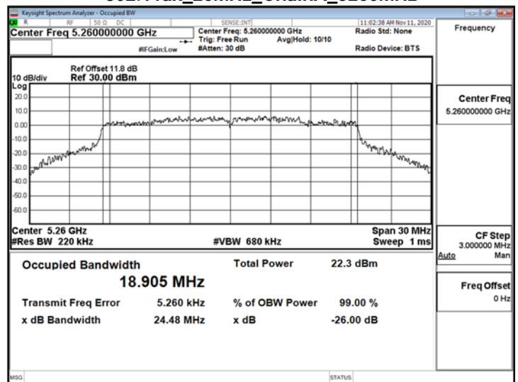
802.11ax_20MHz_ChainA_5260MHz
