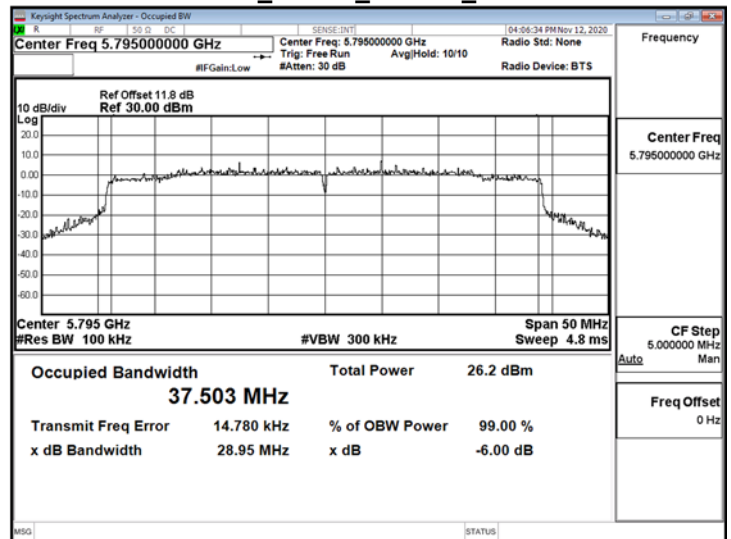
802.11ax_40MHz_ChainB_5795MHz
