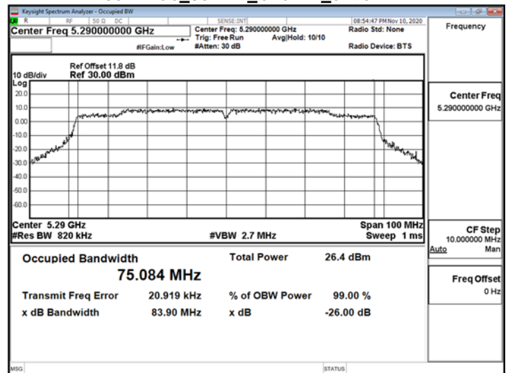
802.11ac_80MHz_ChainA_5290MHz
