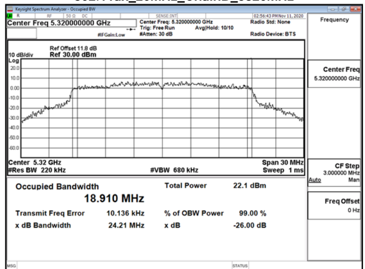
802.11ax_20MHz_ChainB_5320MHz
