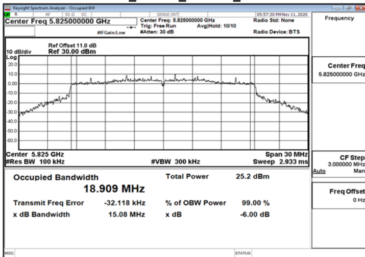
802.11ax_20MHz_ChainB_5825MHz
