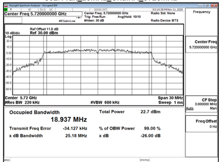
802.11ax_20MHz_ChainA_5720MHz
