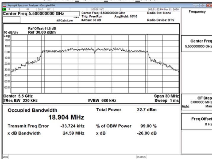
802.11ax_20MHz_ChainA_5500MHz
