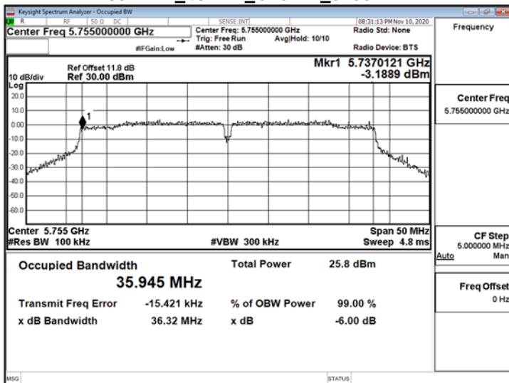
802.11n_40MHz_ChainB_5755MHz
