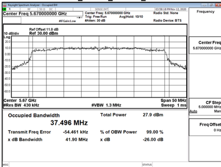
802.11ax_40MHz_ChainB_5670MHz
