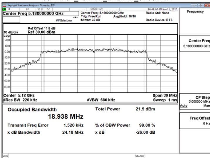
802.11ax_20MHz_ChainA_5180MHz
