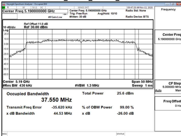
802.11ax_40MHz_ChainB_5190MHz
