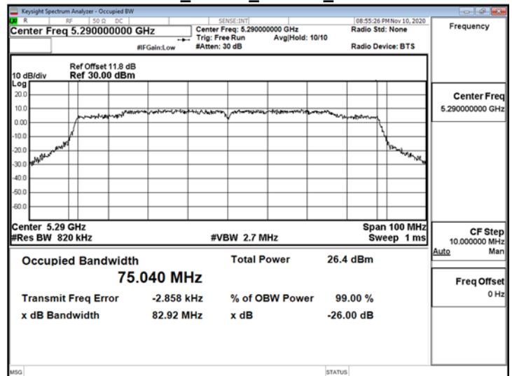
802.11ac_80MHz_ChainB_5290MHz
