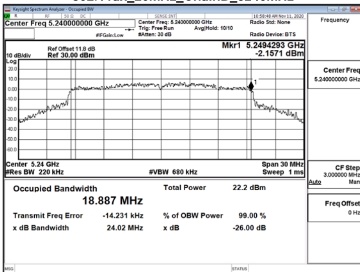
802.11ax_20MHz_ChainB_5240MHz
