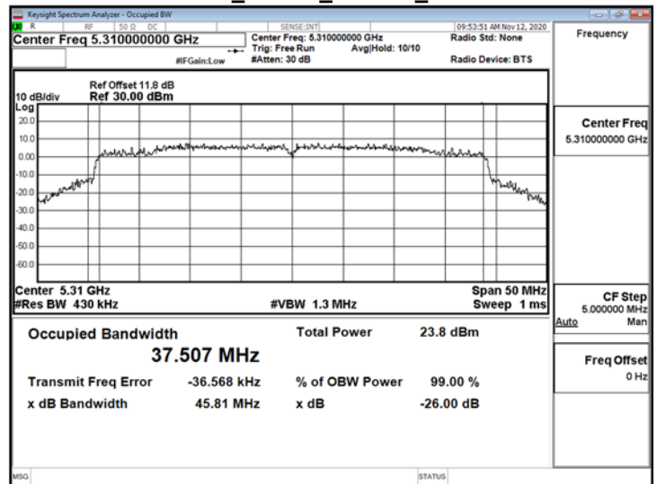
802.11ax_40MHz_ChainB_5310MHz
