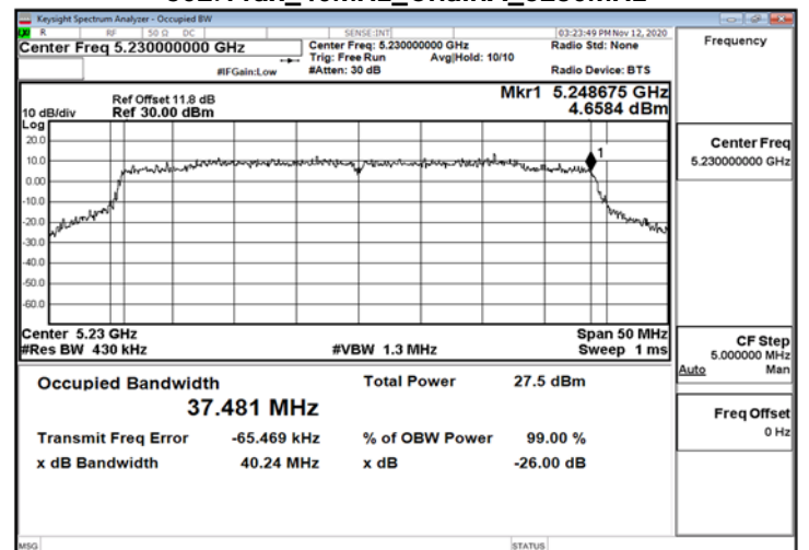
802.11ax_40MHz_ChainA_5230MHz
