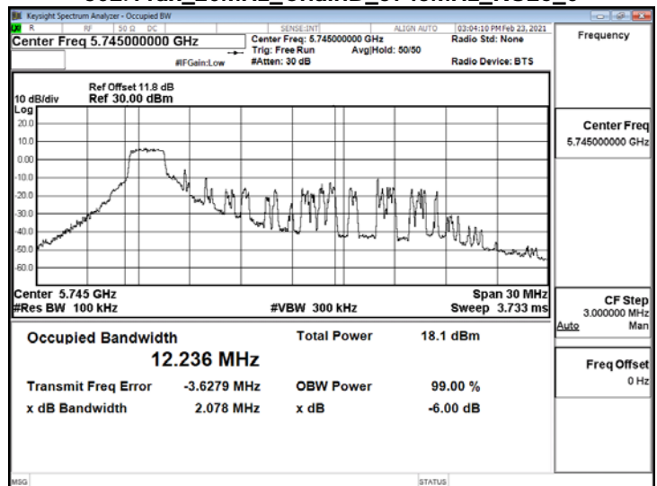
802.11ax_20MHz_ChainB_5745MHz_RU26_0
