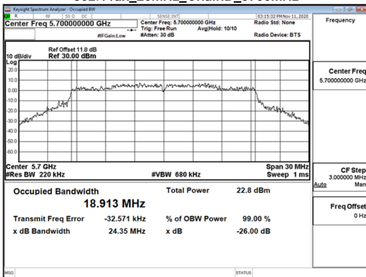
802.11ax_20MHz_ChainB_5700MHz
