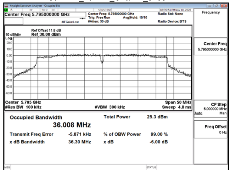
802.11n 40MHz ChainA 5795MHz
