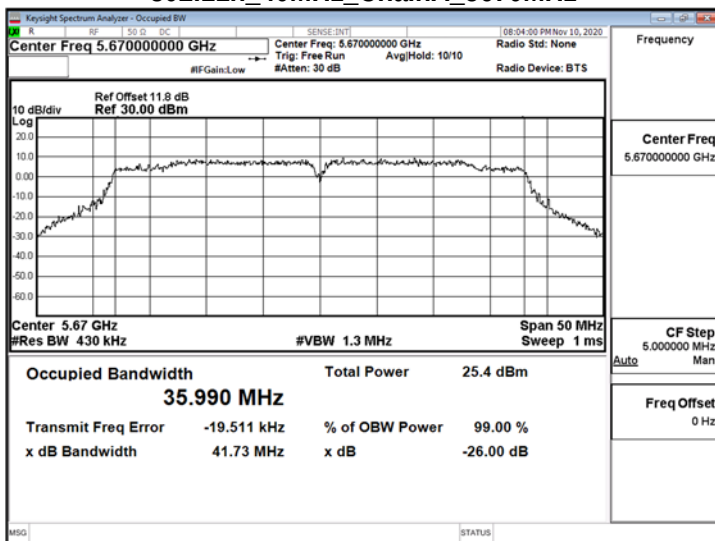
802.11n 40MHz ChainA 5670MHz
