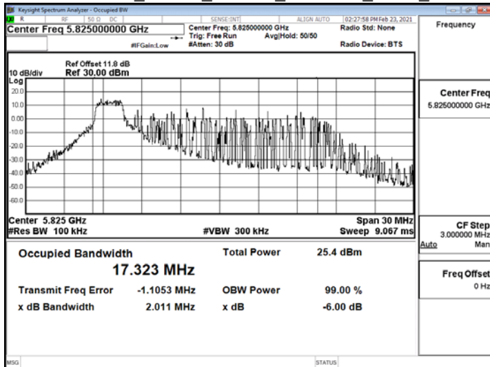
802.11ax 20MHz ChainB 5825MHz RU26 0
