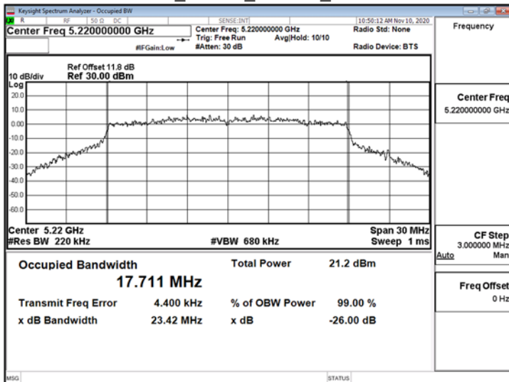
802.11n 20MHz_ChainB 5220MHz
