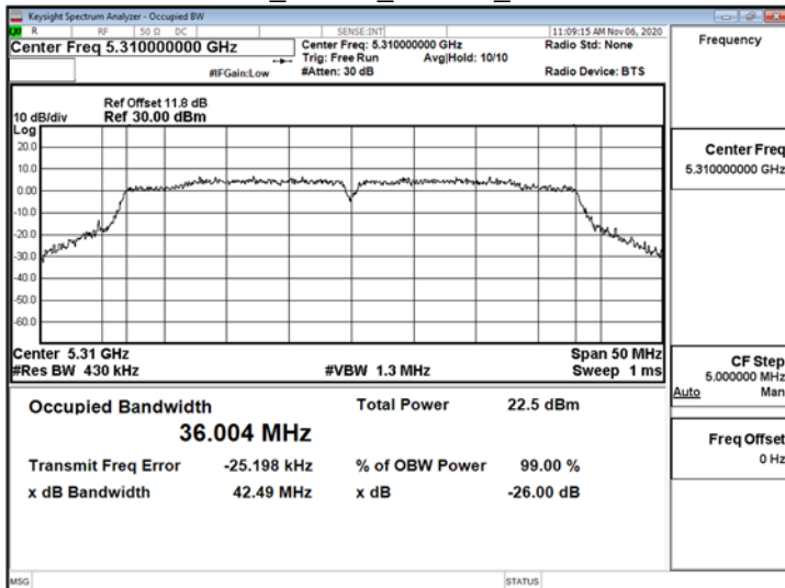
802.11n 40MHz ChainB 5310MHz
