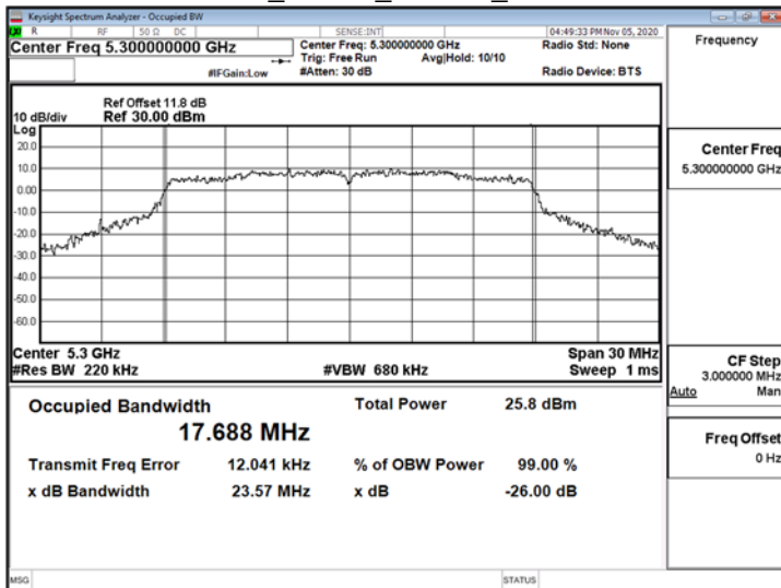
802.11n 20MHz_ChainB 5300MHz
