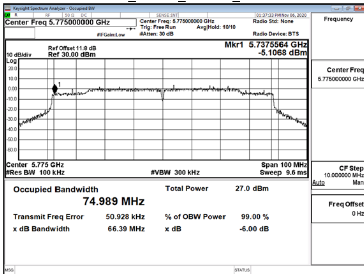
802.11ac_80MHz_ChainB_5775MHz
