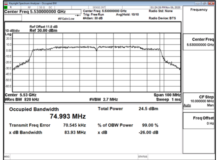
802.11ac_80MHz_ChainB_5530MHz
