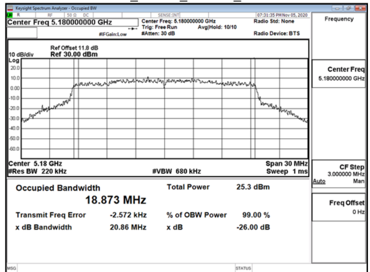
802.11ax_20MHz_ChainB_5180MHz
