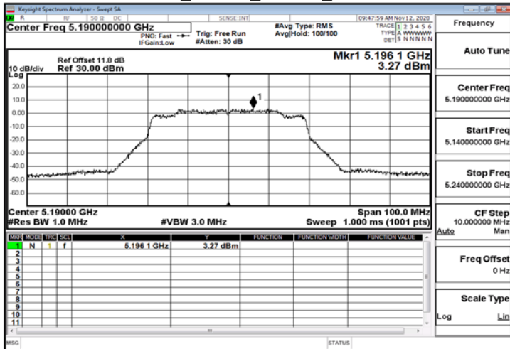
802.11ax_40MHz_ChainA_5190MHz_RU242_61
