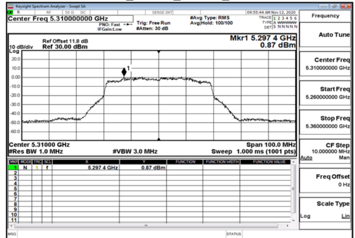
802.11ax_40MHz_ChainB_5310MHz_RU242_62
