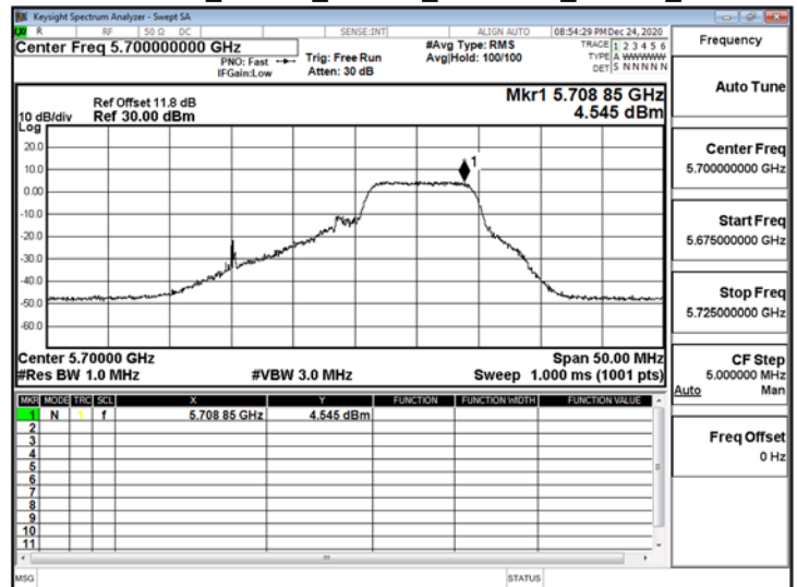
802.11ax_20MHz_ChainB_5700MHz_RU26_8
