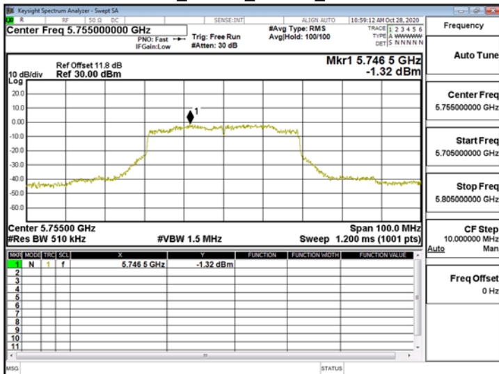
802.11ax_40MHz_ChainA_5755MHz_RU242_61
