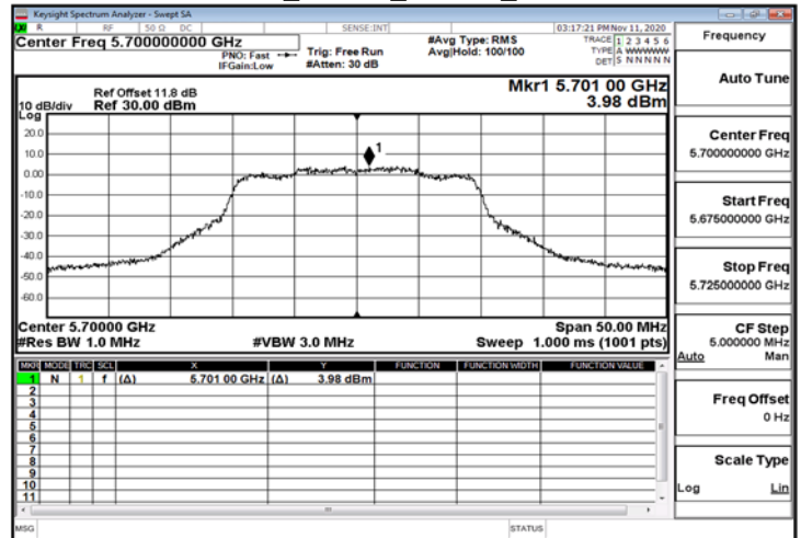
802.11ax_20MHz_ChainB_5700MHz_RU106_54
