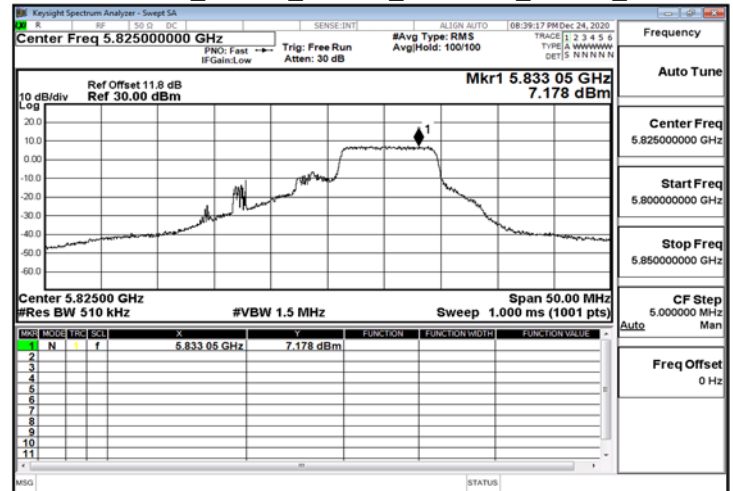
802.11ax_20MHz_ChainB_5825MHz_RU26_0
