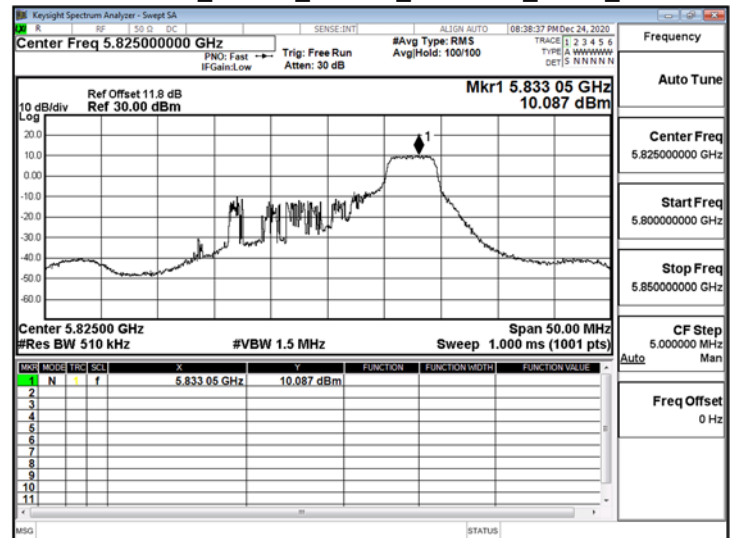
802.11ax_20MHz_ChainB_5825MHz_RU52_40
