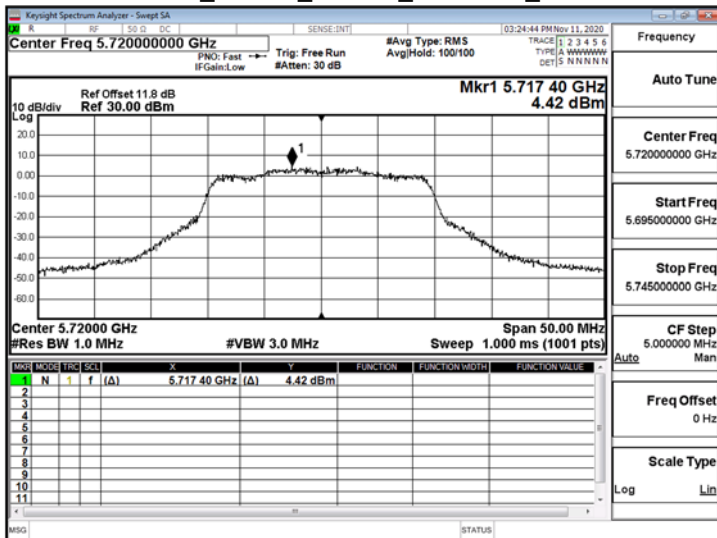
802.11ax_20MHz_ChainB_5720MHz_UNII 3
