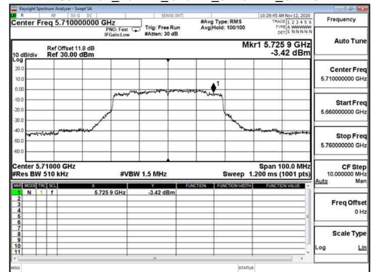
802.11ax_40MHz_ChainB_5710MHz_UNII 3
