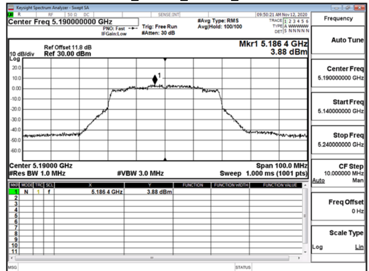
802.11ax_40MHz_ChainB_5190MHz
