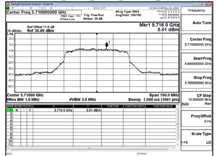
802.11ax_40MHz_ChainB_5710MHz_UNII 3
