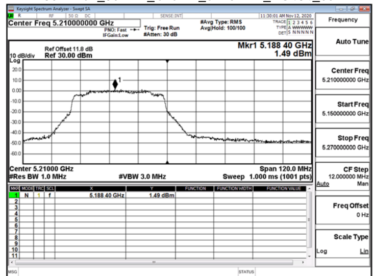
802.11ax_80MHz_ChainA_5210MHz_RU484_65
