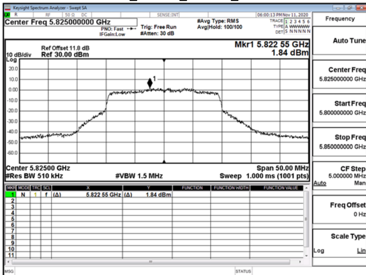
802.11ax_20MHz_ChainB_5825MHz
