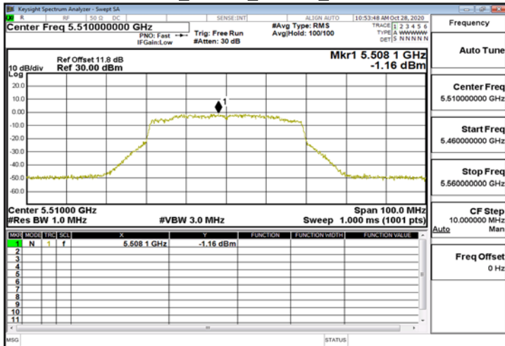
802.11ax_40MHz_ChainA_5510MHz_RU242_61
