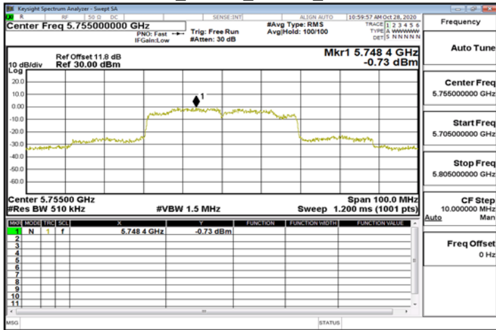
802.11ax_40MHz_ChainB_5755MHz_RU242_61
