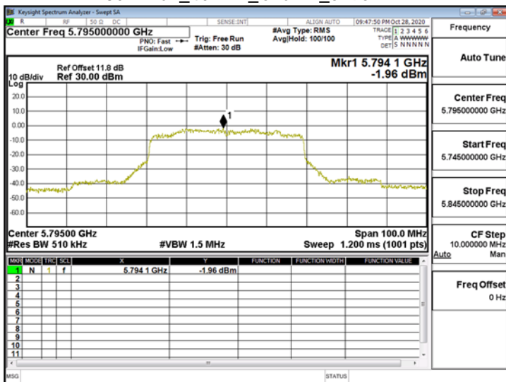
802.11ax_40MHz_ChainB_5795MHz
