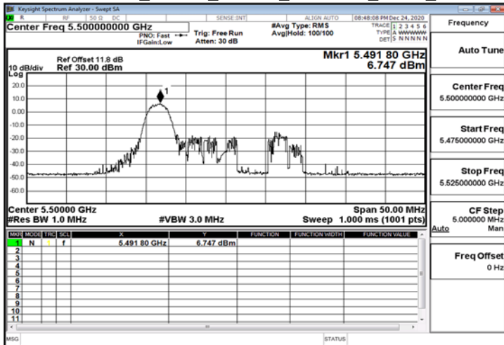
802.11ax_20MHz_ChainB_5500MHz_RU52_37
