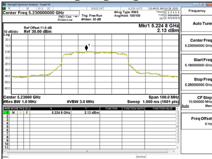
802.11ax_40MHz_ChainA_5230MHz
