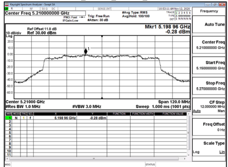
802.11ax_80MHz_ChainA_5210MHz_RU484_65
