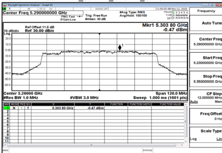
802.11ax_80MHz_ChainA_5290MHz_RU484_66
