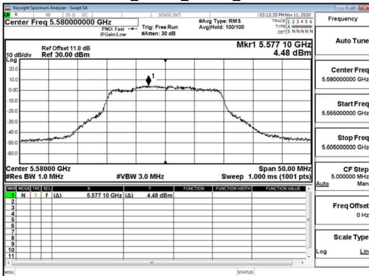
802.11ax_20MHz_ChainB_5580MHz
