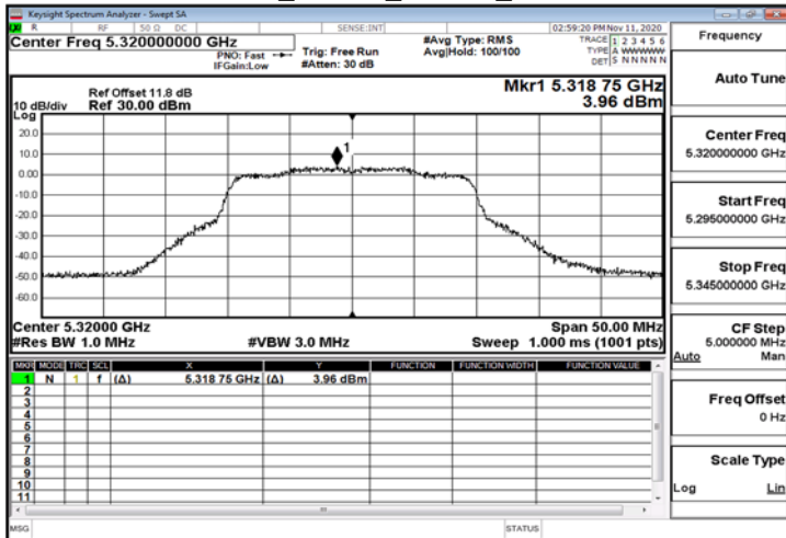
802.11ax_20MHz_ChainB_5320MHz_RU106_54
