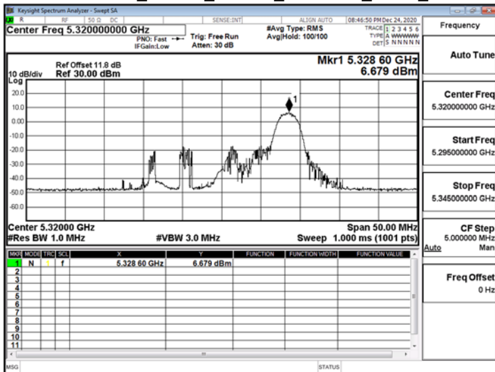
802.11ax_20MHz_ChainB_5320MHz_RU26_8
