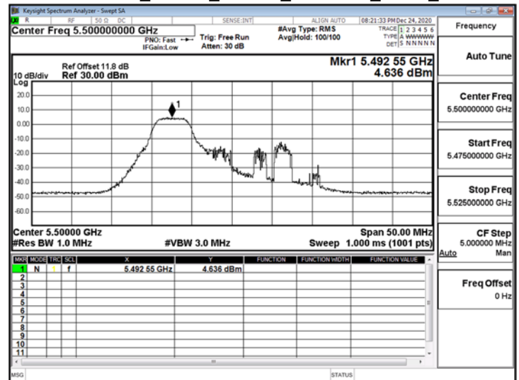
802.11ax_20MHz_ChainA_5500MHz_RU52_37
