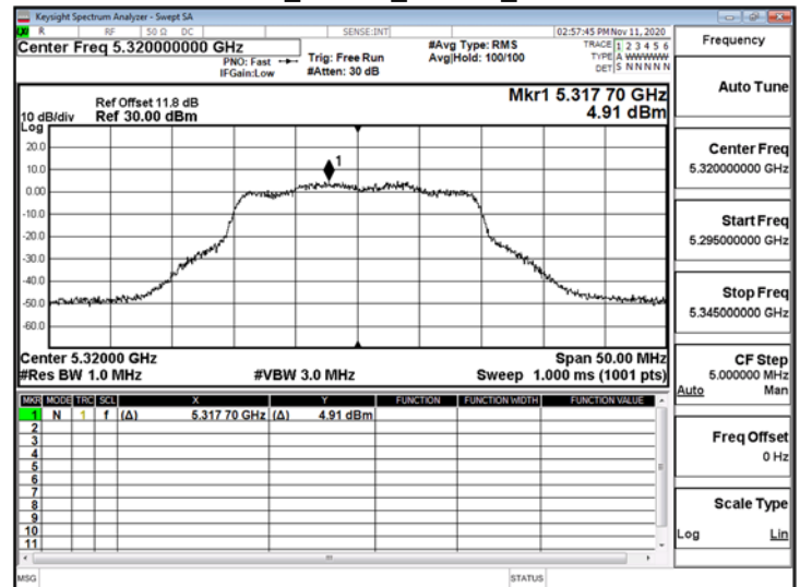
802.11ax_20MHz_ChainA_5320MHz_RU106_54
