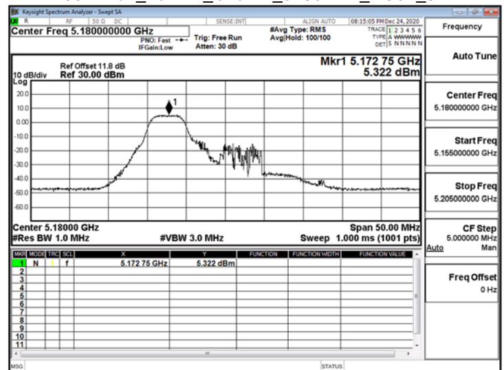
802.11ax_20MHz_ChainA_5180MHz_RU52_37
