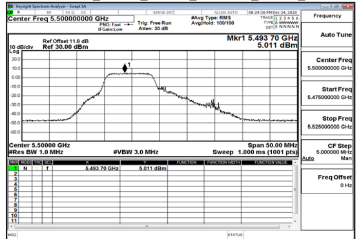
802.11ax_20MHz_ChainA_5500MHz_RU26_0
