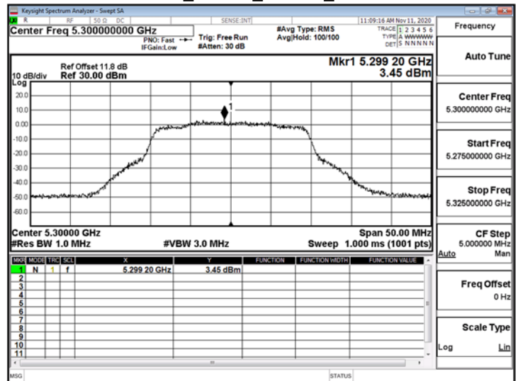
802.11ax_20MHz_ChainB_5300MHz
