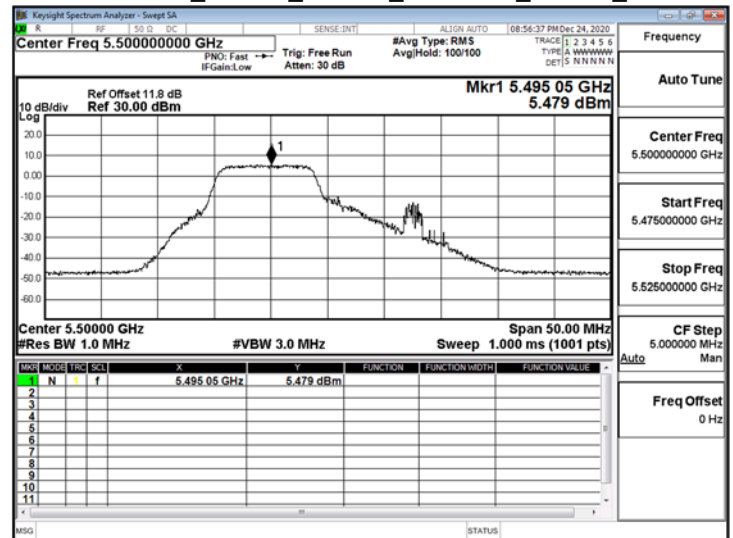
802.11ax_20MHz_ChainB_5500MHz_RU106_53
