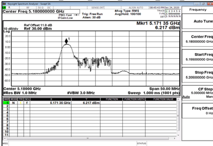
802.11ax_20MHz_ChainB_5180MHz_RU52_37
