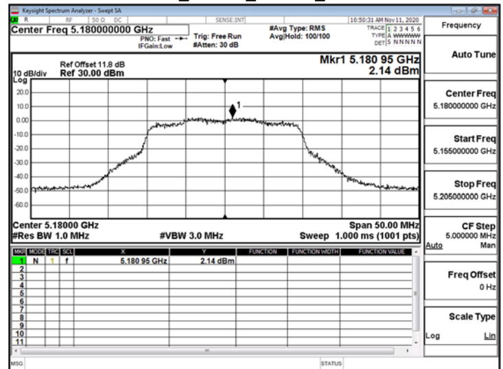
802.11ax_20MHz_ChainB_5180MHz_RU106_53
