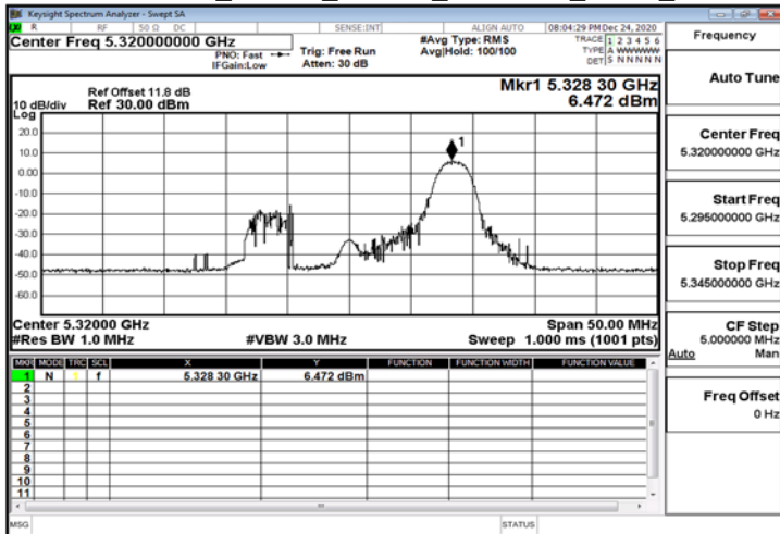
802.11ax_20MHz_ChainA_5320MHz_RU52_40
