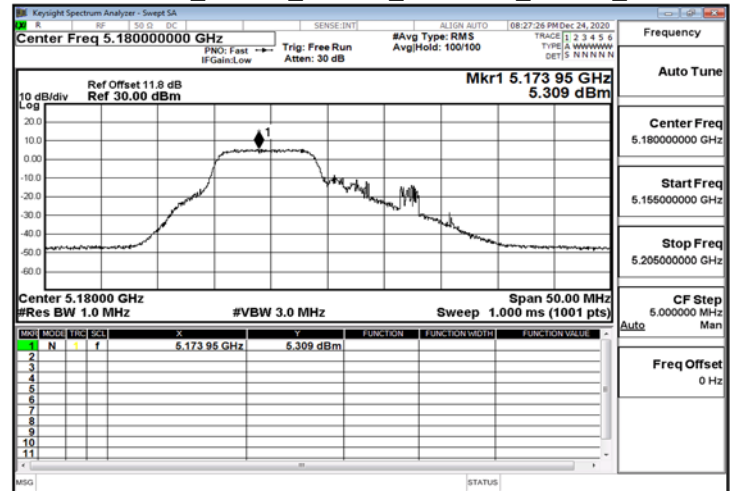
802.11ax_20MHz_ChainA_5180MHz_RU26_0
