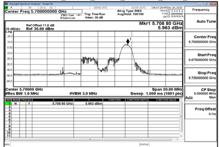
802.11ax_20MHz_ChainA_5700MHz_RU52_40
