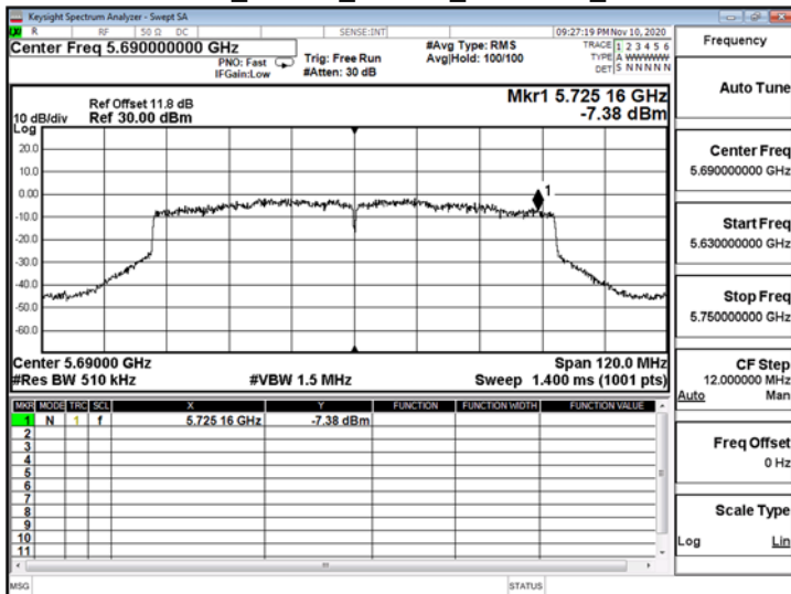
802.11ac_80MHz_ChainB_5690MHz_UNII 3
