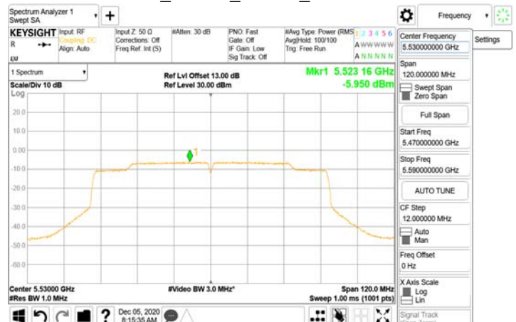
802.11ac_80MHz_Chain1_5530MHz-5530
