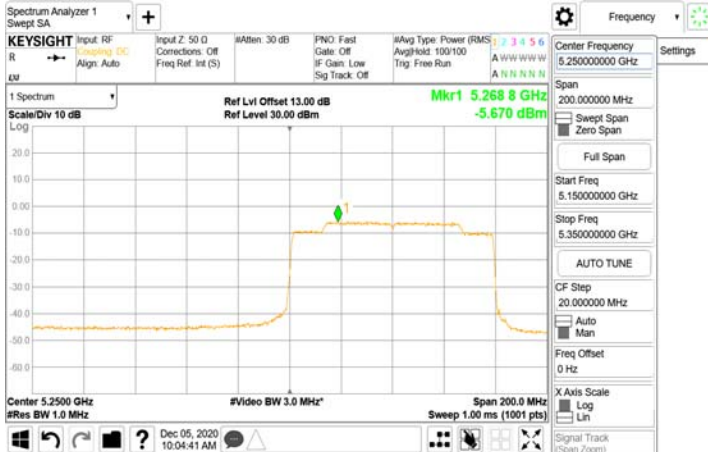
802.11ax_160MHz_Chian1_5250MHz -996-S67
