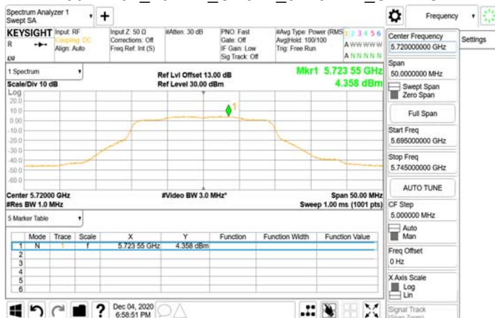
802.11ax_20MHz_Chian1_5720MHz_UNII 3
