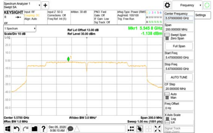
802.11ax_160MHz_Chian1_5570MHz-996-67
