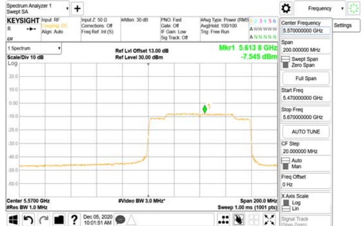
802.11ax_160MHz_Chian1_5570MHz-996-S67
