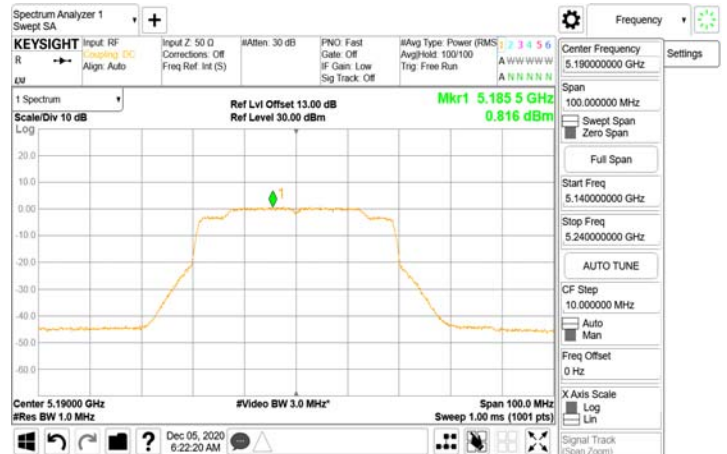
802.11ax_40MHz_Chian1_5190MHz-242-61
