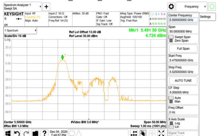
802.11ax_20MHz_Chain1_5500MHz-26-0
