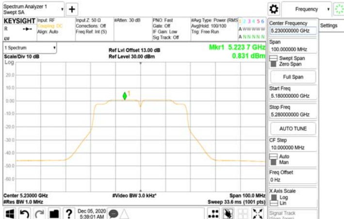
802.11n_40MHz_Chian1_5230MHz-5230
