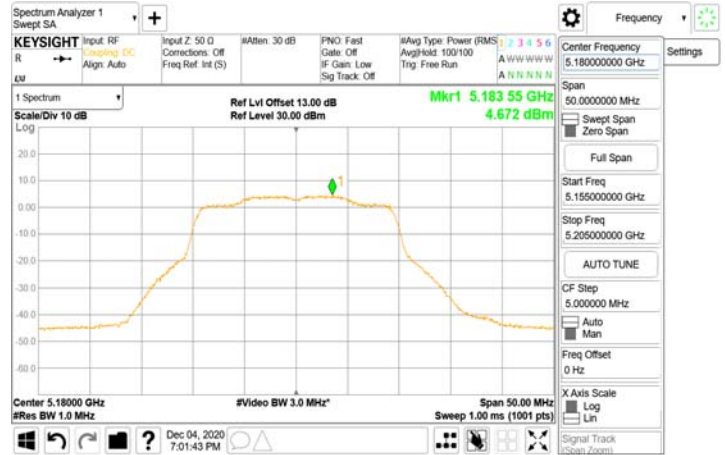
802.11ax_20MHz_Chain1_5180MHz-106-53
