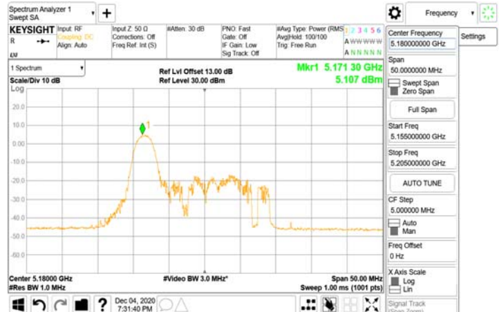
802.11ax_20MHz_Chain1_5180MHz-26-0
