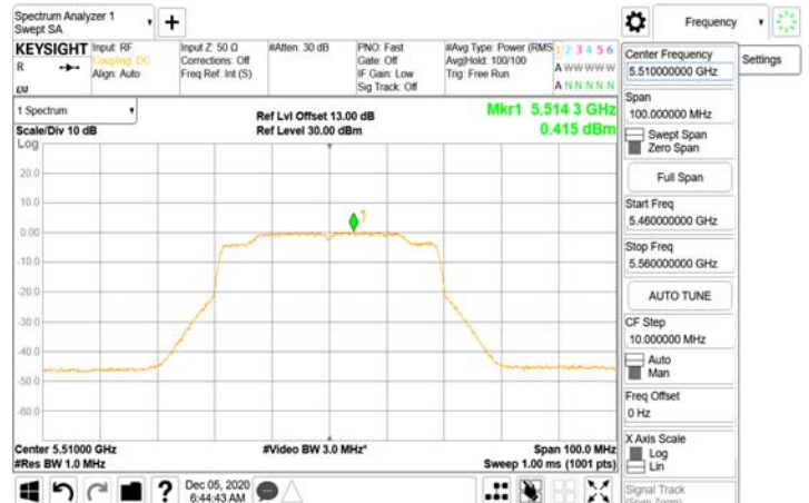
802.11ax_40MHz_Chian1_5510MHz-242-61
