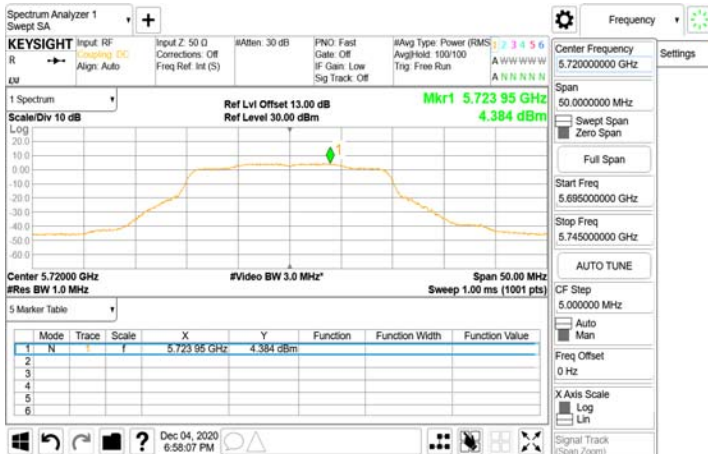
802.11ax_20MHz_Chian0_5720MHz_UNII 3
