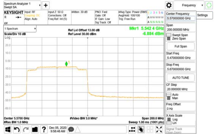
802.11ax_160MHz_Chian1_5570MHz-996-S67
