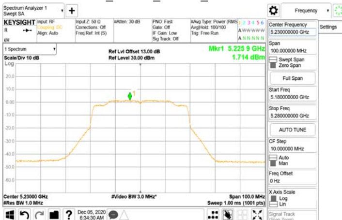
802.11ax_40MHz_Chian0_5230MHz-5230
