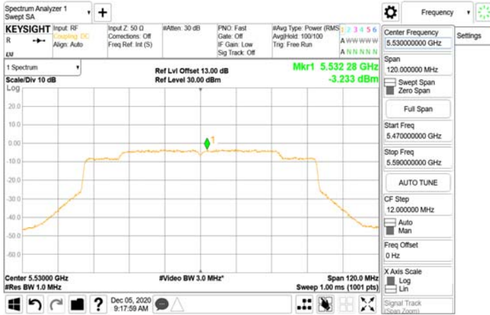
802.11ax_80MHz_Chian1_5530MHz-484-65
