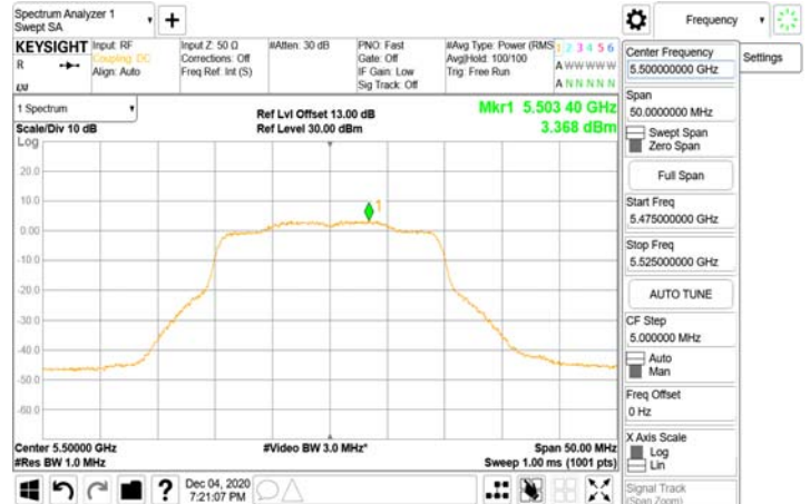
802.11ax_20MHz_Chian1_5500MHz-106-53
