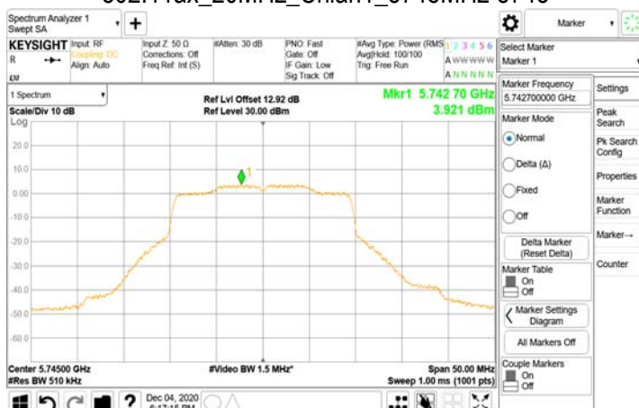
802.11ax_20MHz_Chian1_5745MHz-5745
