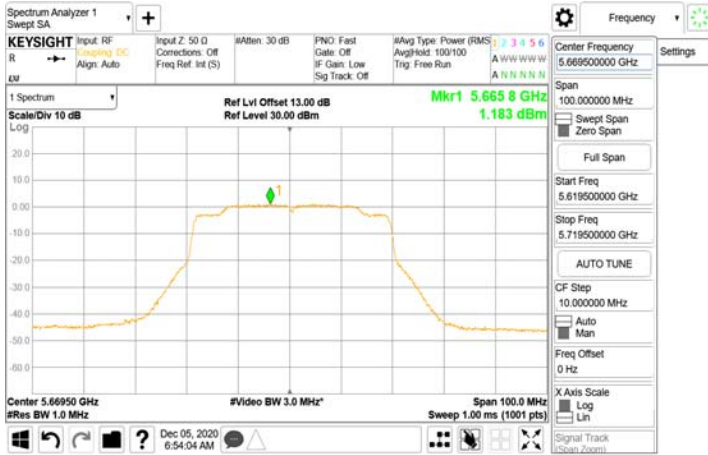
802.11ax_40MHz_Chian1_5670MHz-242-62
