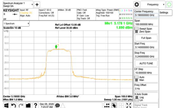
802.11ax_40MHz_Chian1_5190MHz-242-61
