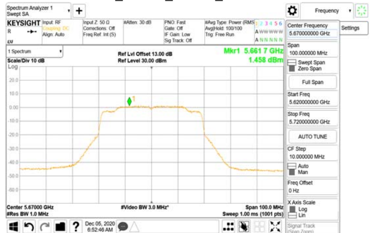
802.11ax_40MHz_Chian0_5670MHz-242-62
