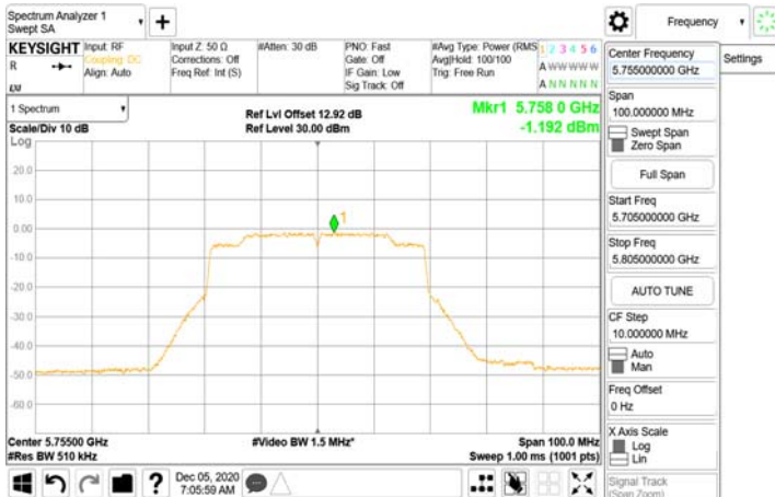
802.11ax_40MHz_Chian0_5755MHz-242-61
