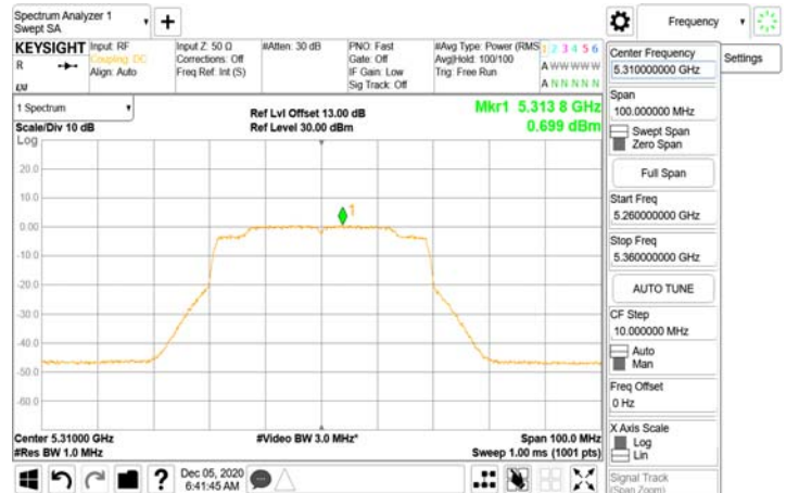
802.11ax_40MHz_Chian0_5310MHz-242-62
