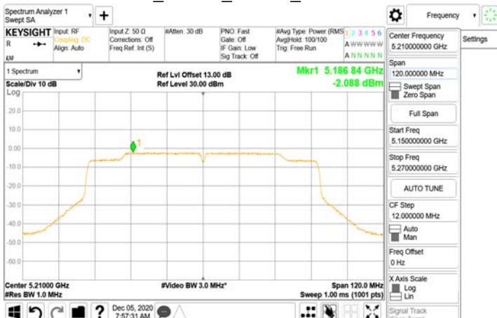
802.11ac_80MHz_Chian0_5210MHz-5210
