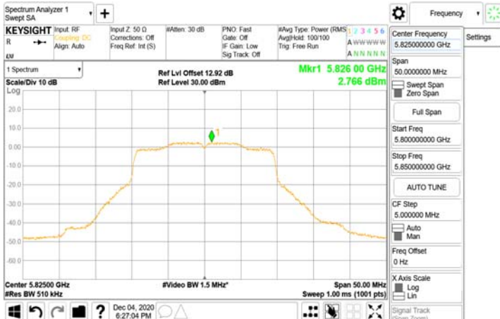
802.11ax_20MHz_Chian0_5825MHz-5825
