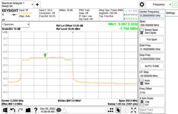
802.11ax_160MHz_Chian1_5250MHz -996-S67
