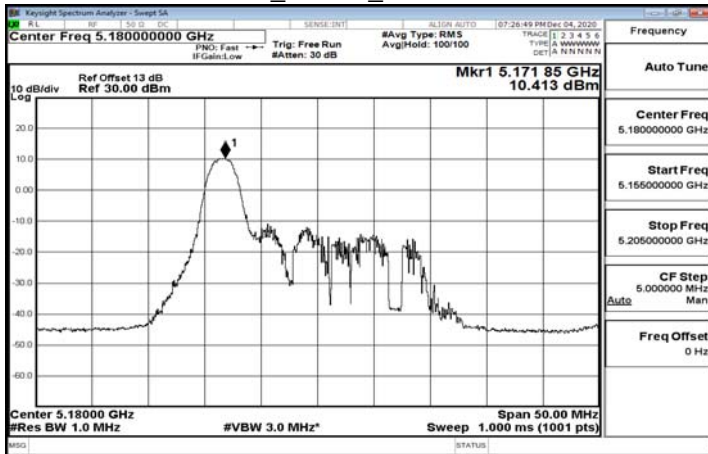
802.11ax_20MHz_5180MHz-52-37
