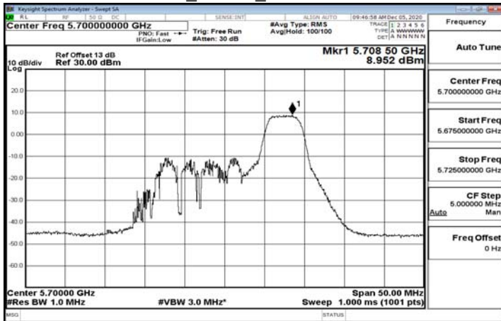
802.11ax_20MHz_5720MHz_UNII 2C
