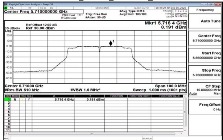
802.11n_40MHz_5710MHz_UNII 3
