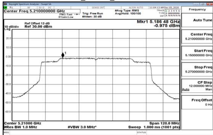
802.11ax_80MHz_5210MHz-484-65
