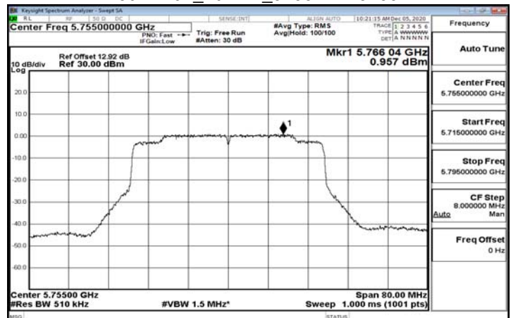
802.11ax_40MHz_5755MHz-242-61
