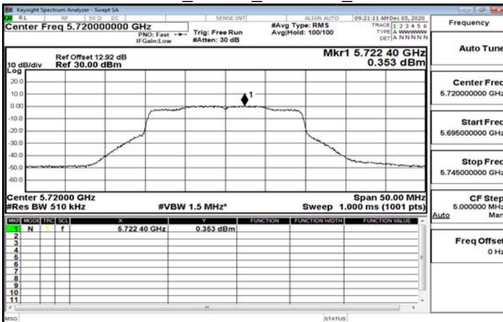
802.11ax_20MHz_5720MHz_UNII 3
