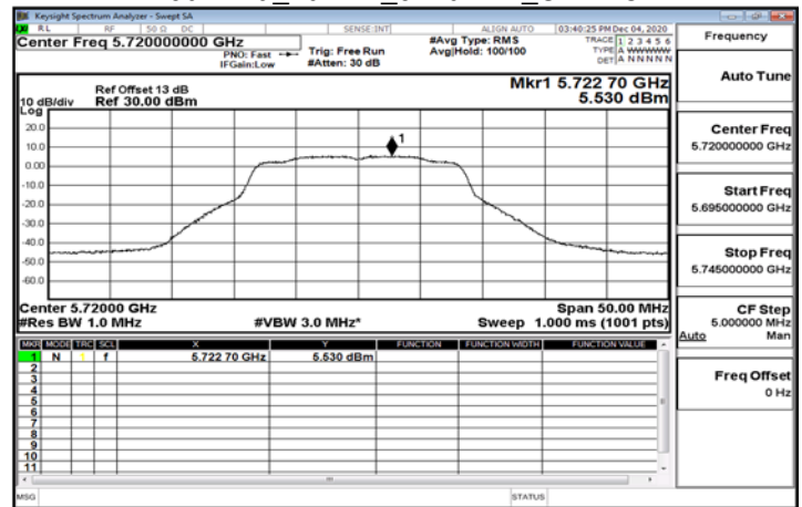
802.11a_20MHz_5720MHz_UNII 3
