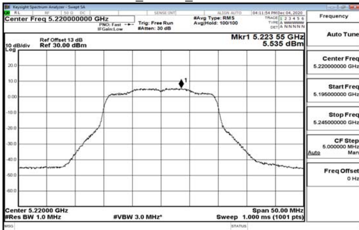
802.11ax_20MHz_5220MHz-5220
