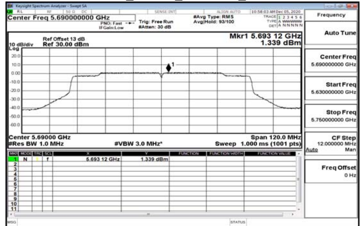
802.11ac_80MHz_5690MHz_UNII 3
