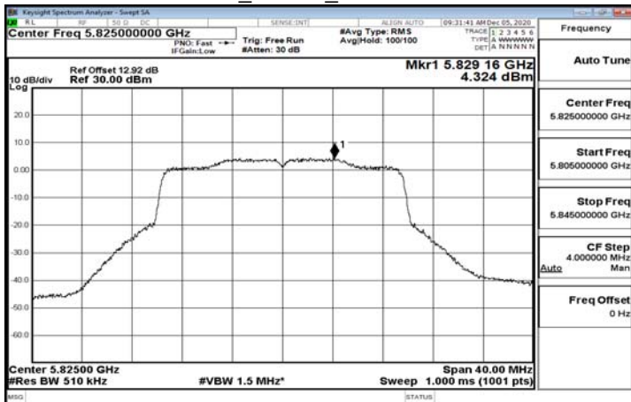
802.11ax_20MHz_5825MHz-5825
