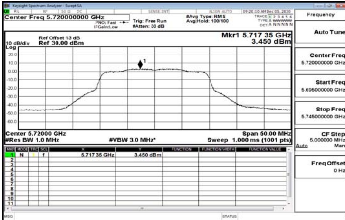
802.11ax_20MHz_5720MHz_UNII 3
