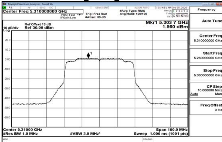
802.11ax_40MHz_5310MHz-242-62
