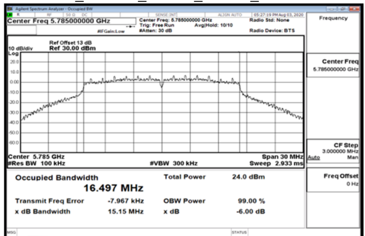
FCC_802.11a_20MHz_Chain1_5785MHz
