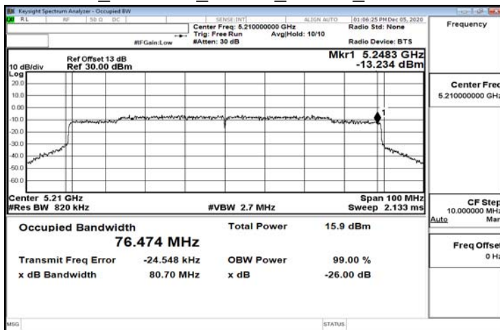
FCC_802.11ax_80MHz_Chain0_5210MHz
