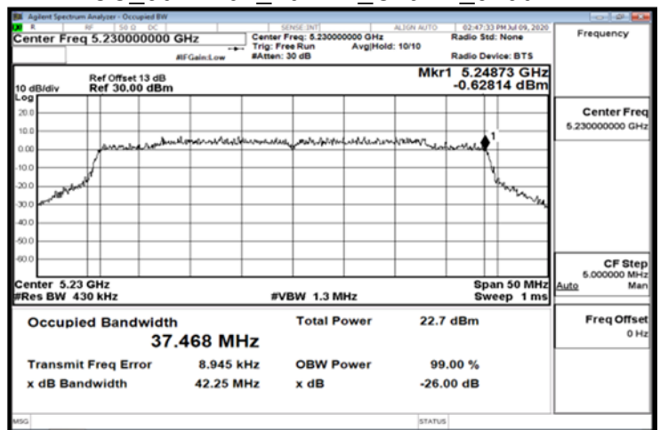
FCC_802.11ax_40MHz_Chain1_5230MHz
