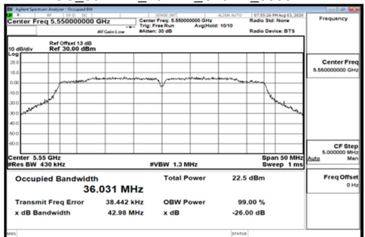
FCC_802.11n_40MHz_Chain1_5550MHz
