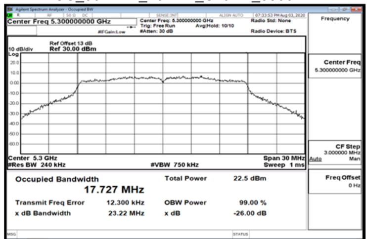
FCC_802.11n_20MHz_Chain1_5300MHz
