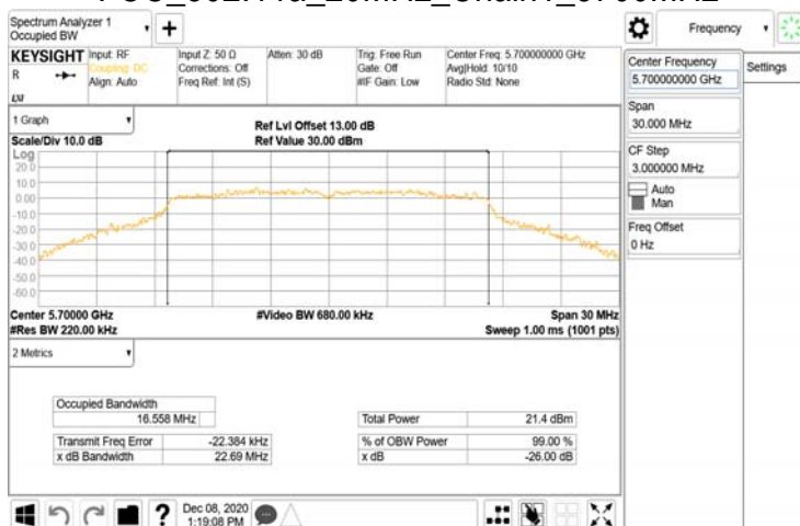
FCC_802.11a_20MHz_Chain1_5700MHz
