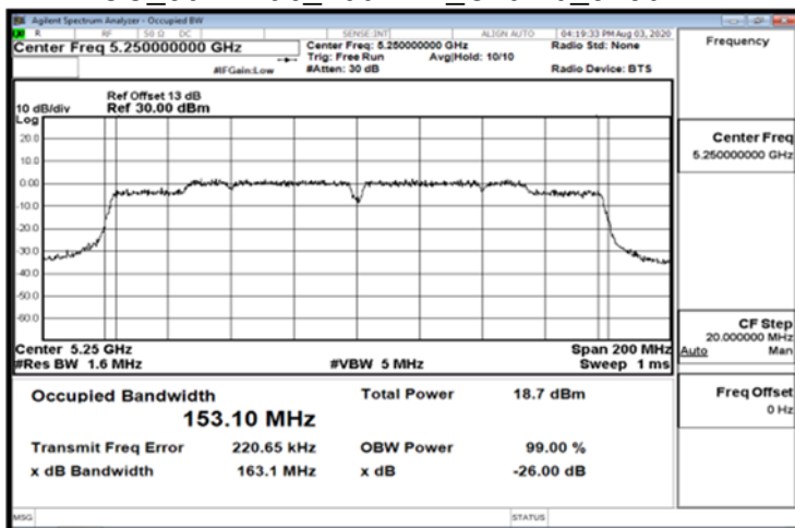
FCC_802.11ac_160MHz_Chain0_5250MHz
