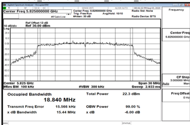
FCC_802.11ax_20MHz_Chain1_5825MHz
