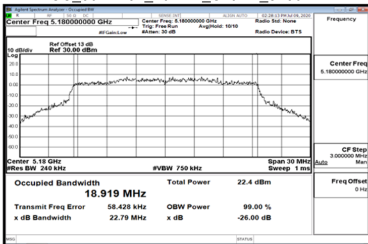
FCC_802.11ax_20MHz_Chain1_5180MHz
