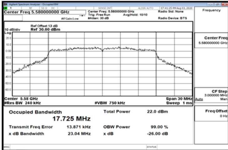
FCC_802.11n_20MHz_Chain1_5580MHz
