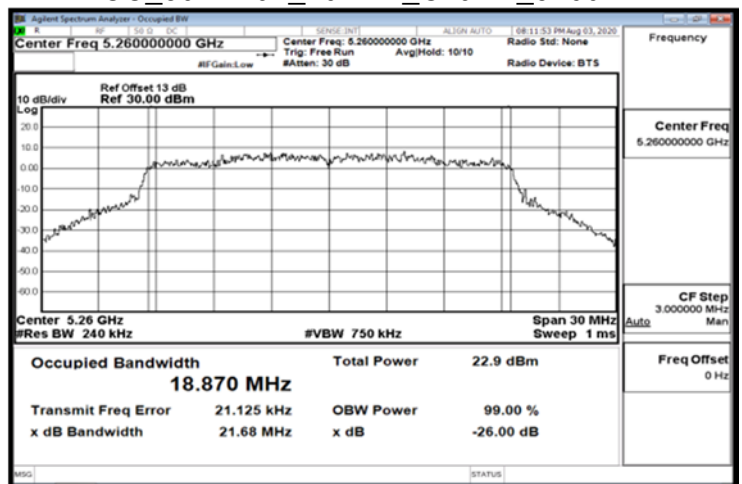
FCC_802.11ax_20MHz_Chain1_5260MHz
