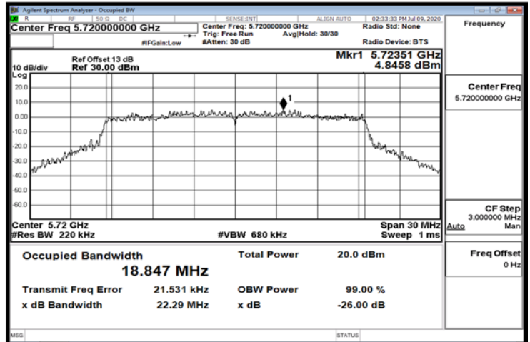
FCC_802.11ax_20MHz_Chain1_5720MHz
