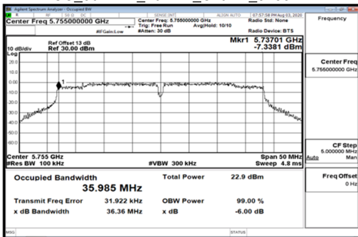
FCC_802.11n_40MHz_Chain1_5755MHz
