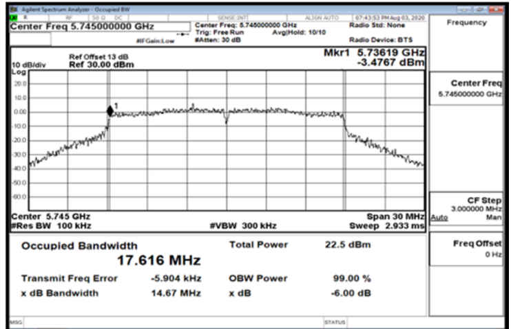
FCC_802.11n_20MHz_Chain1_5745MHz
