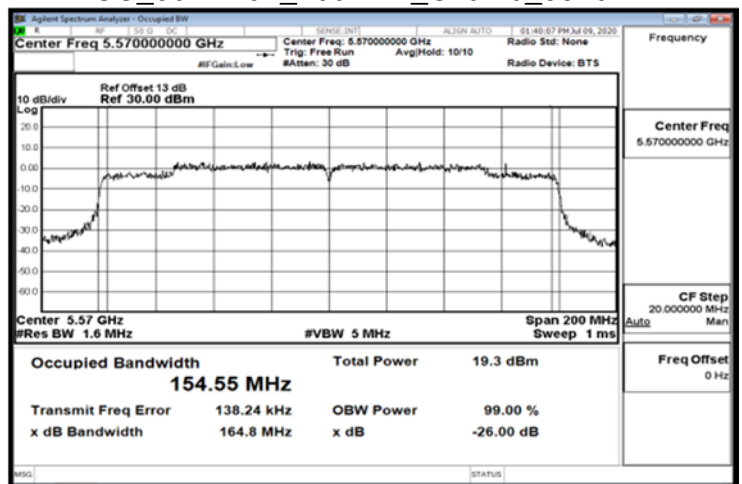
FCC_802.11ax_160MHz_Chain0_5570MHz
