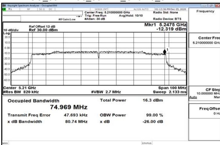
FCC_802.11ac_80MHz_Chain0_5210MHz
