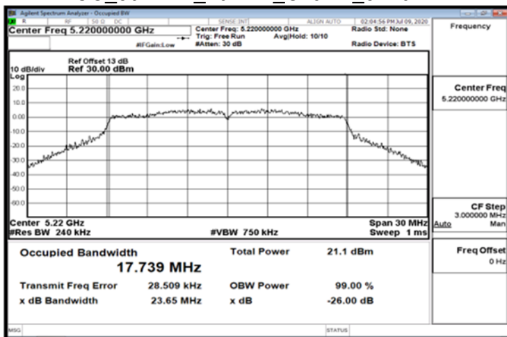
FCC_802.11n_20MHz_Chain1_5220MHz
