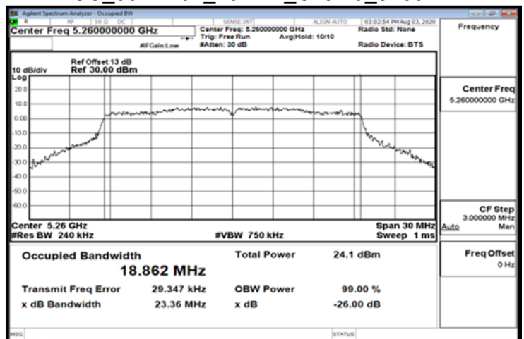
FCC_802.11ax_20MHz_Chain0_5260MHz
