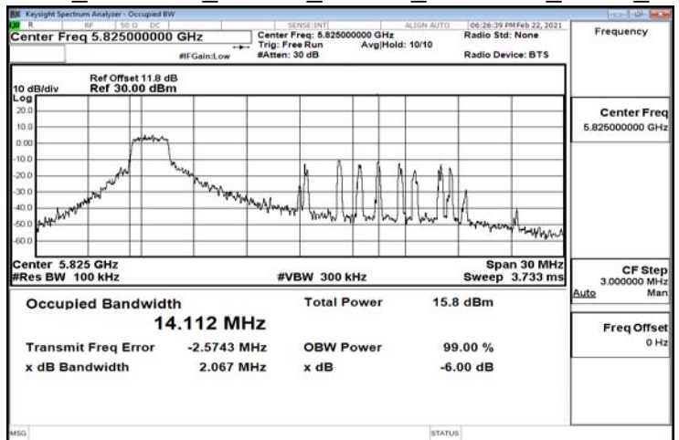
FCC_802.11ax_20MHz_Chain0_5825MHz_RU26_0
