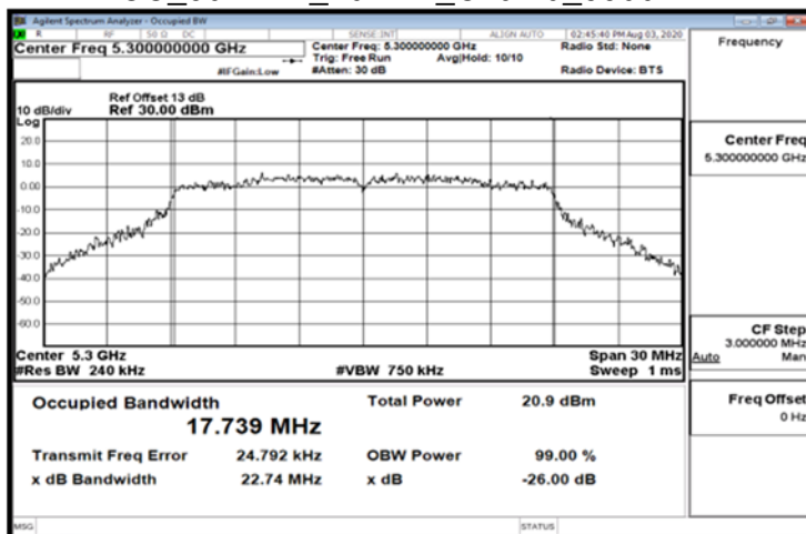
FCC_802.11n_20MHz_Chain0_5300MHz
