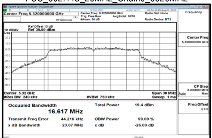
FCC_802.11a_20MHz_Chain0_5320MHz
