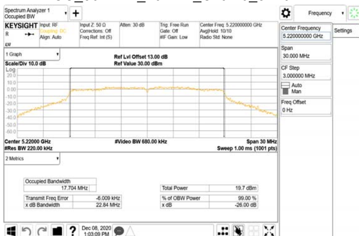
FCC_802.11n_20MHz_Chain0_5220MHz
