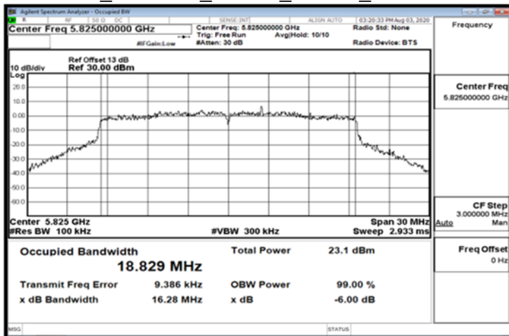
FCC_802.11ax_20MHz_Chain0_5825MHz
