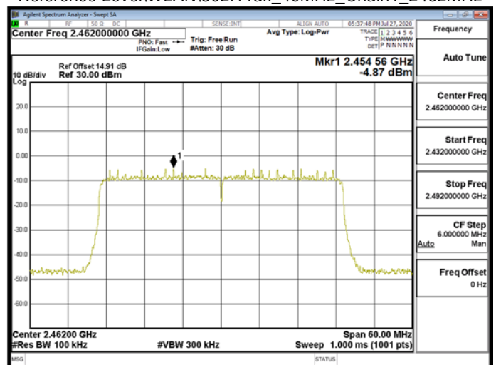
Reference Level\WLAN\802.11ax_40MHz_Chain1_2462MHz
