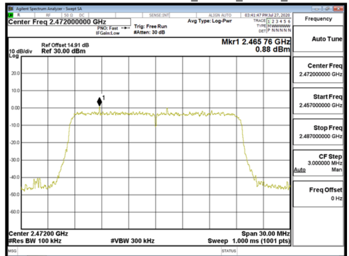
Reference Level\WLAN\802.11ax_20MHz_Chain1_2472MHz
