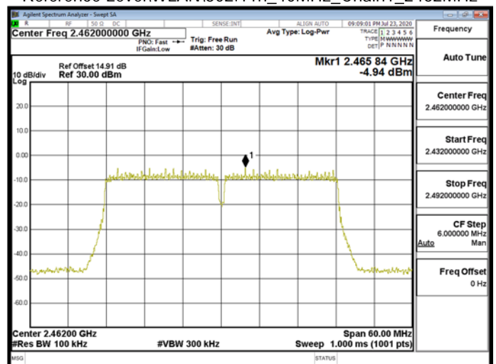
Reference Level\WLAN\802.11n_40MHz_Chain1_2462MHz
