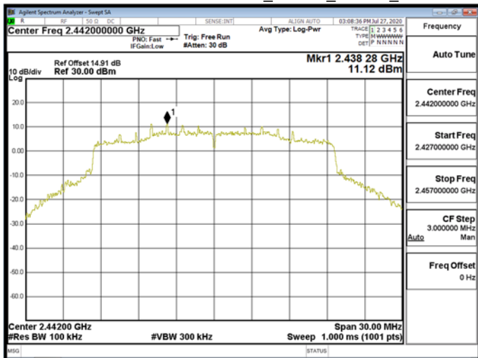
Reference Level\WLAN\802.11ax_20MHz_Chain1_2442MHz
