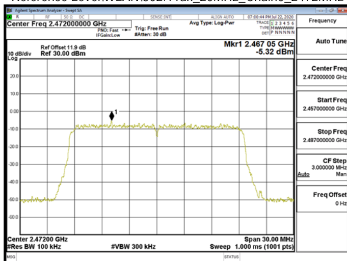
Reference Level\WLAN\802.11ax_20MHz_Chain0_2472MHz
