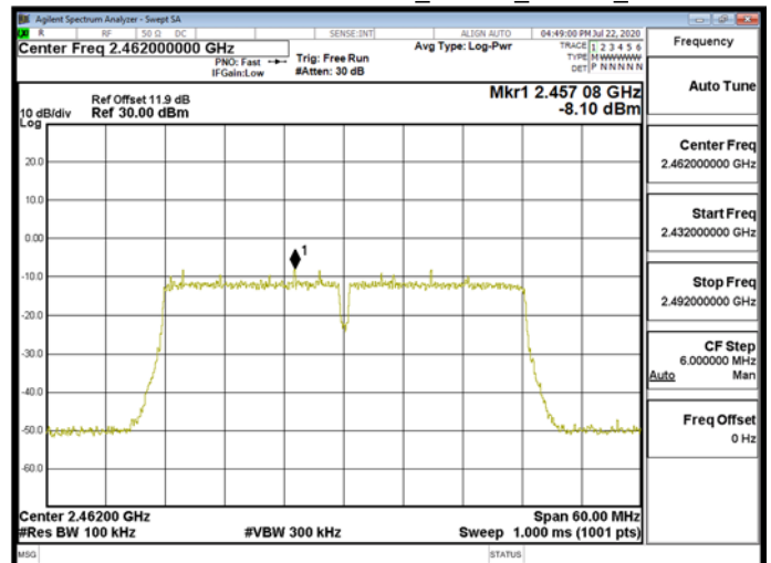
Reference Level\WLAN\802.11n_40MHz_Chain0_2462MHz
