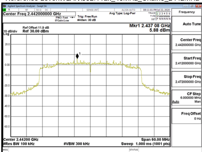
Reference Level\WLAN\802.11ax_40MHz_Chain0_2442MHz
