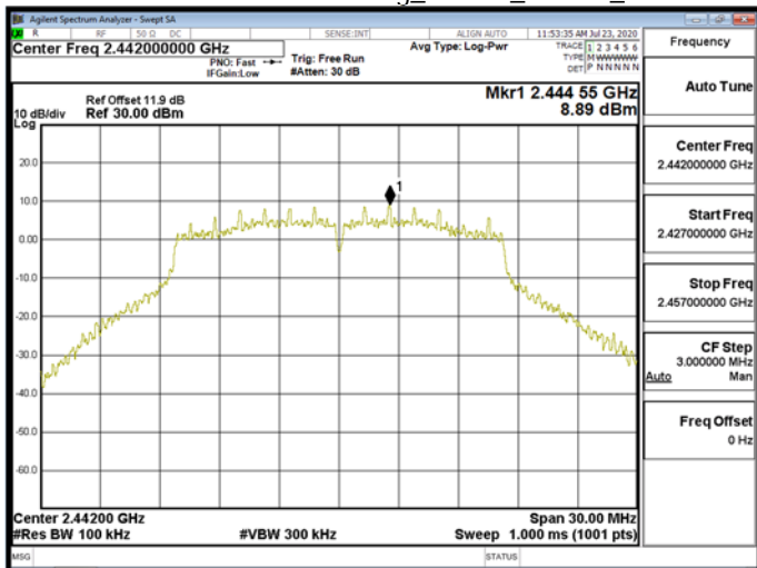
Reference Level\WLAN\802.11g_20MHz_Chain1_2442MHz
