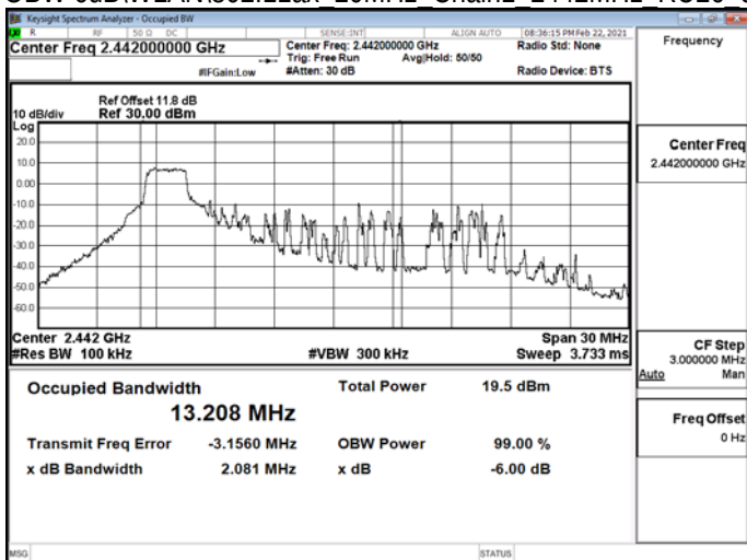
OBW 6dB\WLAN\802.11ax 20MHz Chain1 2442MHz RU26 0
