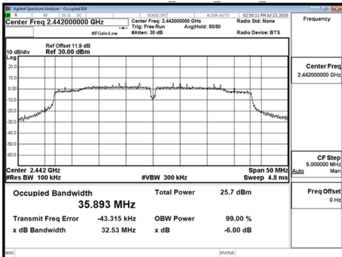
OBW 6dB\WLAN\802.11n_40MHz_Chain1_2442MHz
