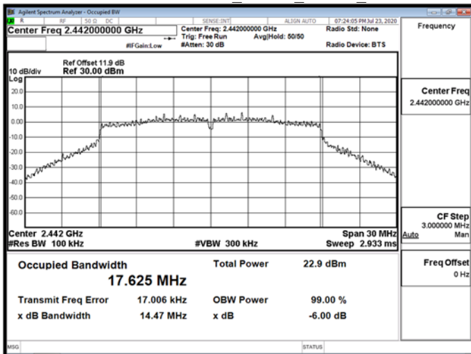
OBW 6dB\WLAN\802.11n_20MHz_Chain1_2442MHz
