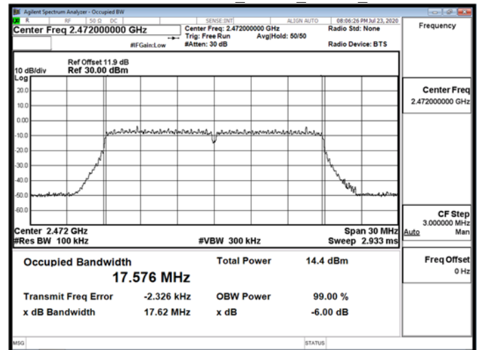
OBW 6dB\WLAN\802.11n_20MHz_Chain1_2472MHz
