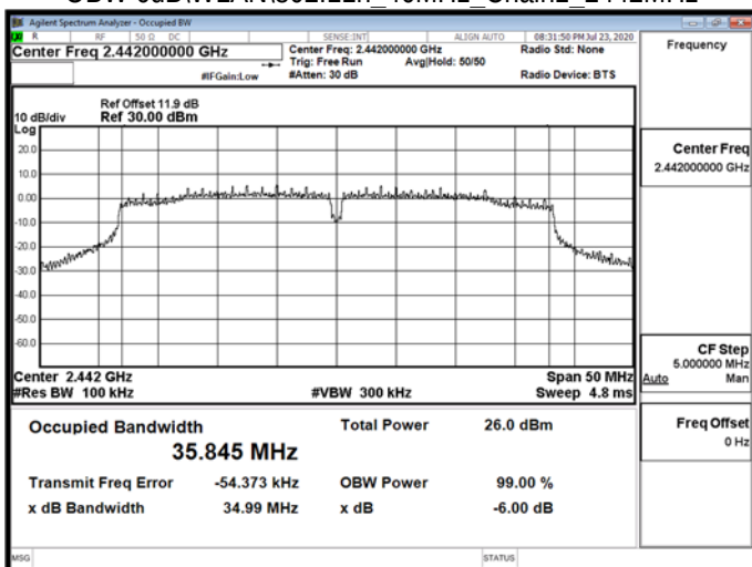
OBW 6dBI\WLAN\802.11n_40MHz_Chain1_2442MHz
