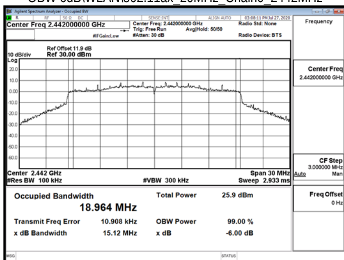
OBW 6dBWLAN\802.11ax_20MHz_Chain0_2442MHz
