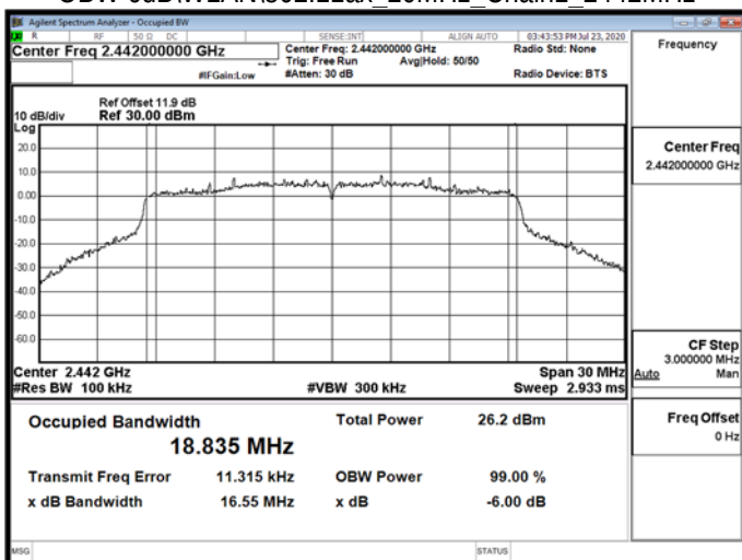
OBW 6dBWLAN\802.11ax_20MHz_Chain1_2442MHz
