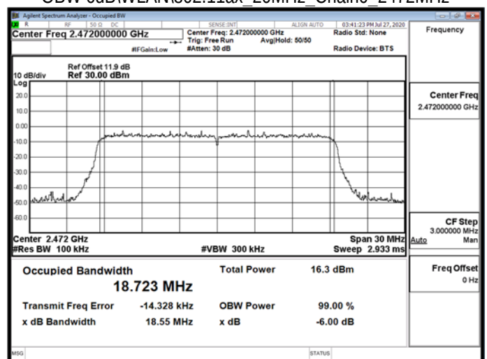
OBW 6dBWLAN\802.11ax_20MHz_Chain0_2472MHz
