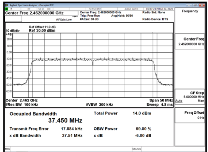
OBW 6dBWLAN\802.11ax_40MHz_Chain0_2462MHz
