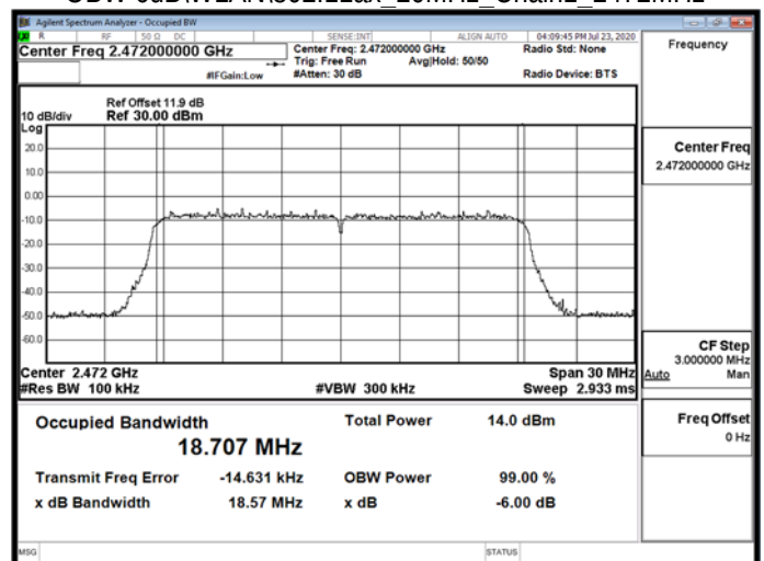
OBW 6dBWLAN\802.11ax_20MHz_Chain1_2472MHz
