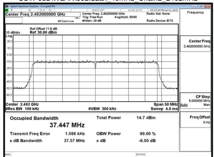
OBW 6dBWLAN\802.11ax_40MHz_Chain1_2462MHz
