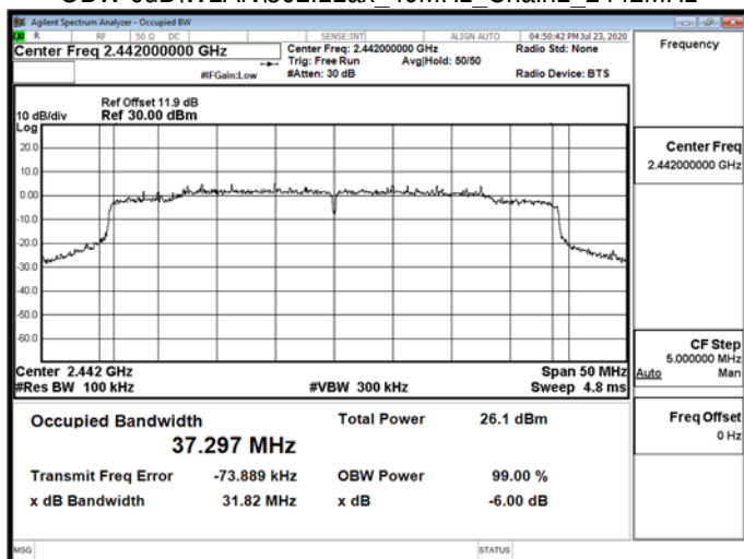
OBW 6dBWLAN\802.11ax_40MHz_Chain1_2442MHz
