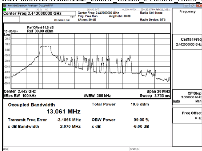
OBW 6dB\WLAN\802.11ax 20MHz Chain0 2442MHz RU26 0
