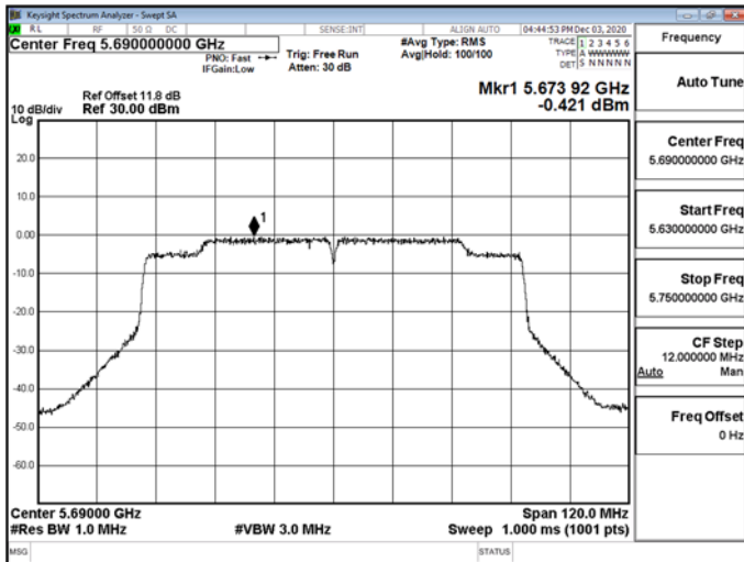
802.11ac_80MHz_CH1_5690MHz_UNII 3
