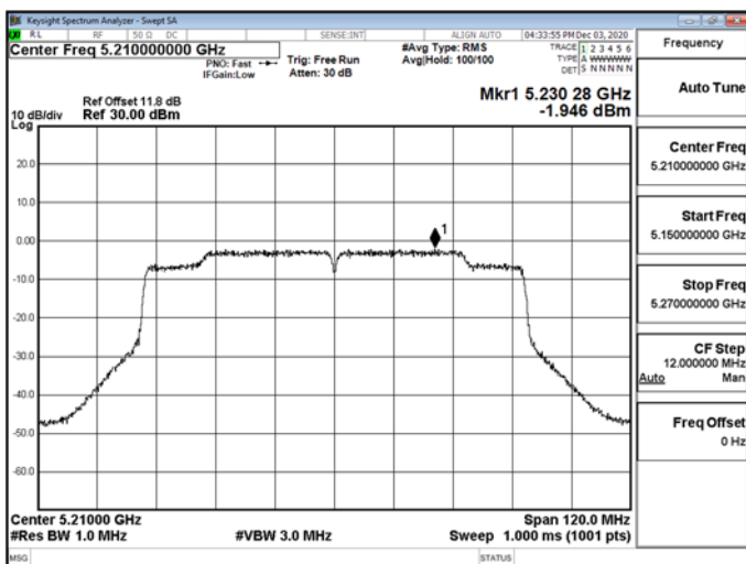
802.11ac_80MHz_CH1_5210MHz-5210
