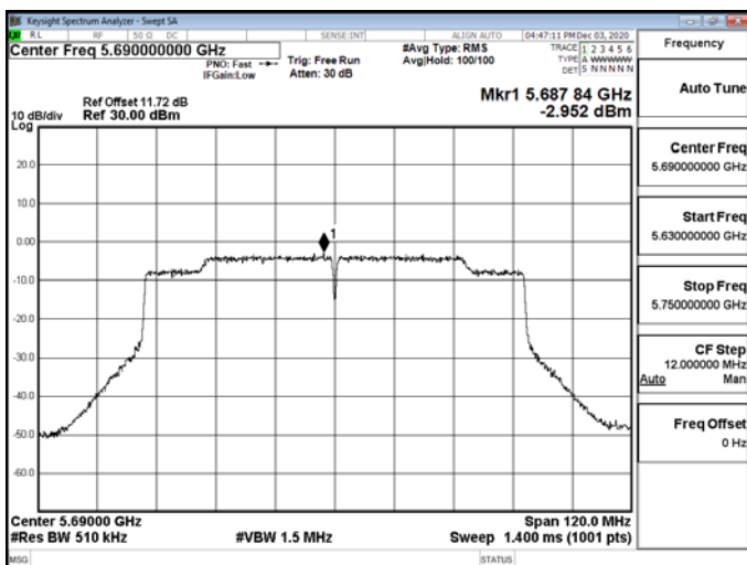
802.11ac_80MHz_CH0_5690MHz_UNII 3
