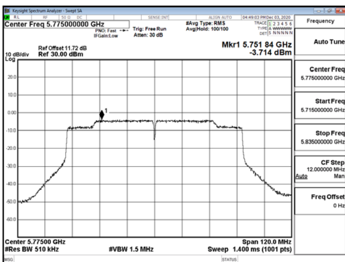
802.11ac_80MHz_CH1_5775MHz-5775
