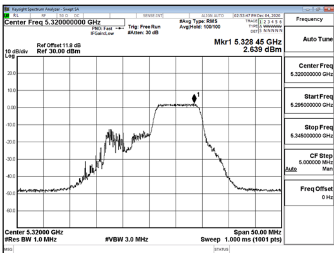
802.11ax_20MHz_RU_106_54_CH1_5320MHz-5320
