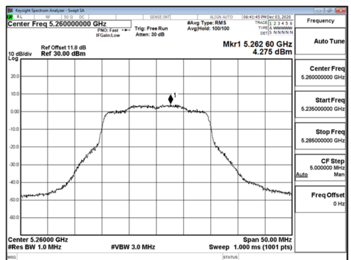
802.11ax_20MHz_CH1_5260MHz-5260
