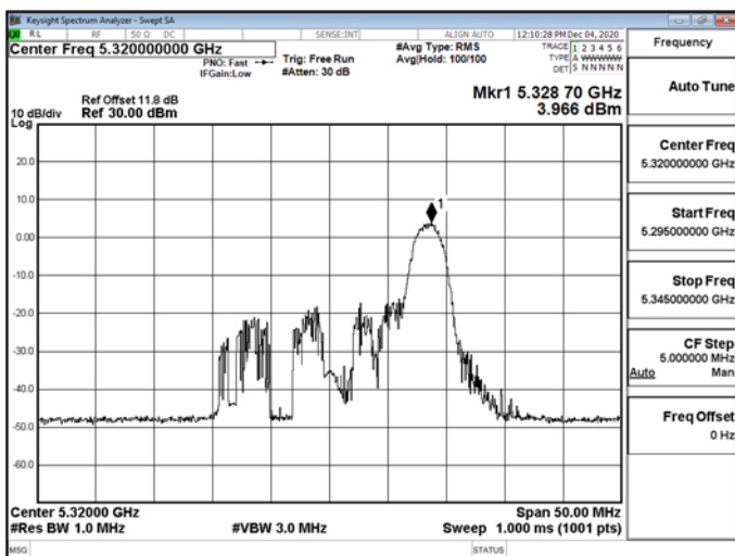
802.11ax_20MHz_RU_26_8_CH0_5320MHz-5320
