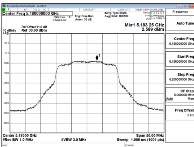
802.11ax_20MHz_CH1_5180MHz-5180
