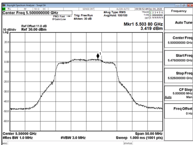
802.11ax_20MHz_CH1_5500MHz-5500
