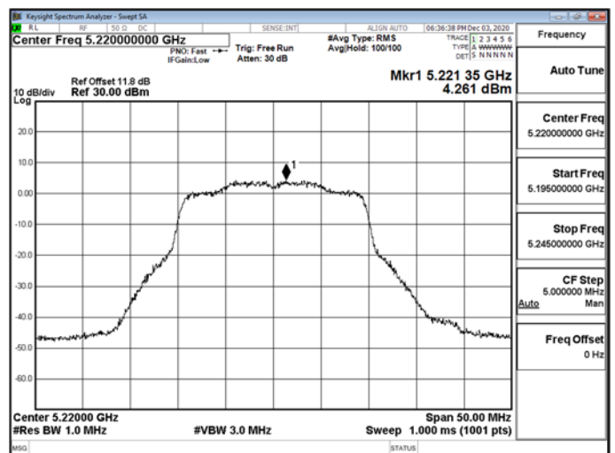
802.11ax_20MHz_CH0_5220MHz-5220
