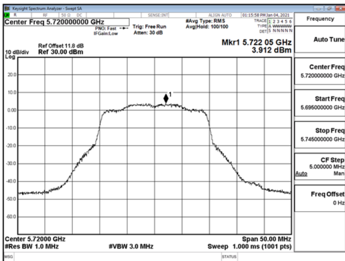
802.11ax_20MHz_CHO_5720MHz_UNII 3
