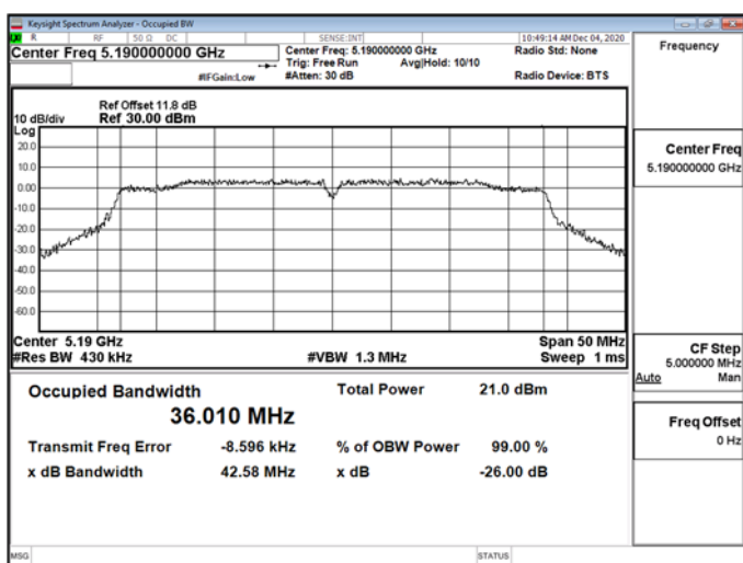
802.11n_40MHz_Chain1_5190MHz
