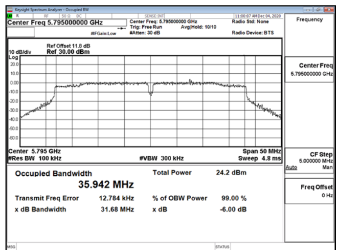
802.11n_40MHz_Chain1_5795MHz
