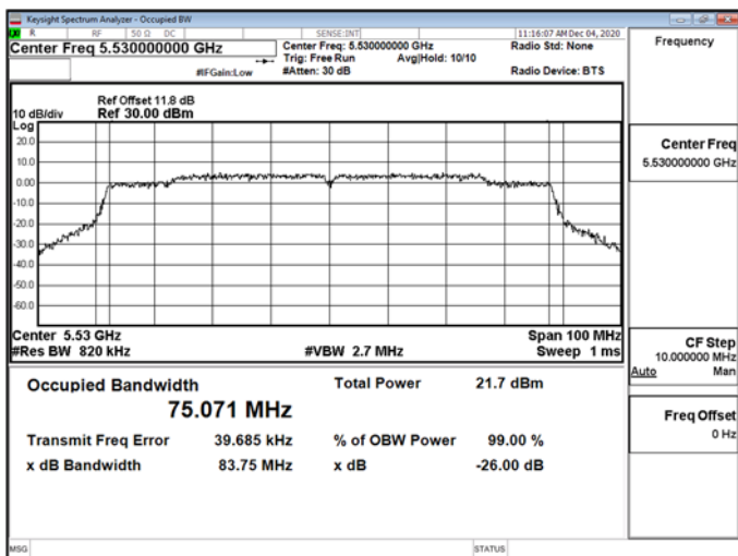
802.11ac_80MHz_Chain1_5530MHz
