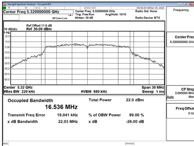
802.11a_20MHz_Chain1_5320MHz
