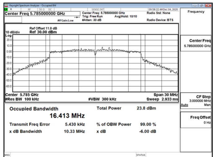
802.11a_20MHz_Chain1_5785MHz
