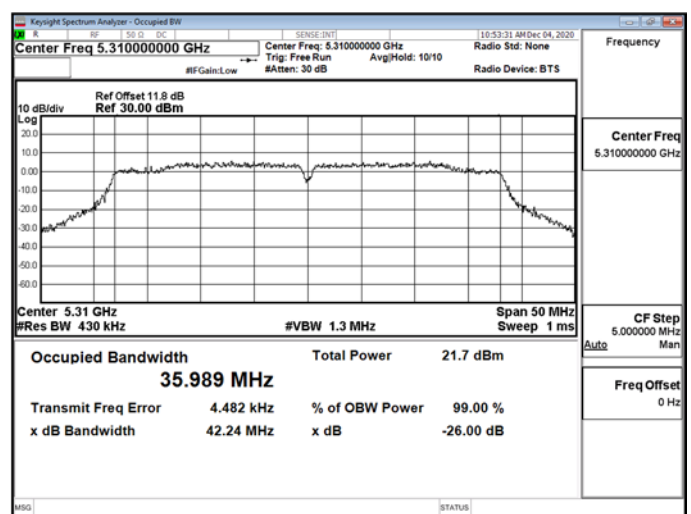
802.11n_40MHz_Chain1_5310MHz
