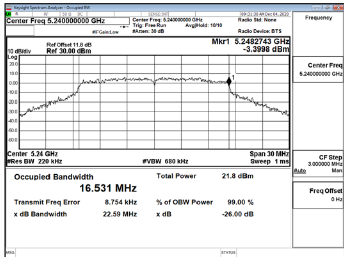
802.11a_20MHz_Chain1_5240MHz
