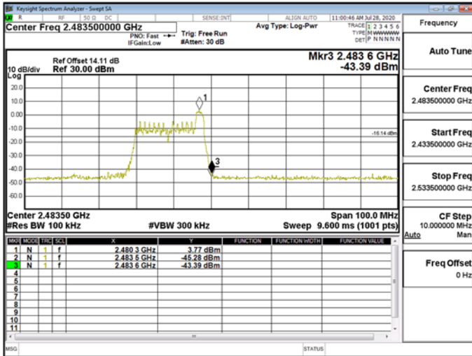
Band Edge\WLAN\802.11ax_20MHz_Chain1_2472MHz_RU52_40
