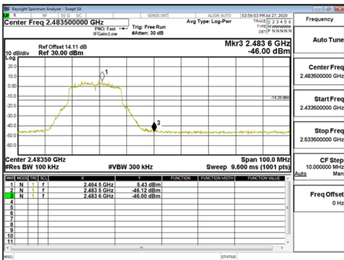
Band Edge\WLAN\802.11ax_20MHz_Chain1_2462MHz
