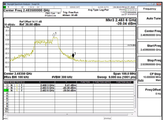
Band Edge\WLAN\802.11ax_20MHz_Chain1_2462MHz_RU52_40
