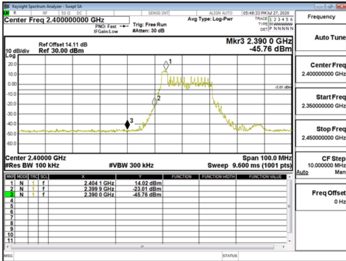
Band Edge\WLAN\802.11ax_20MHz_Chain1_2412MHz_RU52_37
