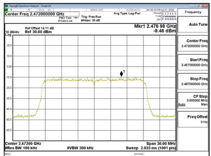
Reference Level\WLAN\802.11ax_20MHz_Chain1_2472MHz
