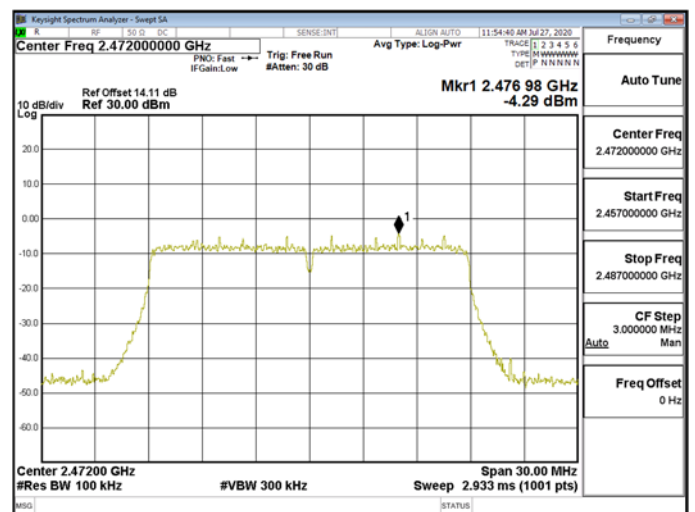
Reference Level\WLAN\802.11n_20MHz_Chain1_2472MHz
