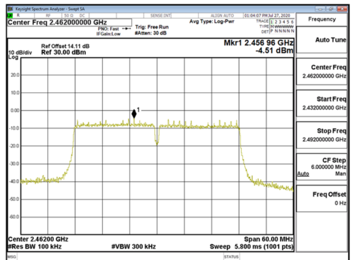
Reference Level\WLAN\802.11n_40MHz_Chain1_2462MHz
