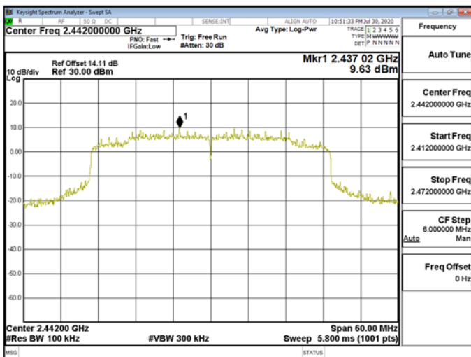
Reference Level\WLAN\802.11ax_40MHz_Chain1_2442MHz
