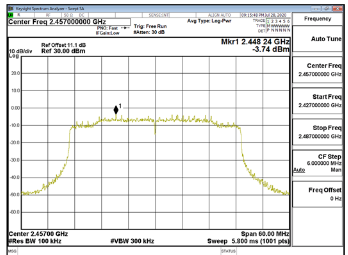
Reference Level\WLAN\802.11ax_40MHz_Chain0_2457MHz
