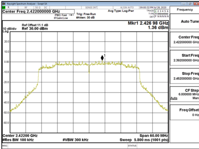
Reference Level\WLAN\802.11ax_40MHz_Chain0_2422MHz_RU242_61
