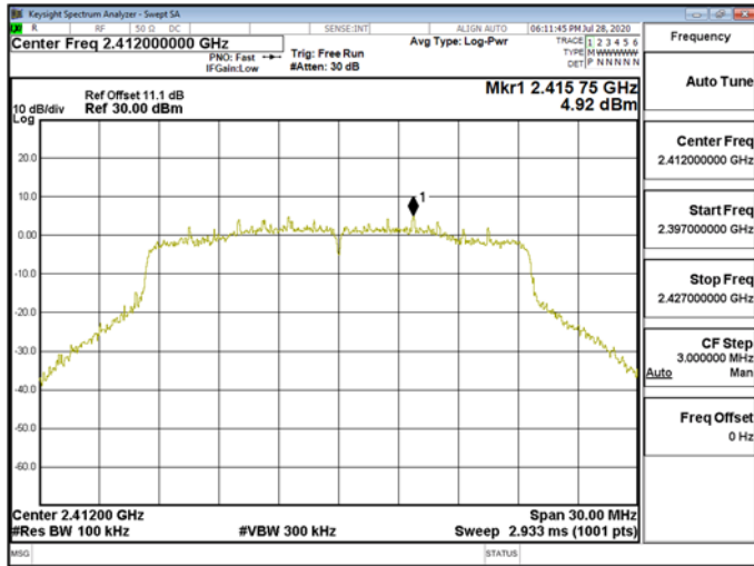
Reference Level\WLAN\802.11ax_20MHz_Chain0_2412MHz_RU106_53
