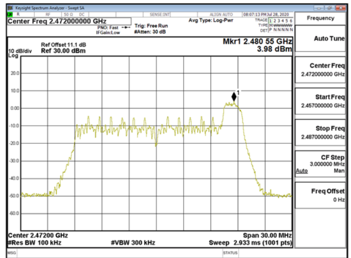
Reference Level\WLAN\802.11ax_20MHz_Chain0_2472MHz_RU26_8
