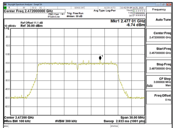
Reference Level\WLAN\802.11n_20MHz_Chain0_2472MHz
