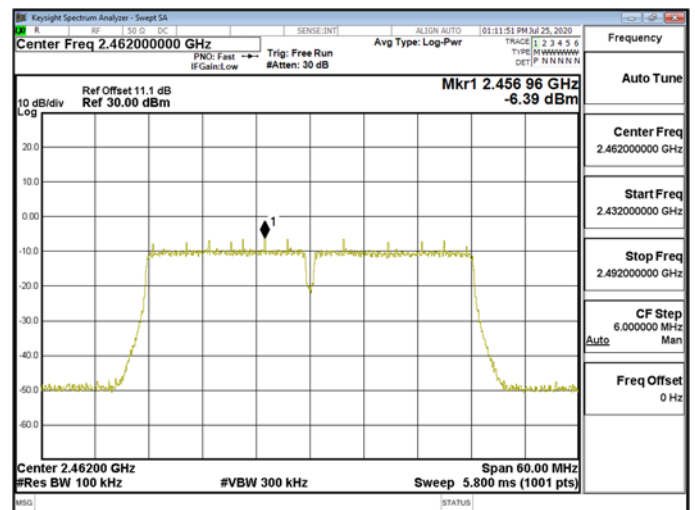
Reference Level\WLAN\802.11n_40MHz_Chain0_2462MHz
