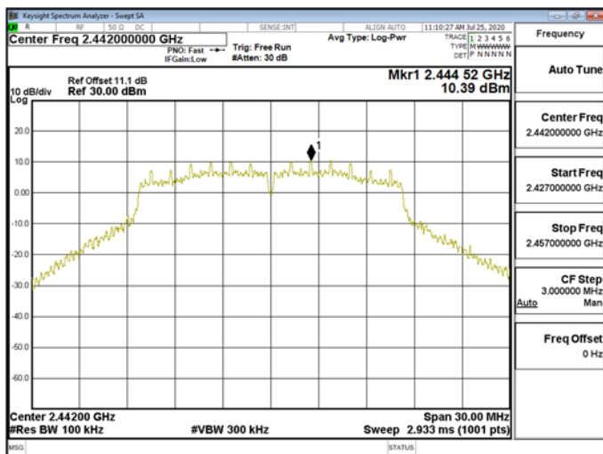
Reference Level\WLAN\802.11g_20MHz_Chain0_2442MHz
