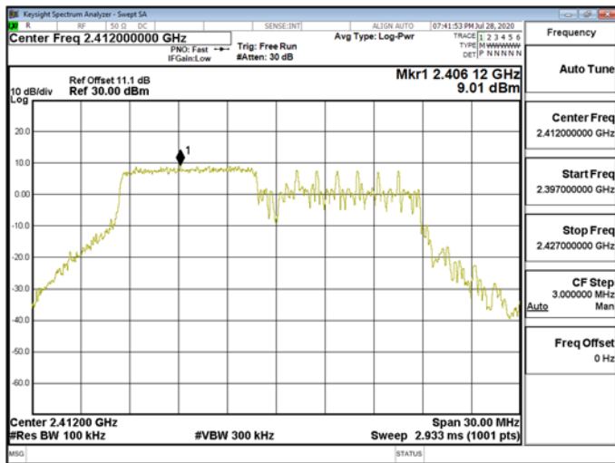
Reference Level\WLAN\802.11ax_20MHz_Chain0_2412MHz_RU26_0
