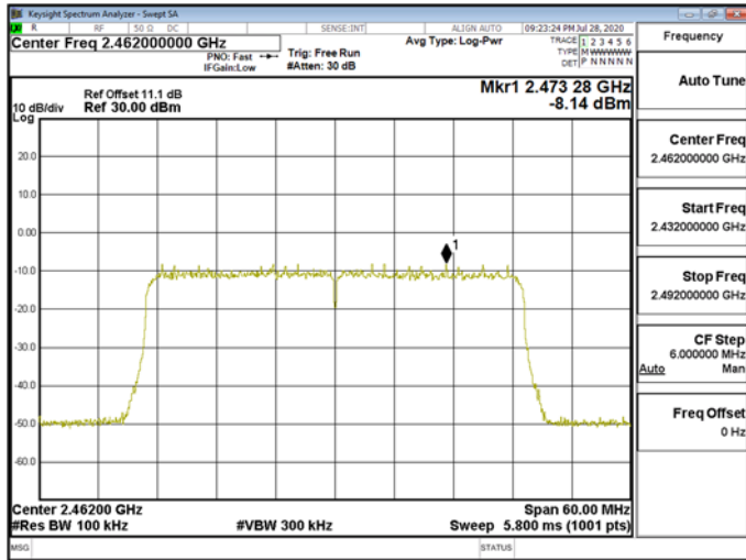
Reference Level\WLAN\802.11ax_40MHz_Chain0_2462MHz_RU242_62
