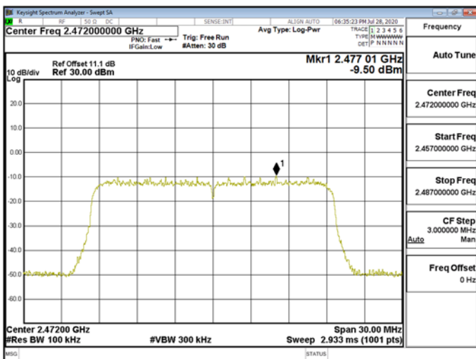
Reference Level\WLAN\802.11ax_20MHz_Chain0_2472MHz
