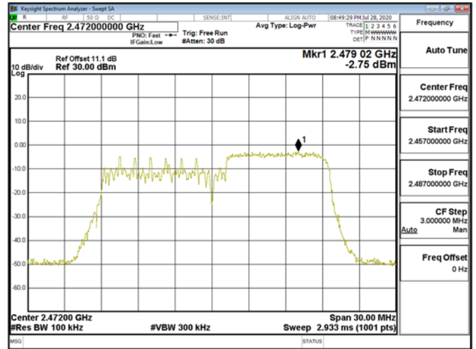
Reference Level\WLAN\802.11ax_20MHz_Chain0_2472MHz_RU26_8
