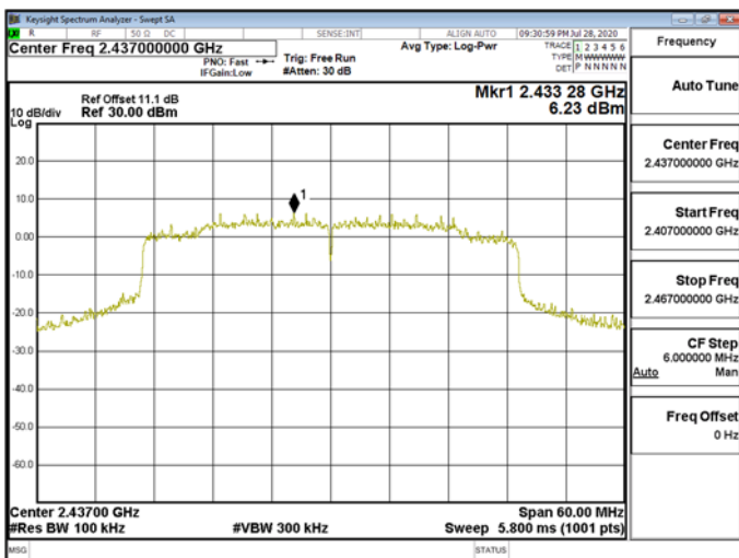
Reference Level\WLAN\802.11ax_40MHz_Chain0_2437MHz
