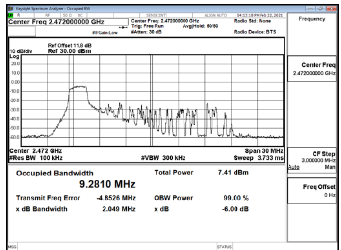
OBW 6dBWLAN\802.11ax_20MHz_Chain1_2472MHz_RU26_0
