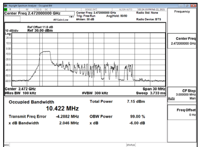
OBW 6dBWLAN\802.11ax_20MHz_Chain1_2472MHz_RU26_0
