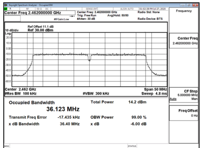
OBW 6dB\WLAN\802.11n_40MHz_Chain1_2462MHz
