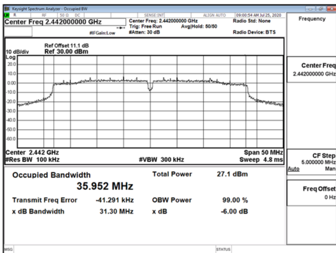
OBW 6dB\WLAN\802.11n_40MHz_Chain1_2442MHz
