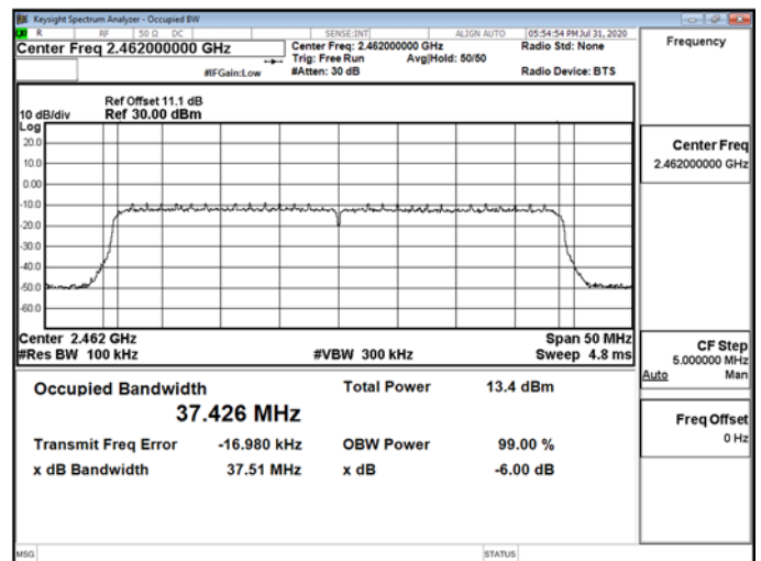
OBW 6dBWLAN802.11ax_40MHz_Chain0_2462MHz
