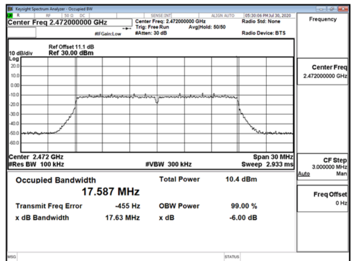
OBW 6dB\WLAN\802.11n_20MHz_Chain0_2472MHz
