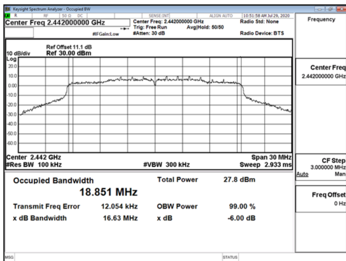
OBW 6dBWLAN802.11ax_20MHz_Chain1_2442MHz
