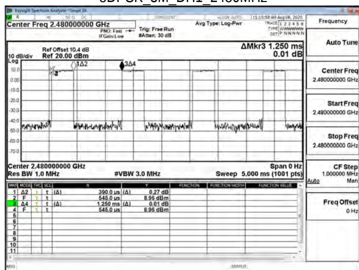
8DPSK 3M DH1 2480MHz
