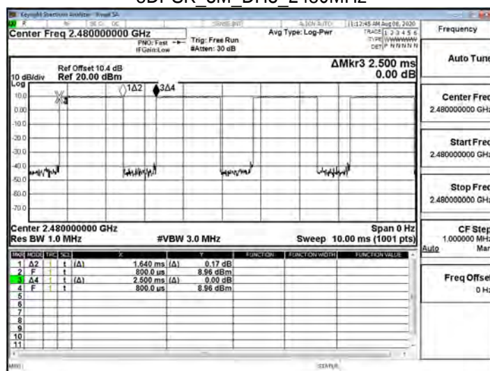
8DPSK 3M DH3 2480MHz
