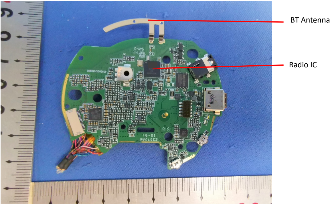
Right PCB
