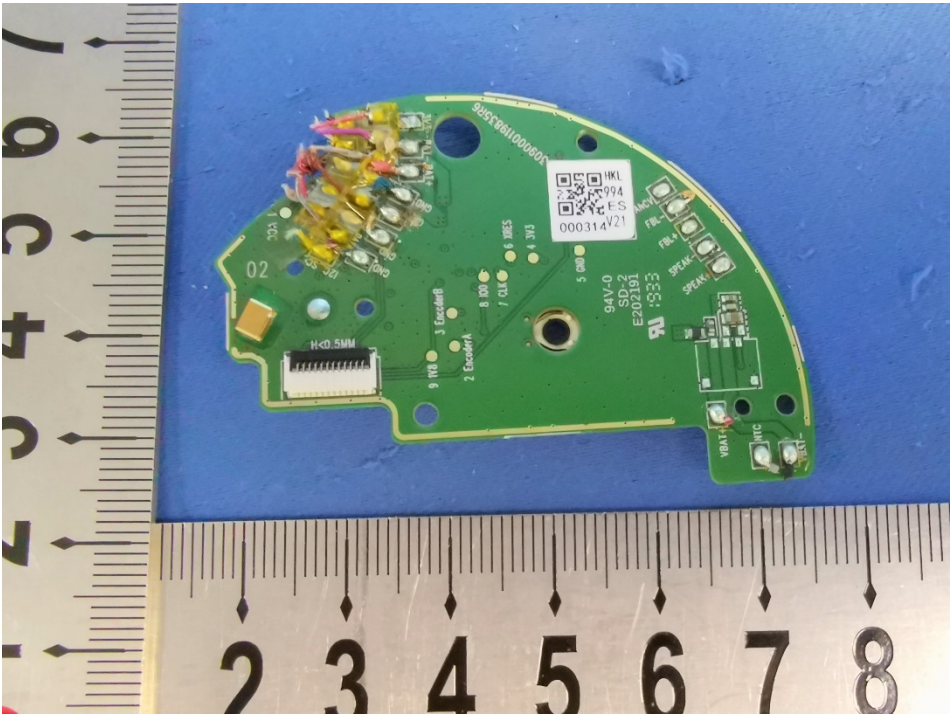
Left PCB
