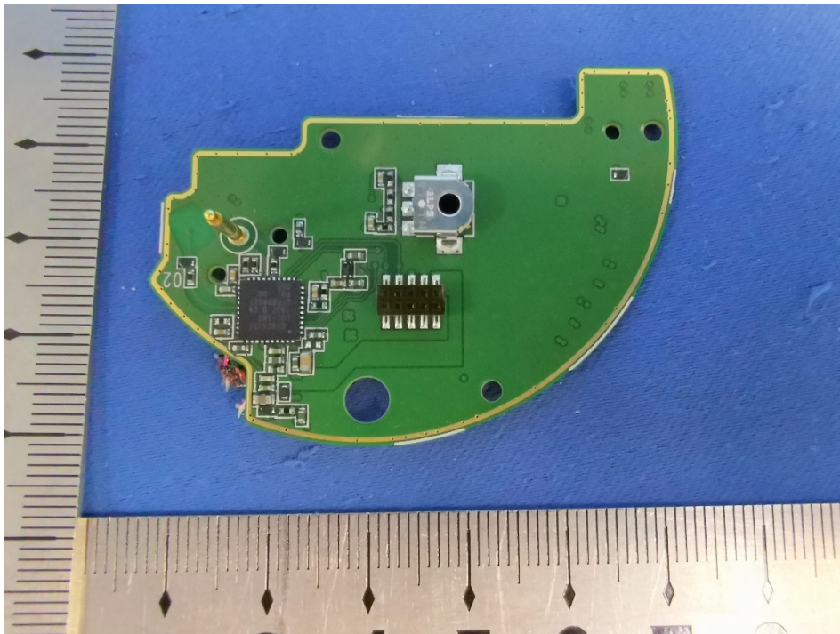
Left PCB – bottom side
