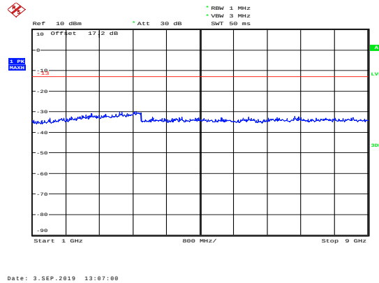
GSM 850 CH-Middle 1GHz ~ 9GHz
