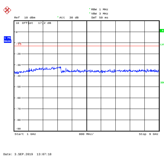
GSM 850 CH-Middle 1GHz ~ 9GHz
