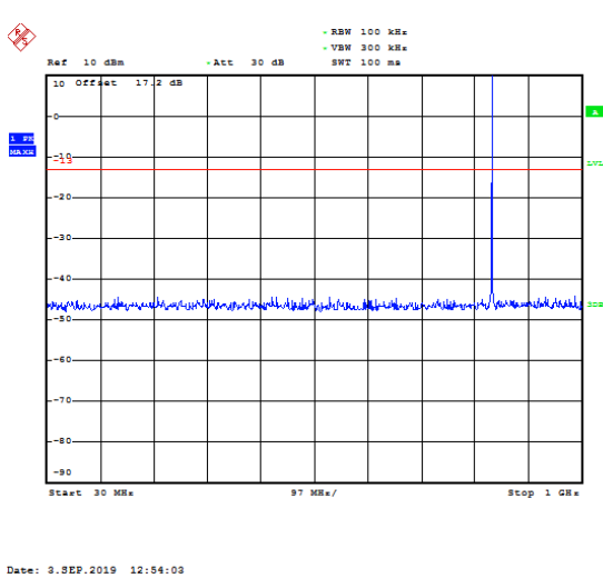
GSM 850 CH-Middle 30MHz ~ 1GHz
