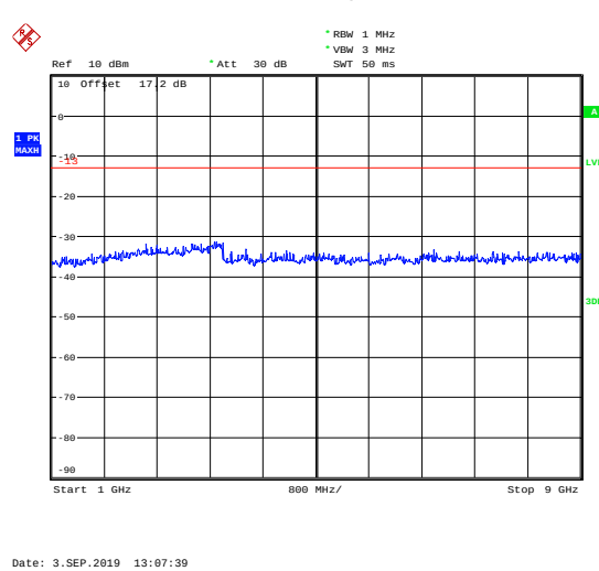
GSM 850 CH-High 1GHz ~ 9GHz
