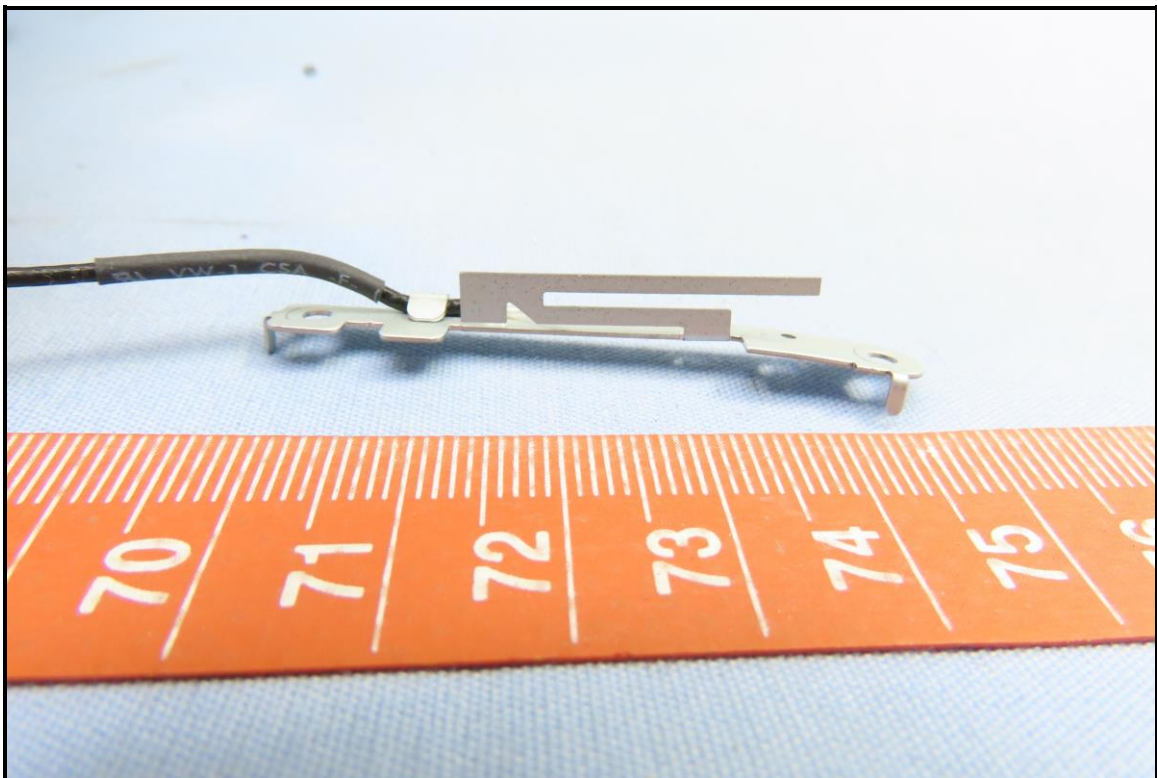
Wi-Fi/BT Antenna
