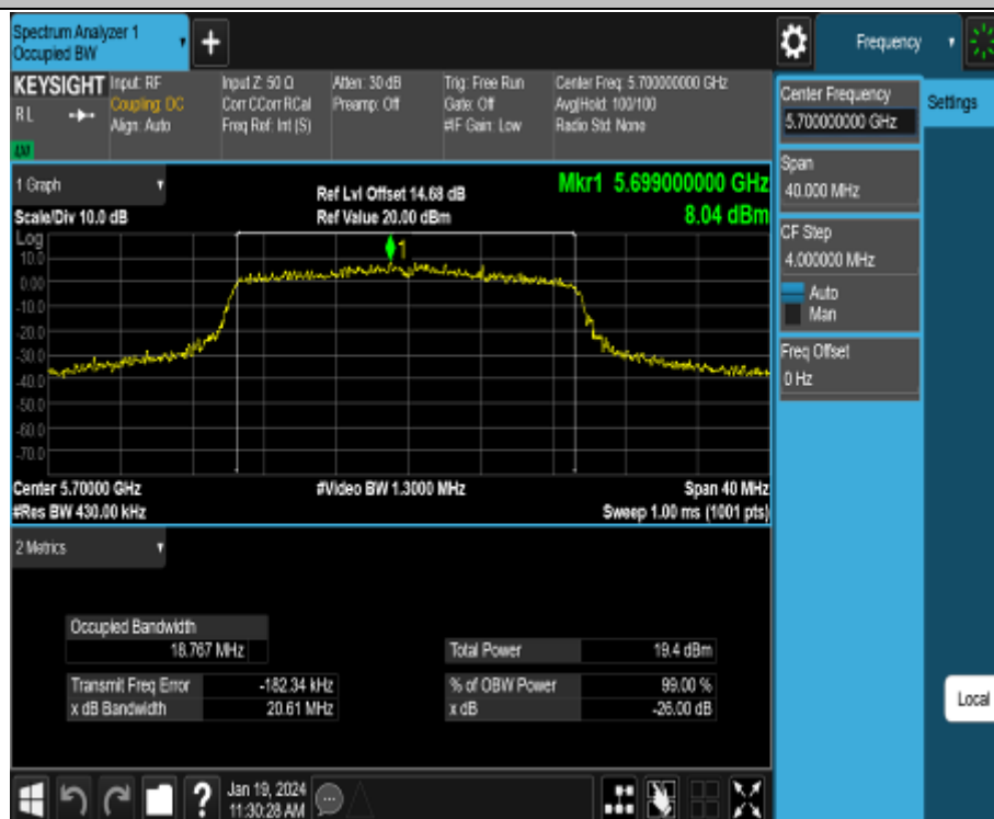
11AX20MIMO_Ant2_5700
