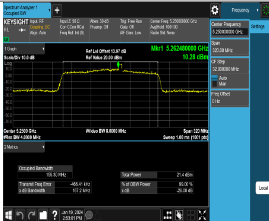
11AX160MIMO_Ant2_5250
