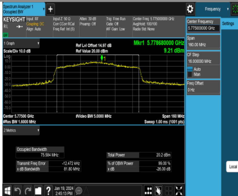
11AX80MIMO_Ant2_5775
