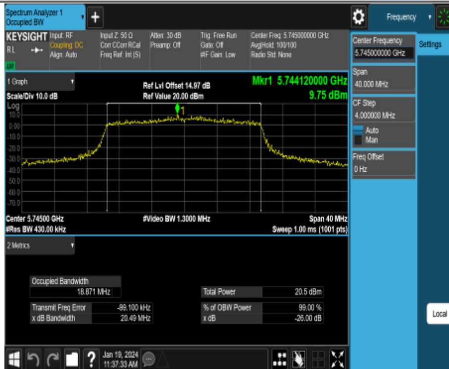
11AX20MIMO_Ant2_5745
