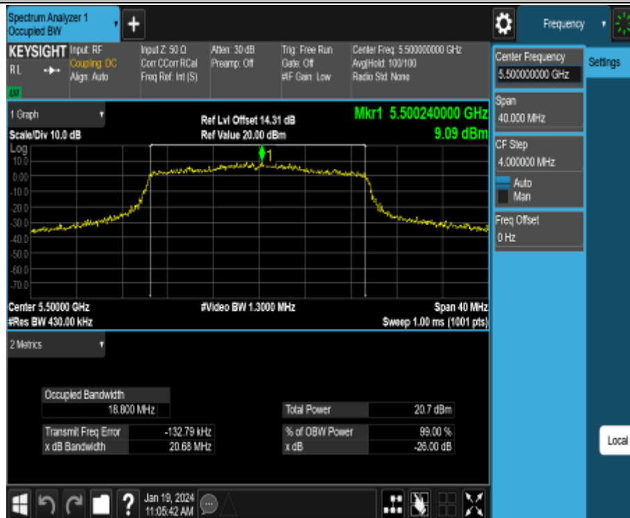
11AX20MIMO_Ant2_5500
