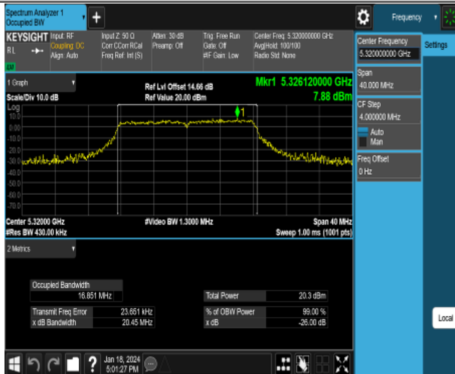
11N20MIMO_Ant2_5320
