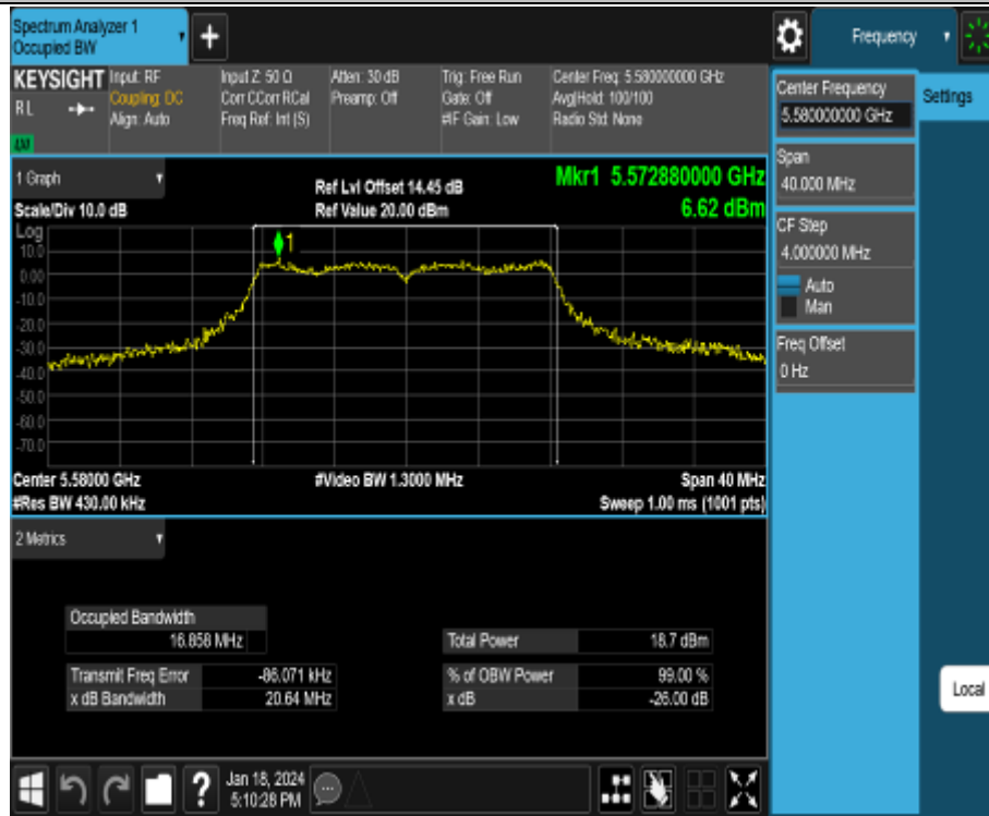
11N20MIMO_Ant2_5580
