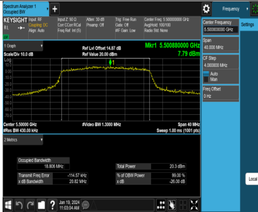
11AX20MIMO_Ant2_5500
