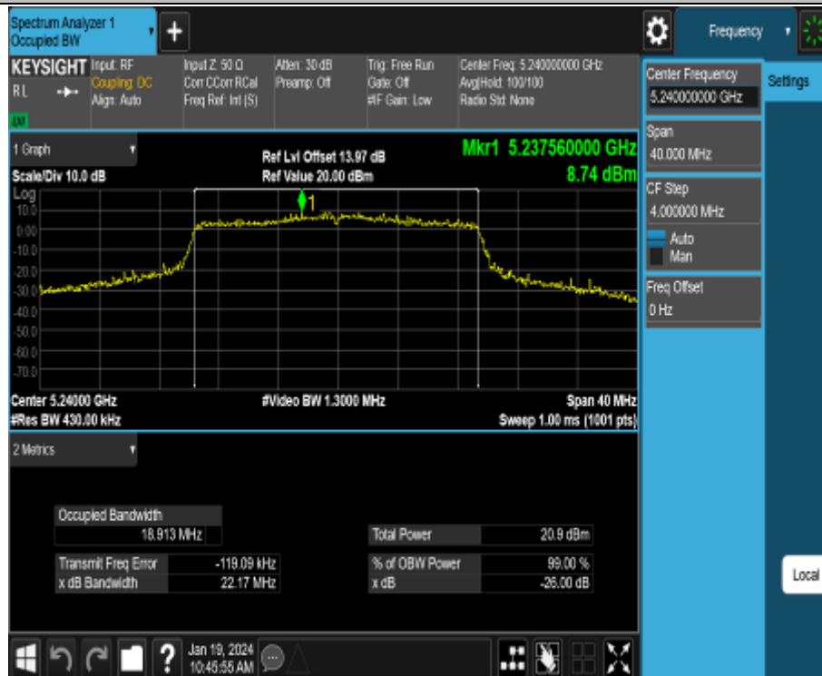
11AX20MIMO_Ant2_5240
