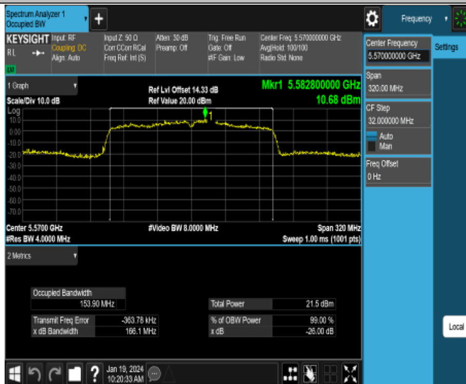
11AC160MIMO_Ant2_5570
