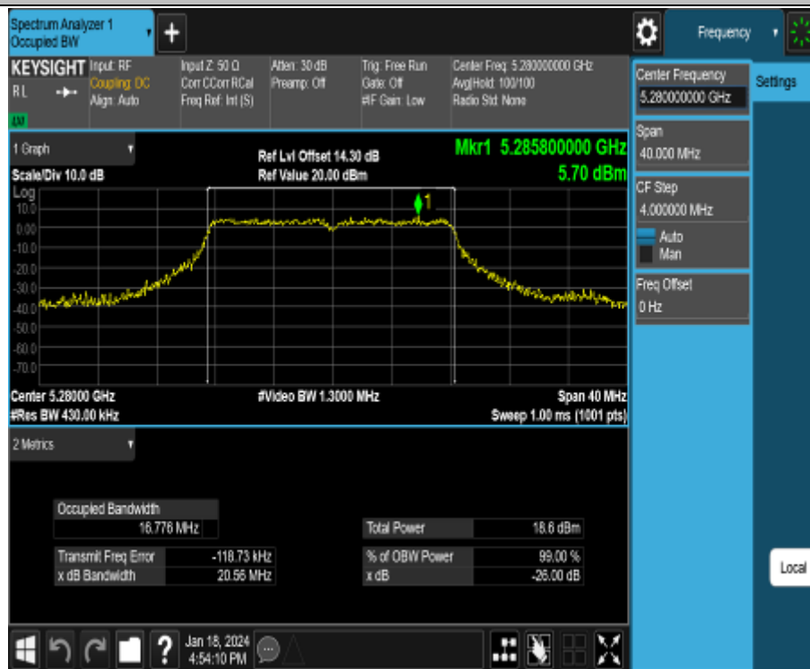
11N20MIMO_Ant2_5280
