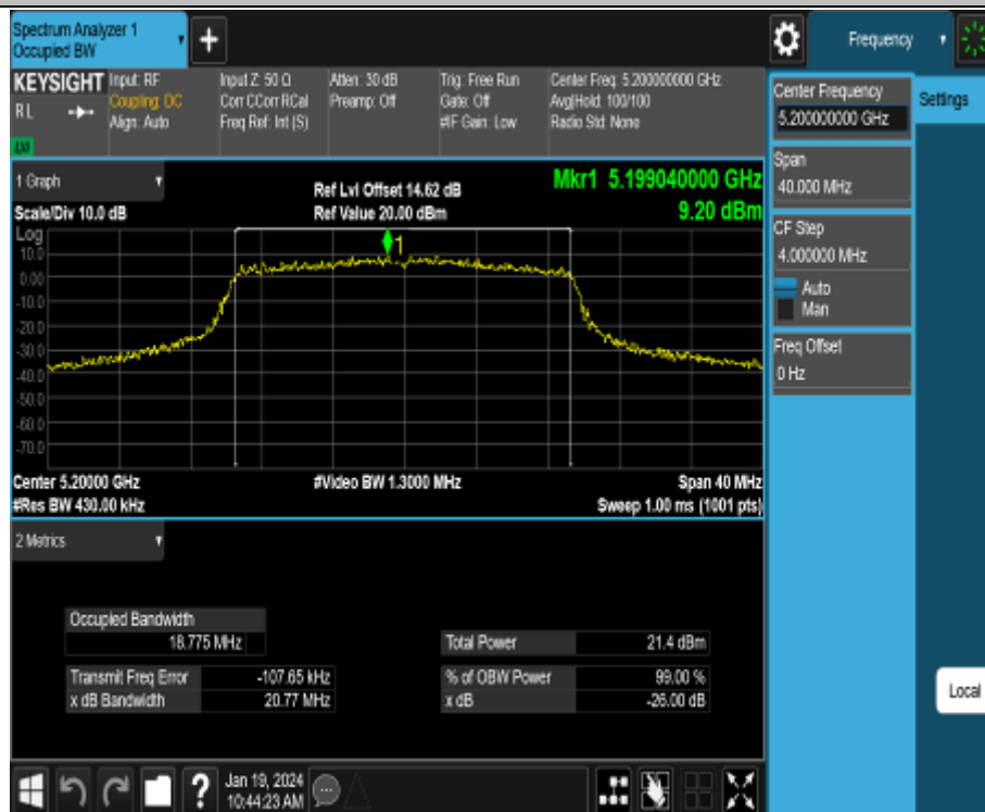
11AX20MIMO_Ant2_5200
