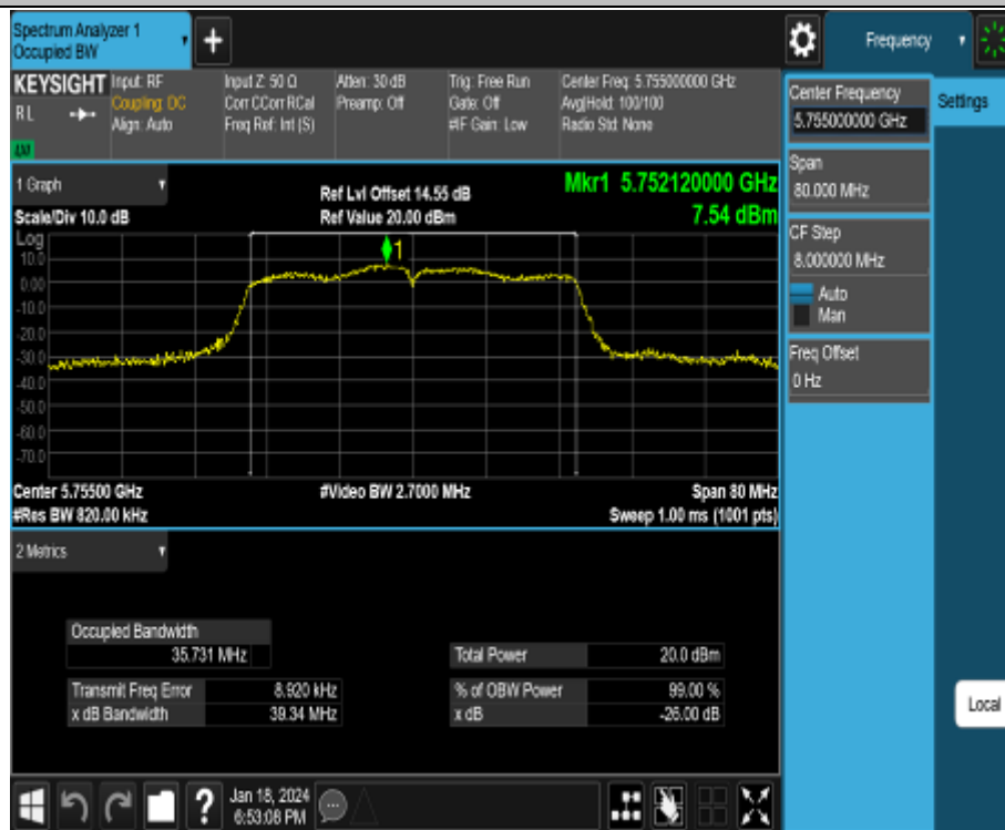
11N40MIMO_Ant2_5755
