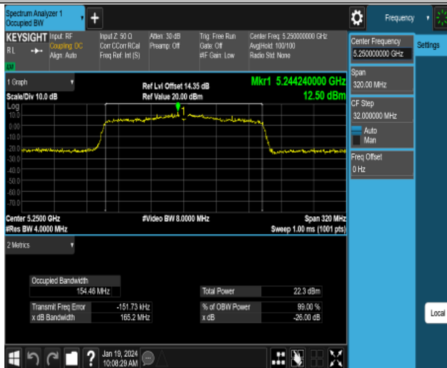
11AC160MIMO_Ant2_5250
