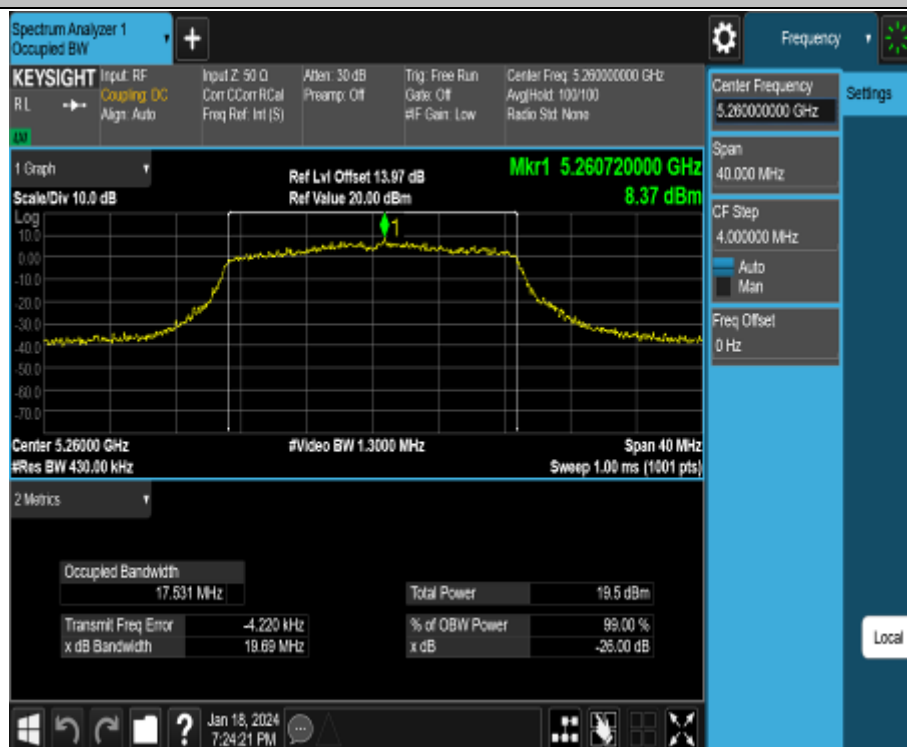
11AC20MIMO_Ant2_5260
