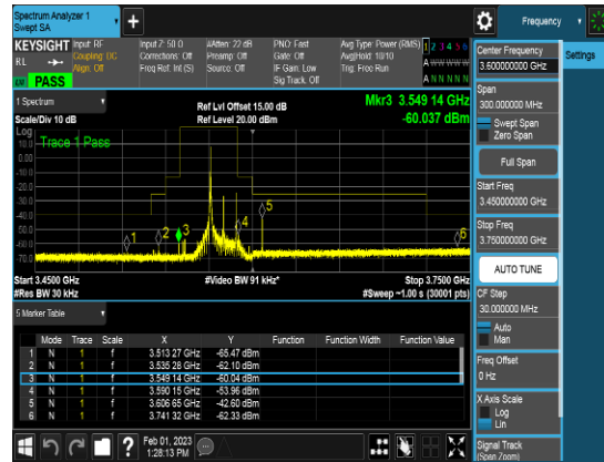
SCC_20M_3579.8MHz_Q64_1RB_CSEpart96
