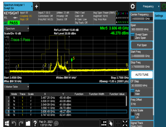
SCC_20M_3579.8MHz_QPSK_1RB_CSEpart96
