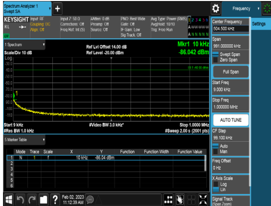
SCC_20M_3579.8MHz_QPSK_1RB_CSE1
