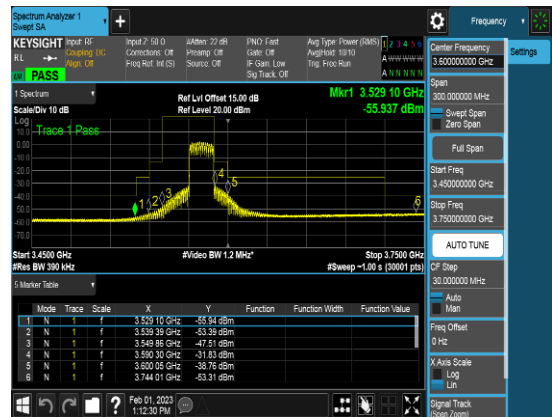
SCC_20M_3579.8MHz_Q16_FULLLRB_CSEpart9 6
