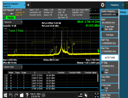
SCC_20M_3634.9MHz_Q16_1RB_CSEpart96
