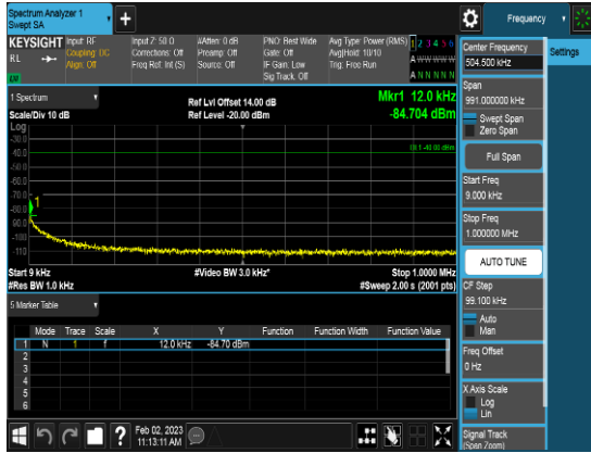
SCC_20M_3579.8MHz_Q16_FULLLRB_CSE1
