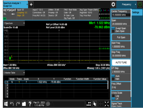
SCC_20M_3579.8MHz_Q16_FULLLRB_CSE2
