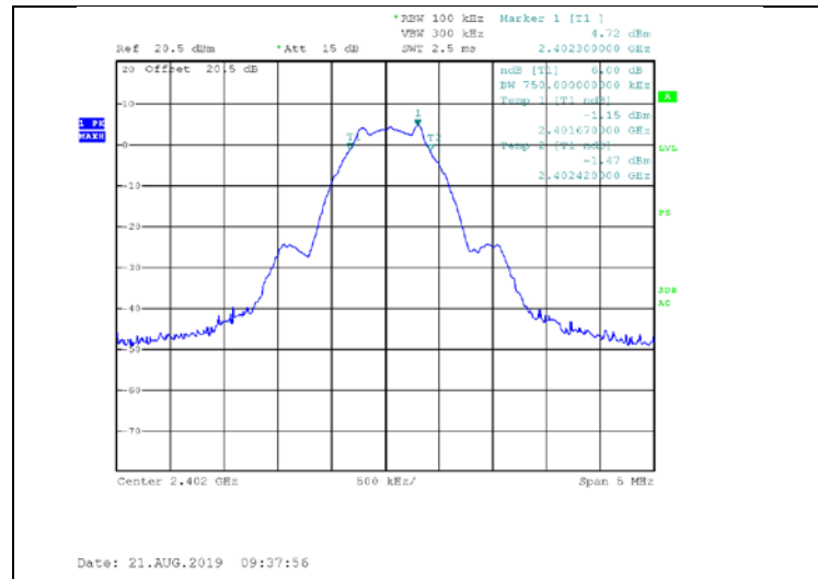
Figure 11. 2402.0 MHz, BLE
