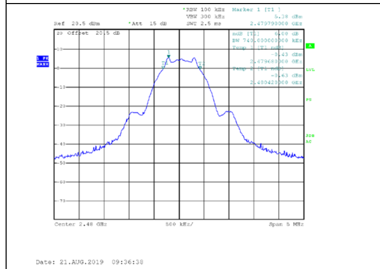
Figure 13. 2480.0 MHz, BLE
