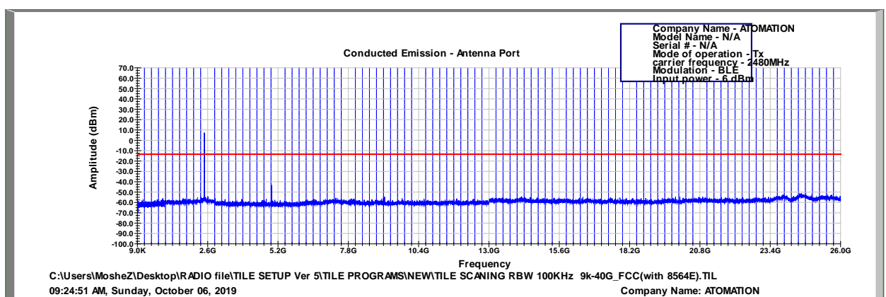
Figure 36 2480.0 MHz, BLE
