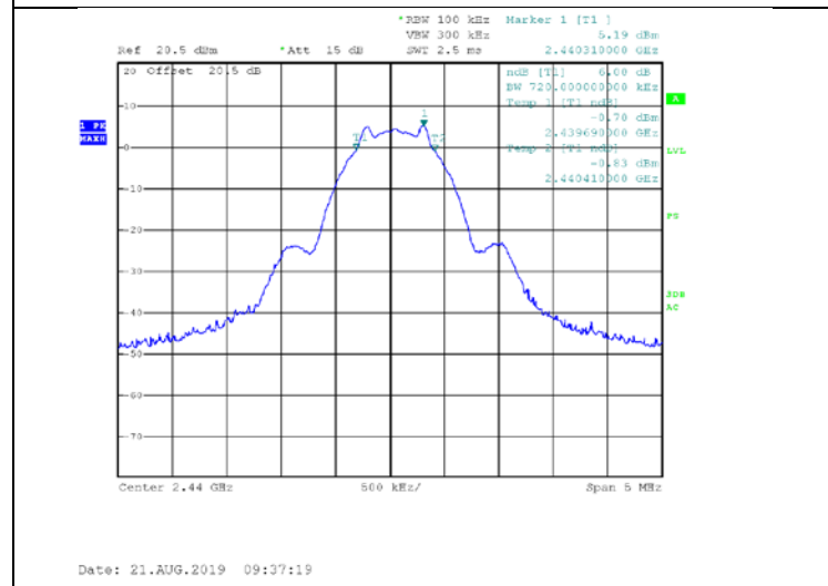
Figure 12. 2440.0 MHz, BLE
