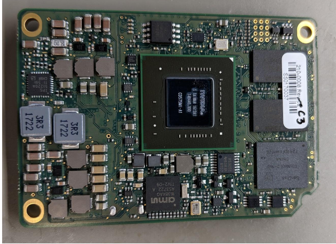
Plus PCBA Side B
