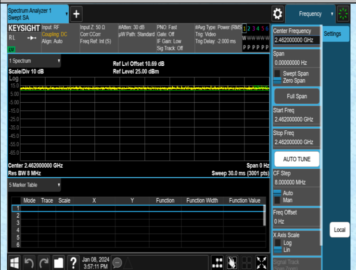
NTNV-11N20MIMO-Ant4-2462
