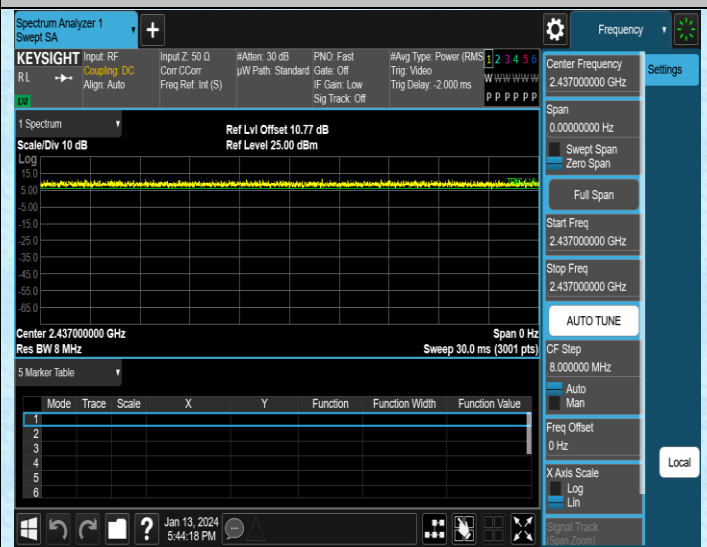
NTNV-11N20MIMO-Ant2-2437
