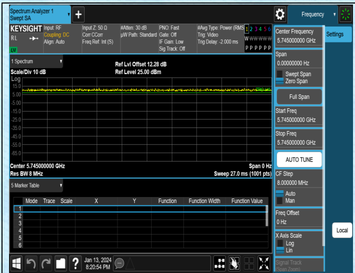
NTNV-11N20MIMO-Ant1-5745
