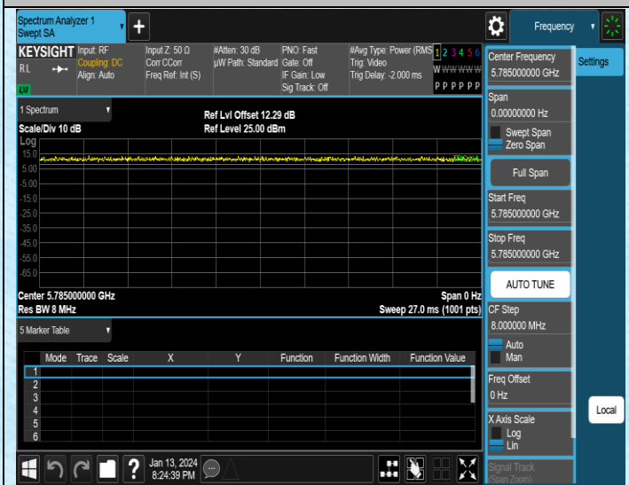
NTNV-11N20MIMO-Ant1-5785
